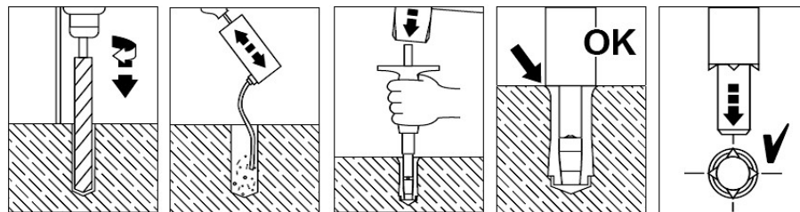
Fig. 4-2: Instrucciones de colocación de los tacos (Proveedor: Hilti)
