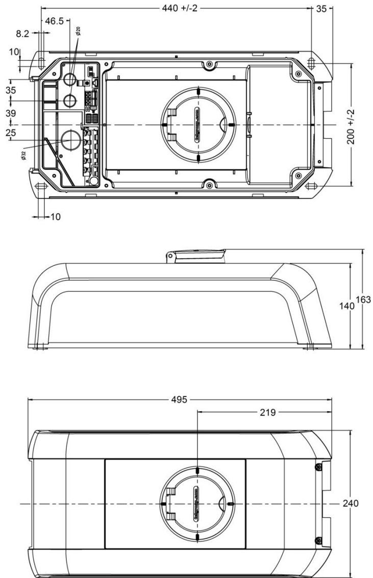
Abb. 12-20: Abmessungen in Millimeter
