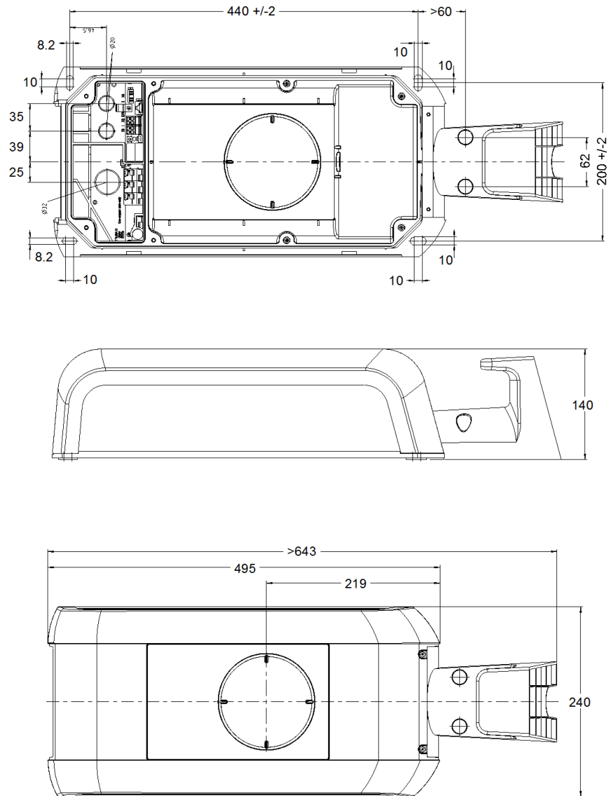
Abb. 12-21: Abmessungen in Millimeter
