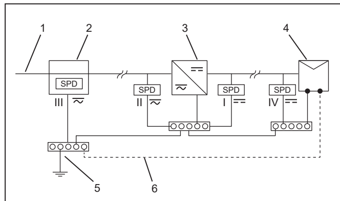
Figura 3.10 Protezione contro le sovratensioni nel sistema fotovoltaico
