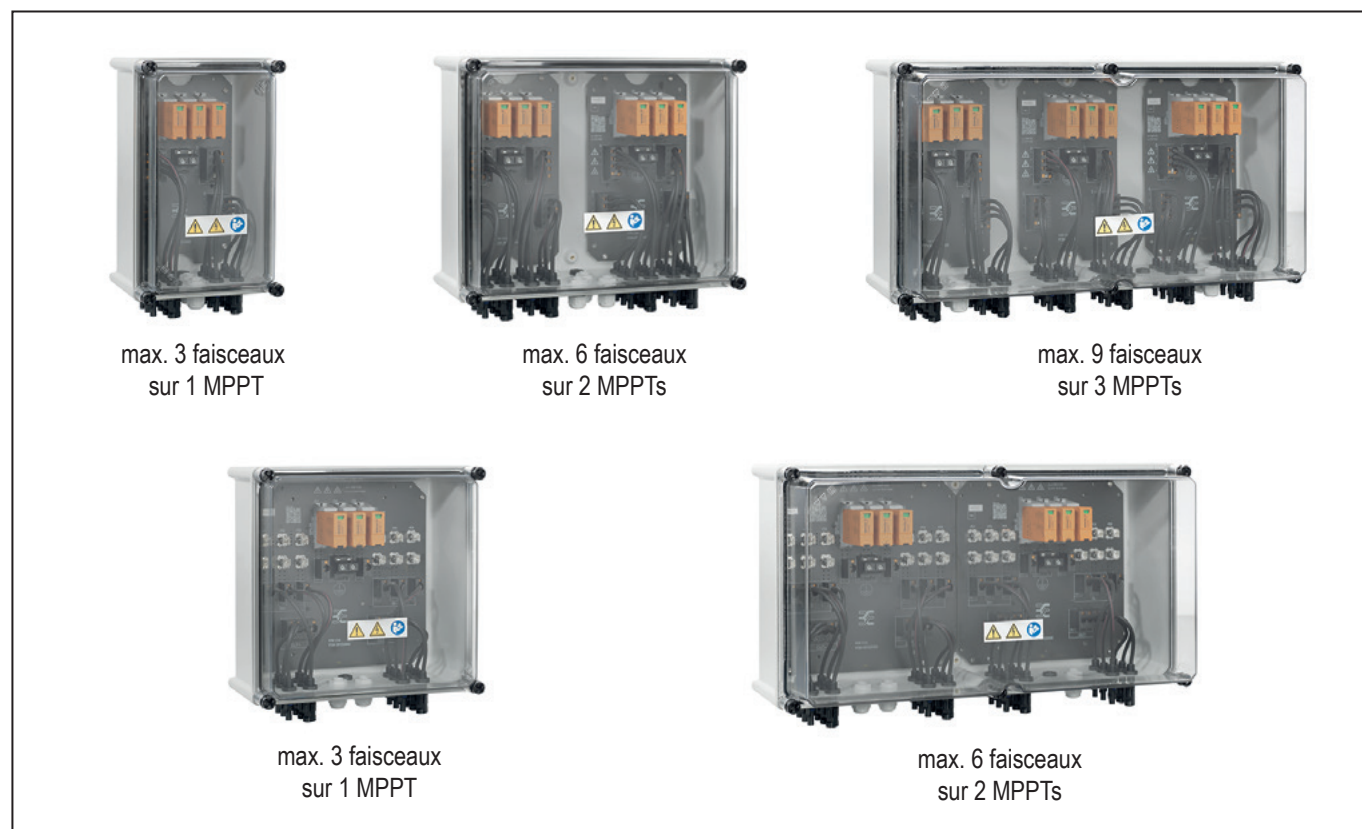
Figure 3.4 Aperçu des différentes versions (seuls les modèles avec connecteurs PV sont affichés sans interrupteurs ni presse-étoupes en option)
