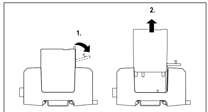
Figure 8.19 Retrait des parafoudres
