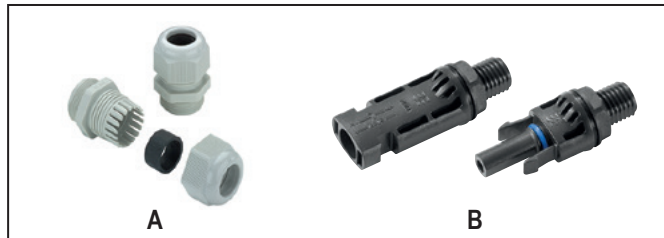
Ilustración 3.6 Prensaestopas (A) y conectores FV (B)
