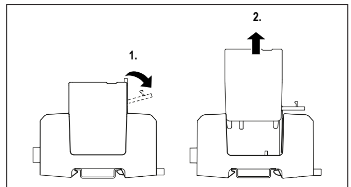
Figura 8.2 Rimozione degli scaricatori dei dispositivi di protezione contro le sovratensioni
