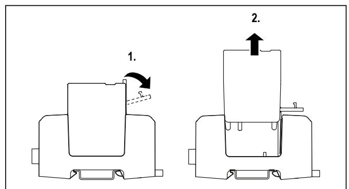
Ilustración 8.2 Retirar los descargadores de protección contra sobretensiones
