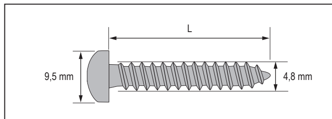
Ilustración 5.3 Dimensiones de los tornillos de sujeción
