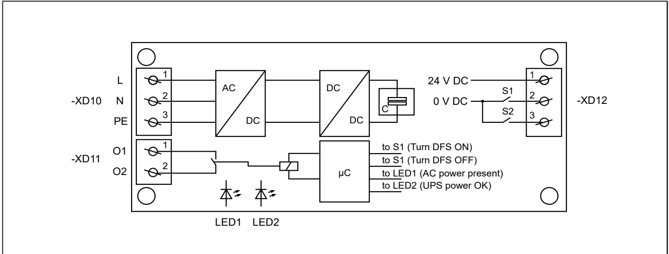
Bild 3.4 Blockschaltbild
