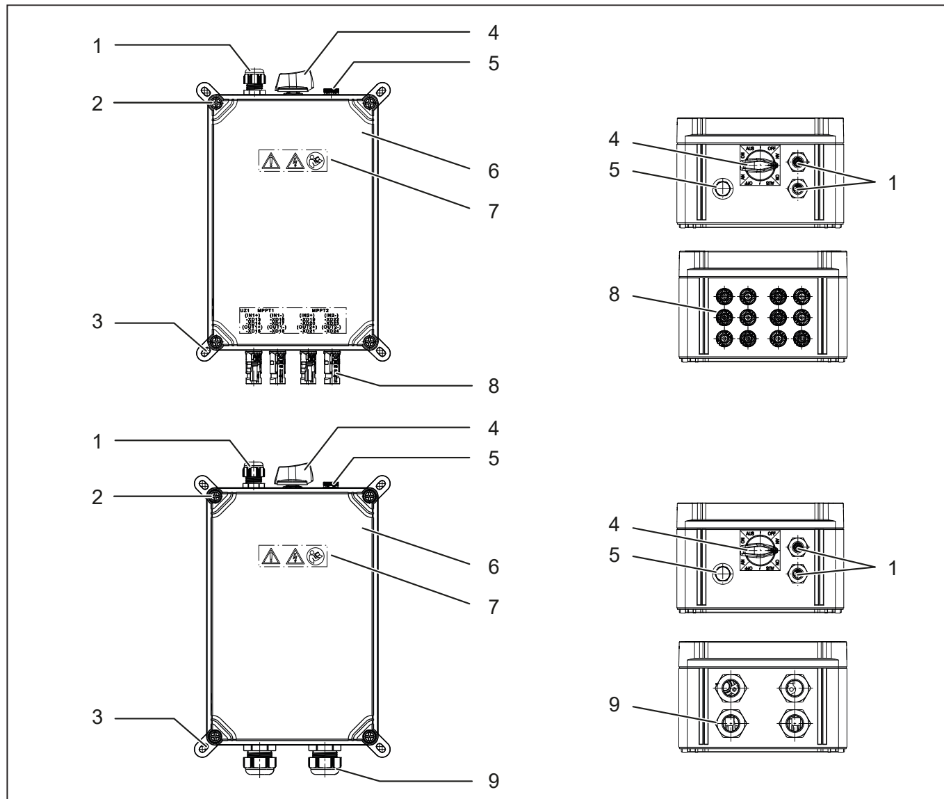
Bild 3.2 Produktübersicht (Beispiel)
