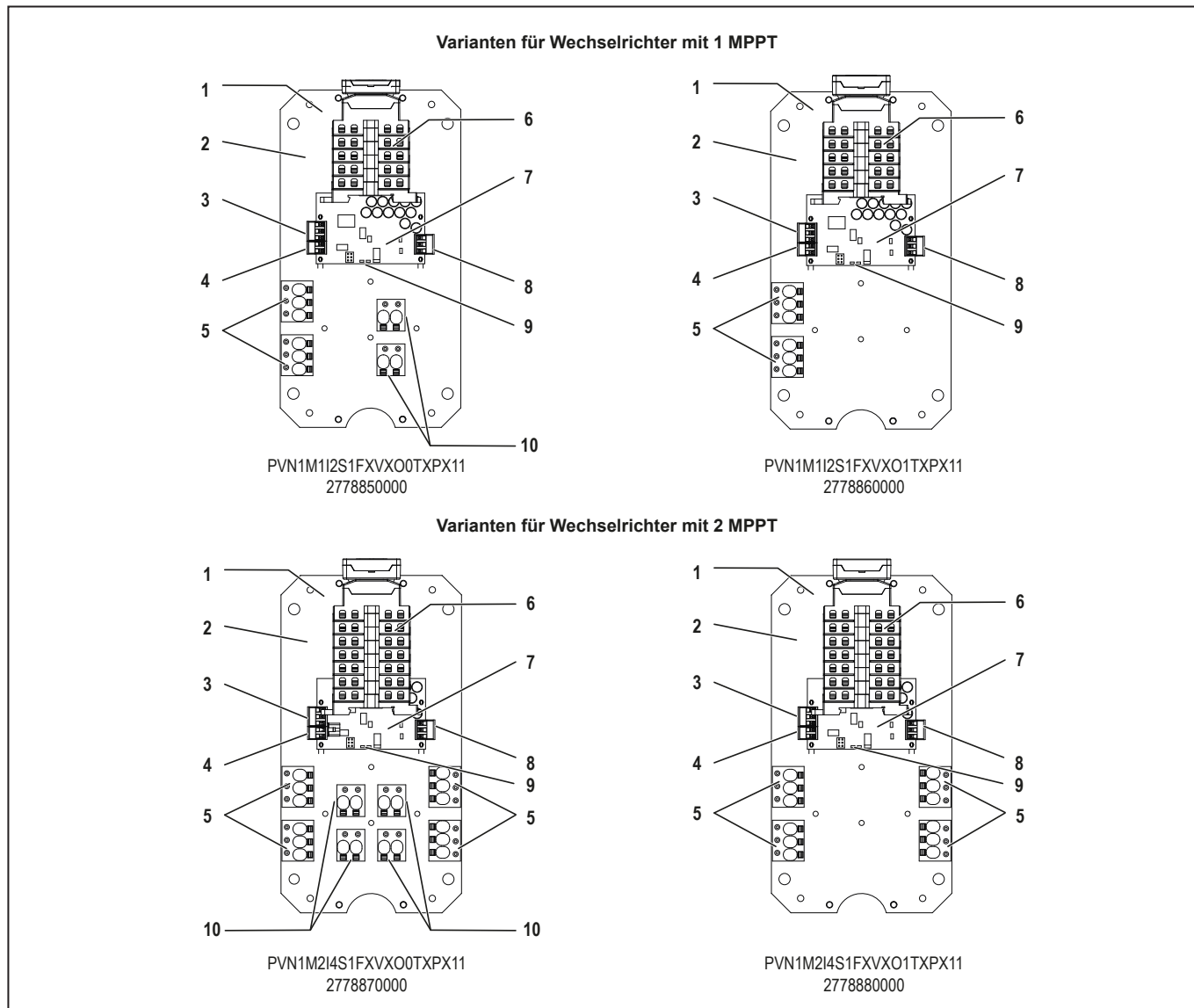
Bild 3.3 Übersicht der Komponenten auf der Leiterplatte
