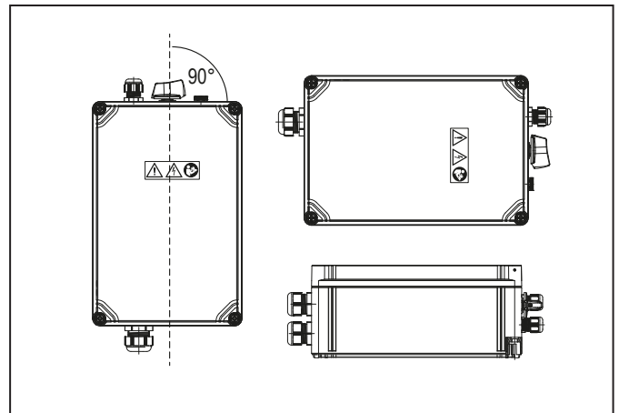
Bild 5.1 Senkrechte und waagerechte Ausrichtung und auf der Rückseite liegend montiert
