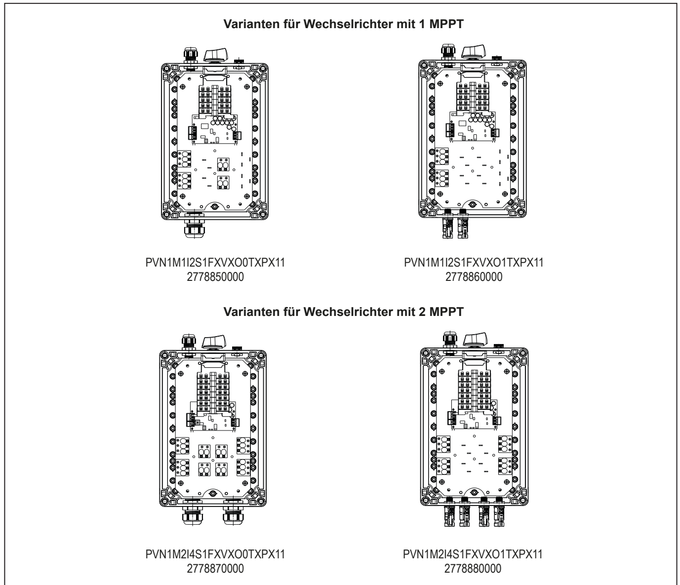
Bild 3.1 Übersicht der Produktvarianten
