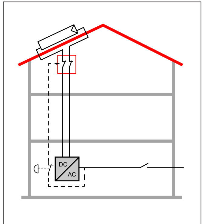
Bild 3.5 Anschlussbeispiel
