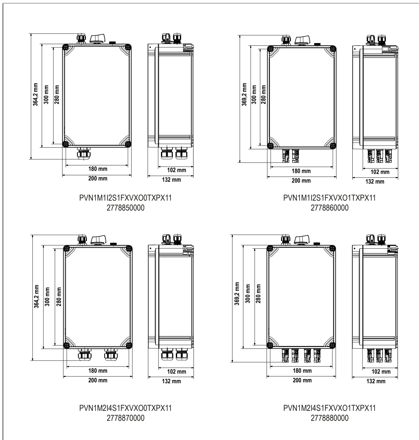
Bild 5.5 Maße für Direktmontage ohne Befestigungslaschen
