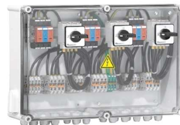
(Beispielbild, kann vom eigentlichen Produkt abweichen) (Example of Combiner Box. Picture may differ from product)
