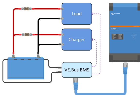
Il VE.Bus BMS V2 scollega i carichi e i caricabatterie tramite la “disconnessione del carico” e la “disconnessione della carica” e controlla l'inverter/caricabatterie
