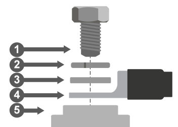
Collegamento del cavo della batteria
