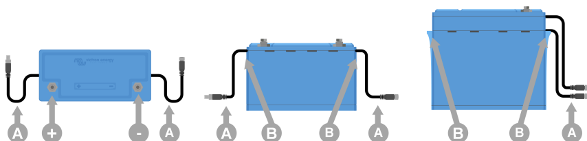
Vista superiore e viste laterali, nelle quali appaiono i morsetti della batteria (+ e -), i cavi BMS (A) e le maniglie di trasporto (B)
