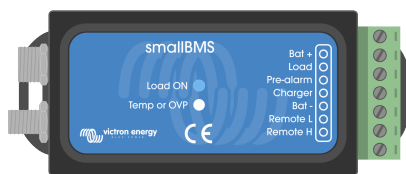
Lo smallBMS
