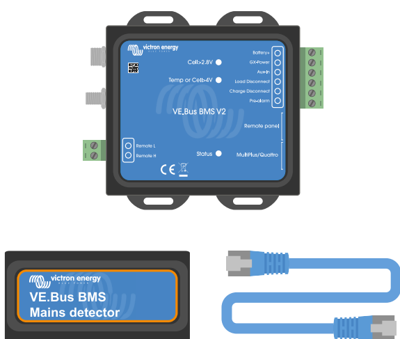
VE.Bus BMS V2, rilevatore di rete del VE.Bus BMS e cavo RJ45 UTP
