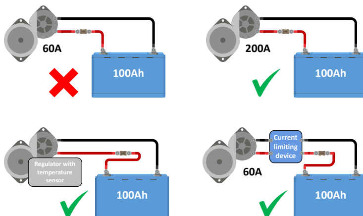
Carica dall'alternatore
