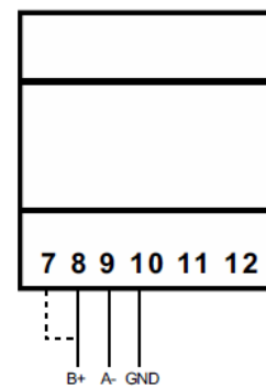
Fig. 13 Dernier appareil sur RS485
