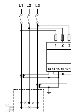
Fig. 7 Triphasé sans neutre (3 fils). MID
