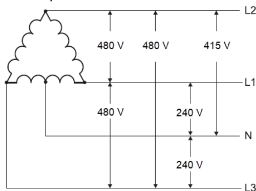
Fig. 4 Système biphasé avec neutre (3 fils)
