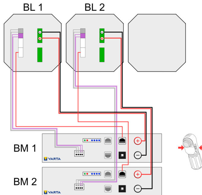
Abbildung 7: Batterielader 1 und 2, Batteriemodul 1 und 2
