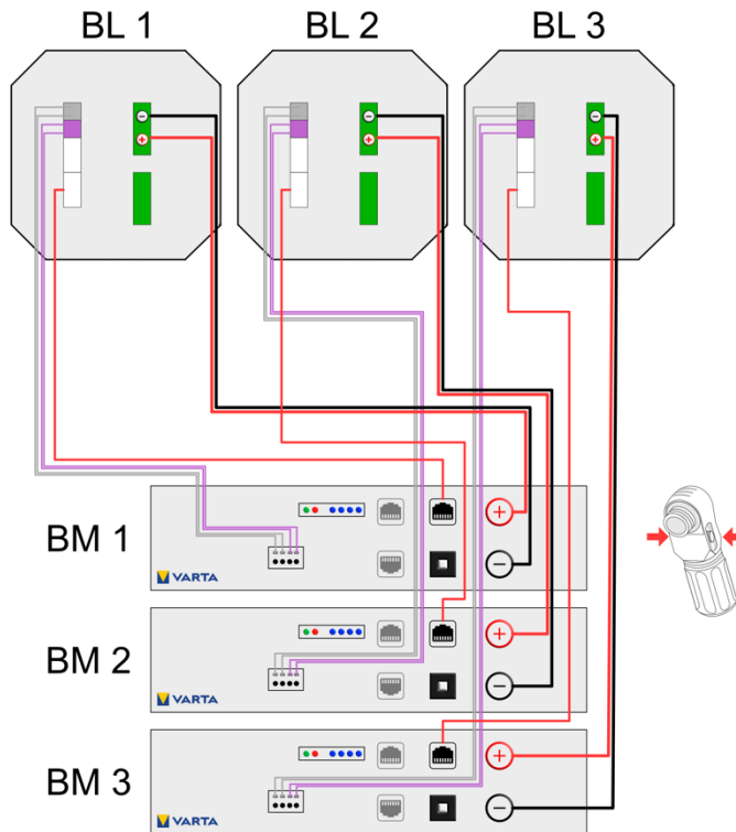
Abbildung 5: Batterielader 1 und 2, Batteriemodul 1, 2 und 3, Batteriemodul 1, 2 und 3
