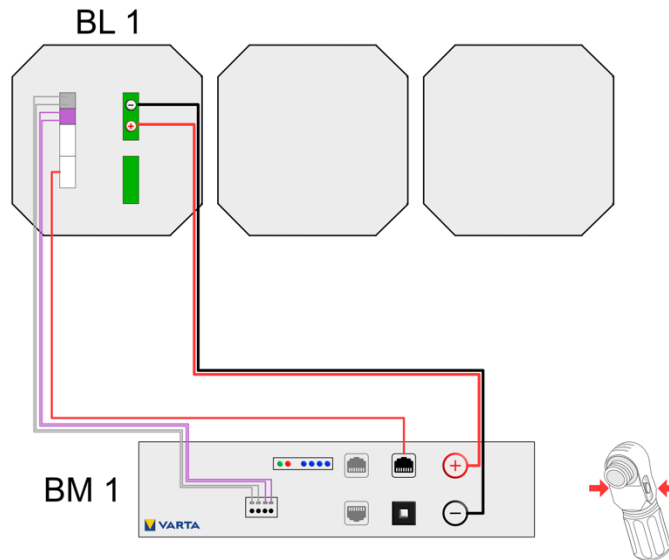
Abbildung 1: Batterielader 1 - Batteriemodul 1
