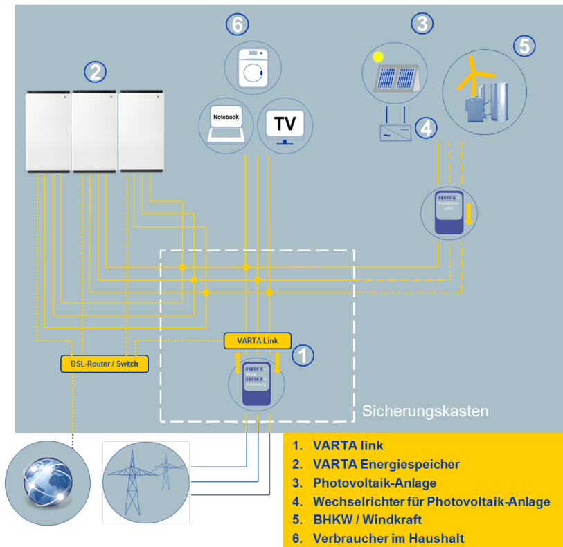
Abbildung 1: Systemübersicht
