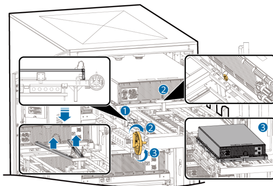
Abbildung 4-14 Einbau der Batterieverbindungsstange
