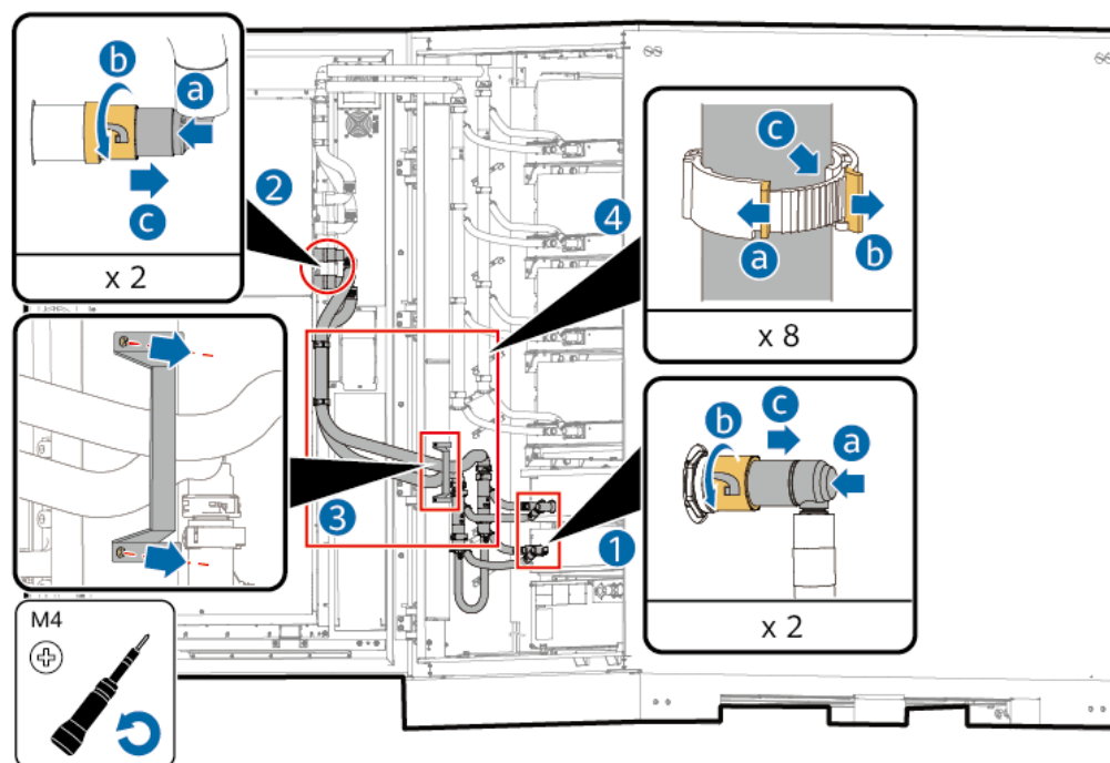
Abbildung 9-4 Trennen des Rohrs
