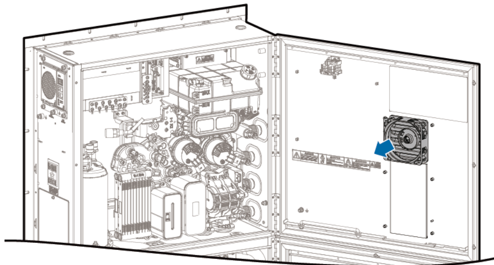
Abbildung 8-10 Entfernen des Entfeuchtungslüfters
