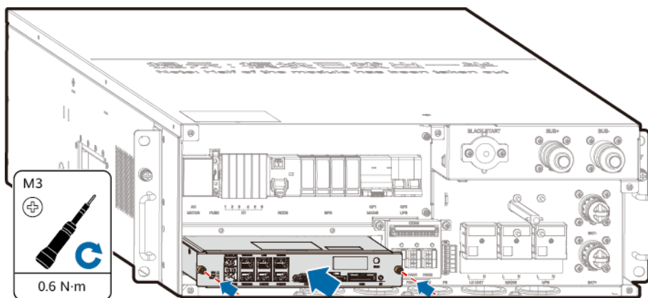
Abbildung 7-20 Installieren des neuen Batteriesteuergeräts
