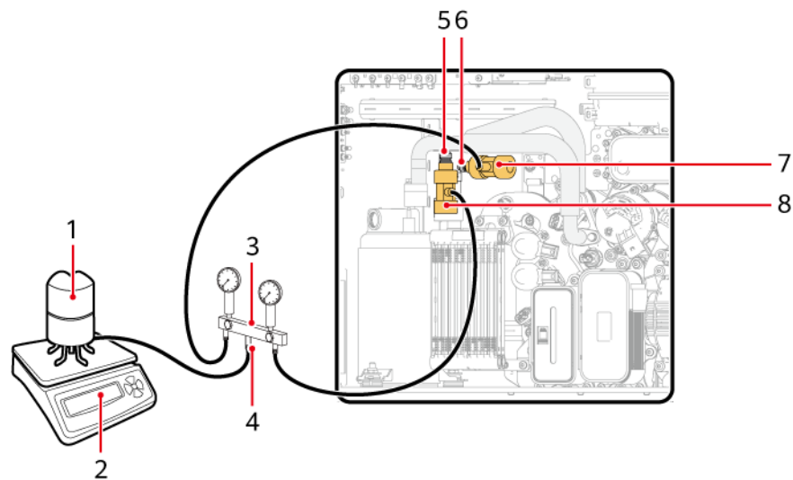
Abbildung 19-21 Vorfüllen des Kältemittels
