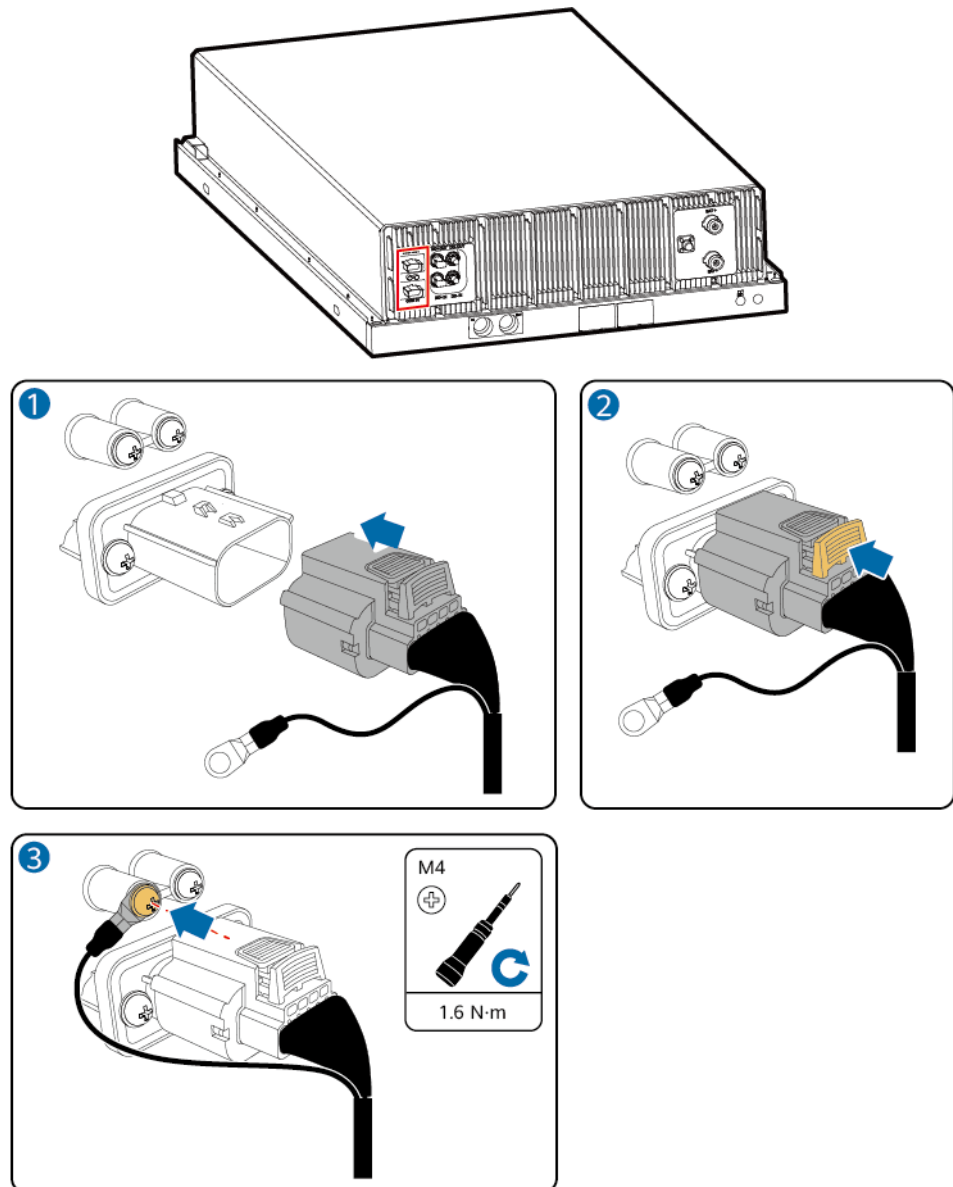
Abbildung 4-23 Anschließen des Kommunikationskabels
