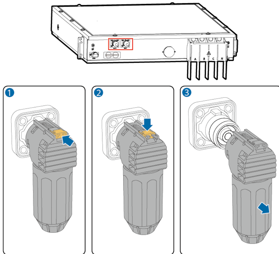
Abbildung 5-4 Methode 2 zum Entfernen der Leistungsklemme
