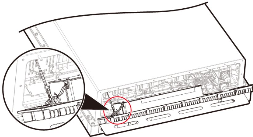
Abbildung 4-43 Installieren des Kabelbaums auf der linken Seite
