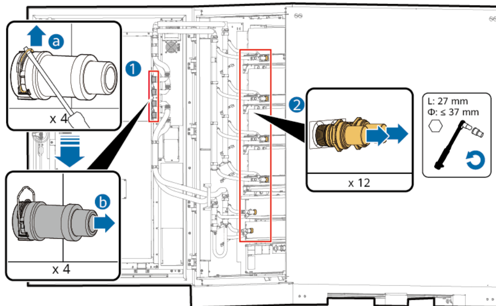
Abbildung 9-5 Entfernen der Stecker der Absperrventile
