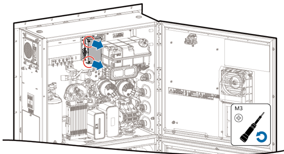
Abbildung 8-20 Entfernen der Abdeckung von der Hauptsteuerungs-Backplane
