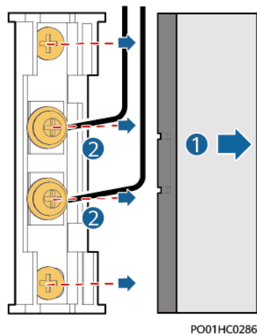
Abbildung 15-2 Entfernen des defekten Türzustandssensors
