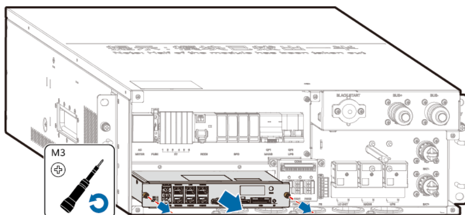
Abbildung 7-19 Entfernen des defekten Batteriesteuergeräts
