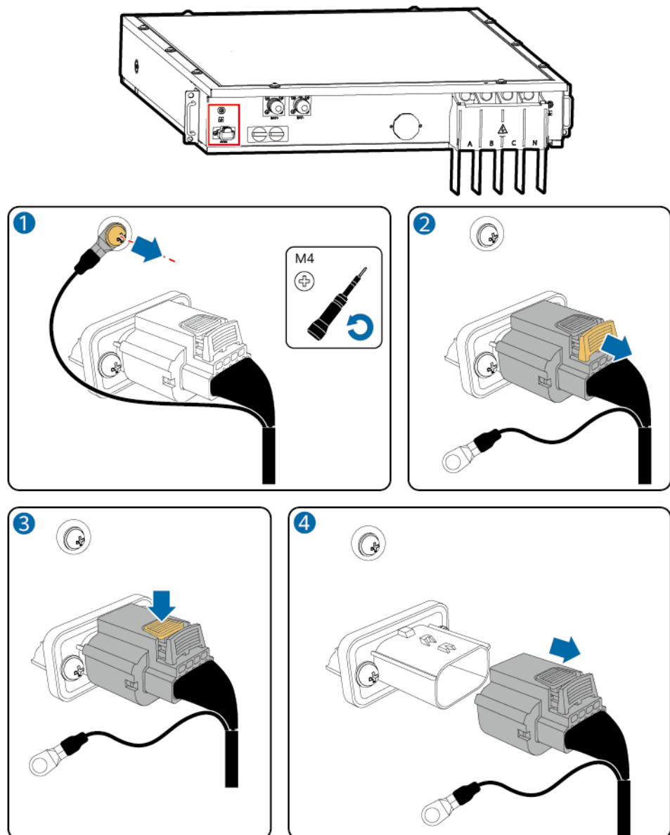
Abbildung 5-6 Entfernen der Kommunikationsklemme
