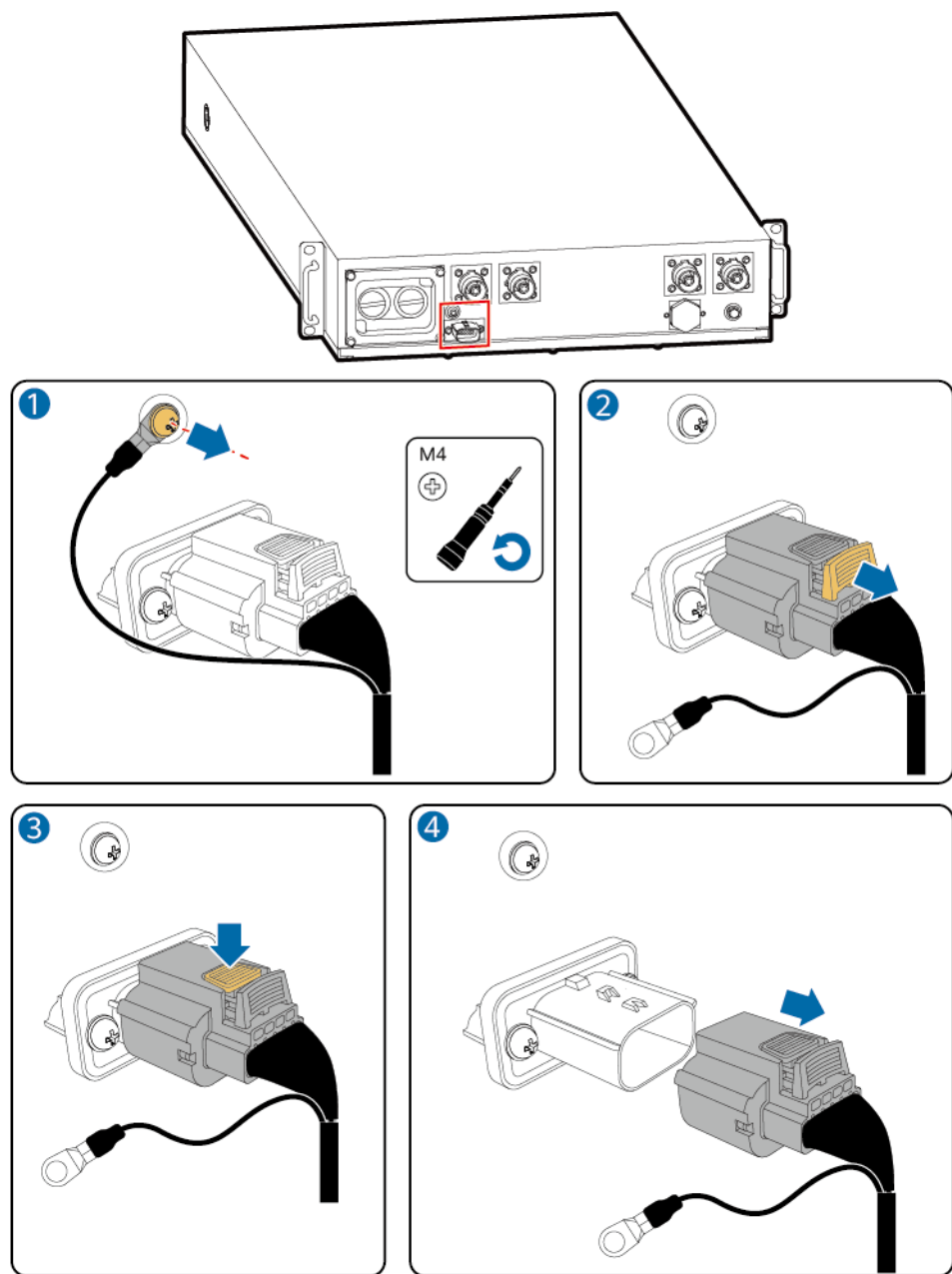
Abbildung 6-4 Entfernen der Kommunikationsklemme
