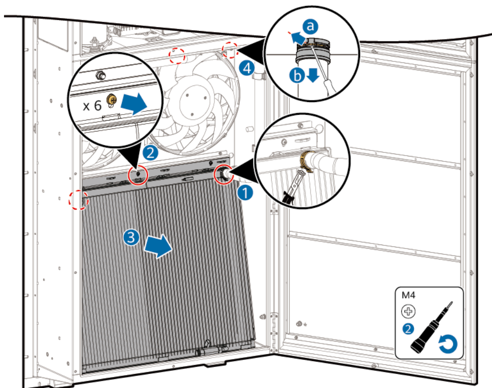
Abbildung 8-27 Entfernen des defekten Außenwärmetauschers und der defekten Rohre
