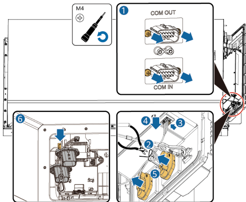
Abbildung 4-54 Entfernen des Kabelbaums auf der linken Seite
