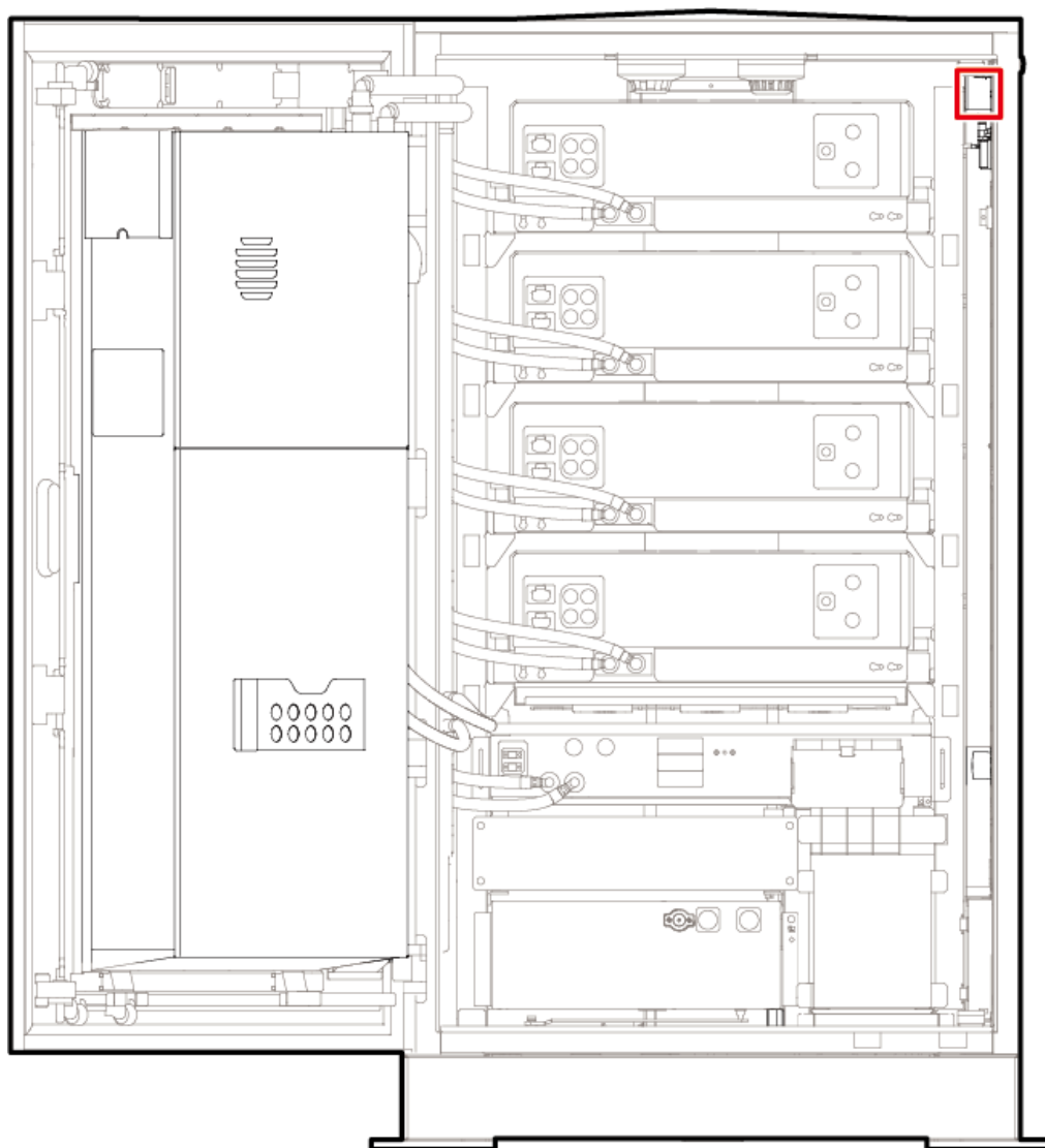
Abbildung 10-5 Position des CO-Sensors
