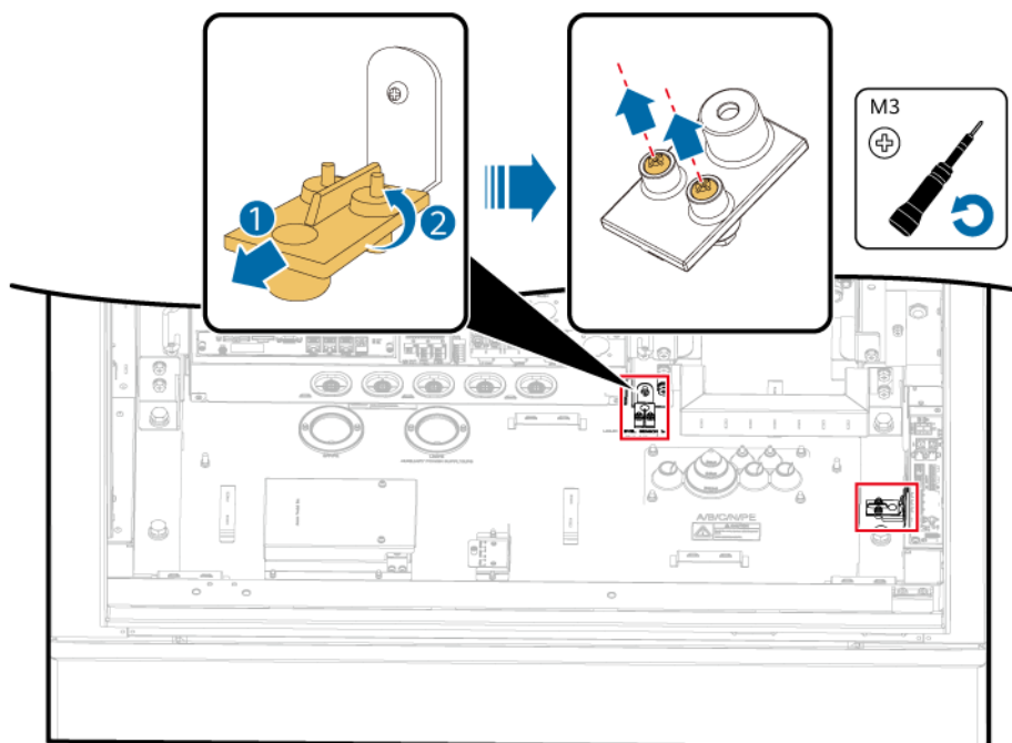
Abbildung 14-3 Entfernen des defekten Wassersensors
