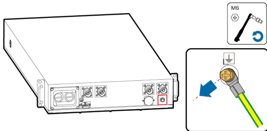
Abbildung 6-6 Entfernen des PE-Kabels
