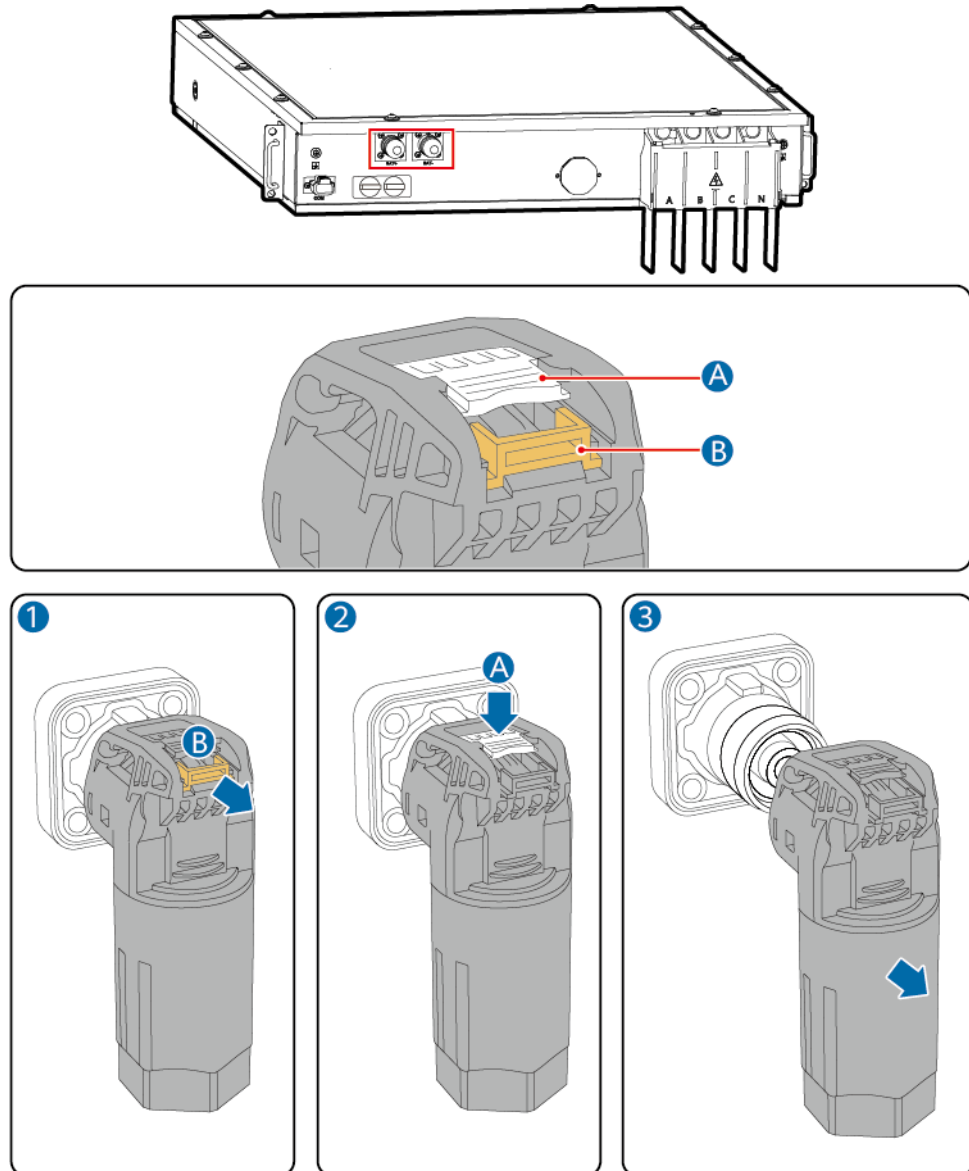
Abbildung 5-3 Methode 1 zum Entfernen der Leistungsklemme
