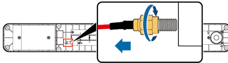
Abbildung 11-4 Trennen des Kabels
