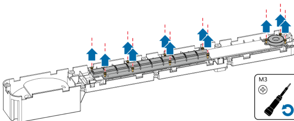
Abbildung 11-3 Entfernen des Lichtleiters und der Lichtleiterhalterung
