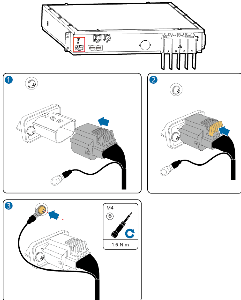
Abbildung 5-13 Anschließen der Kommunikationsklemme
