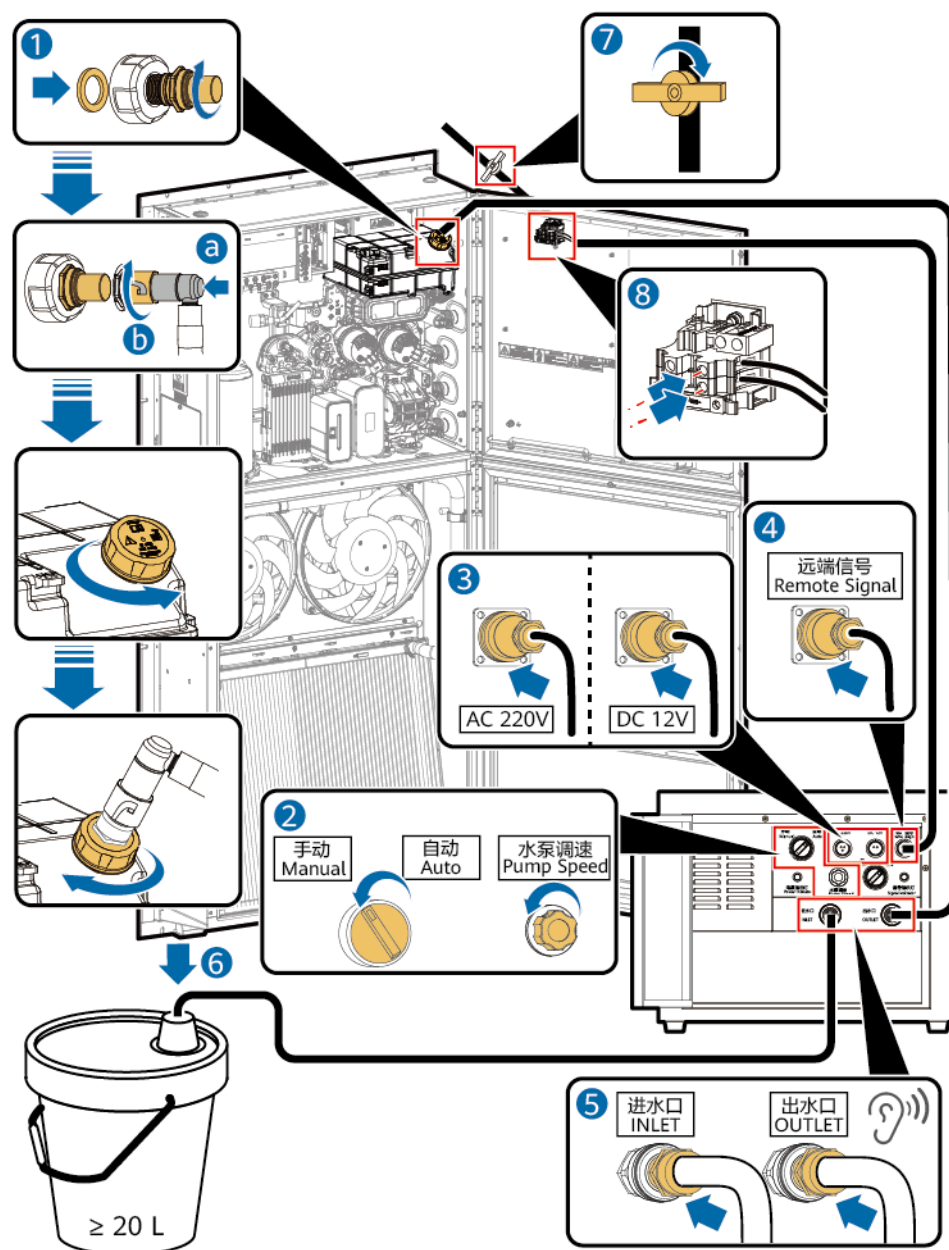
Abbildung 19-15 Installieren der Maschine
