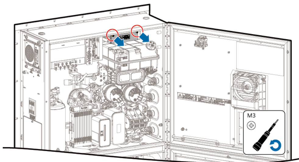
Abbildung 8-28 Entfernen des vorderen Ablenkblechs der Filterplatte
