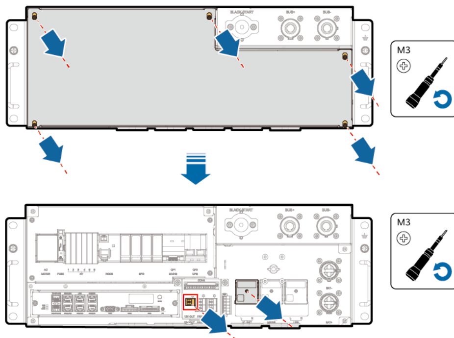
Abbildung 8-4 Entfernen der Kabel
