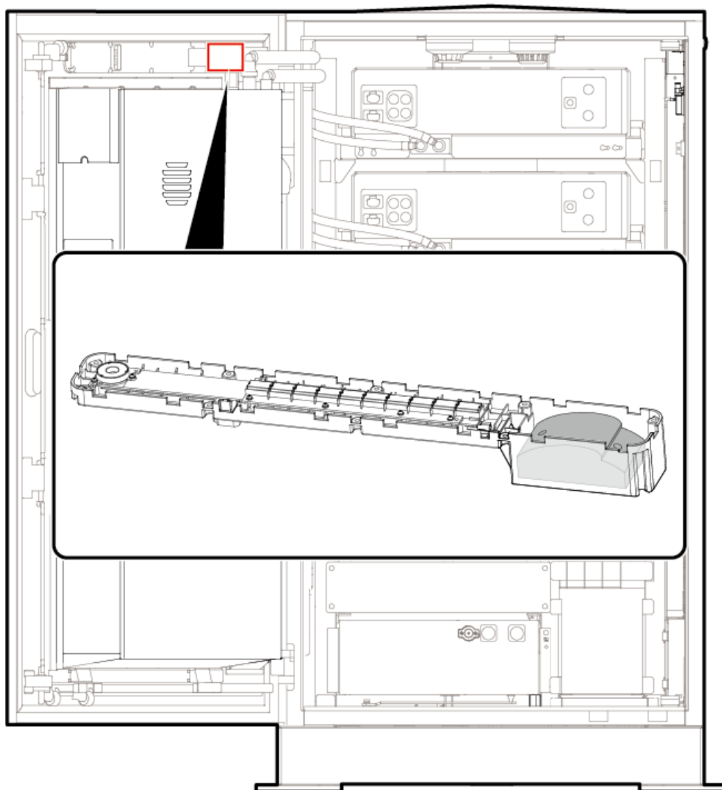
Abbildung 10-7 Position der Feueralarmhupe/-rundumleuchte
