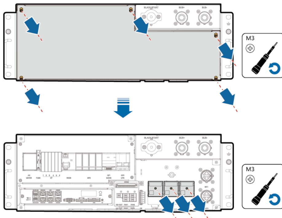
Abbildung 7-23 Entfernen der Wartungsfachabdeckung und der Kabelschutzabdeckung
