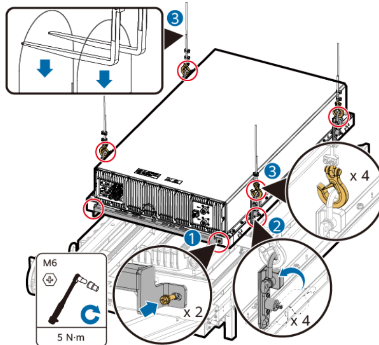
Abbildung 4-16 Befestigen des Akkupacks an der Packvorrichtung (1)
