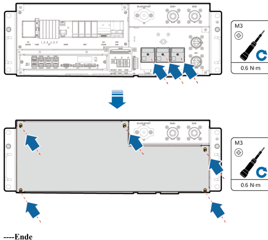
Abbildung 7-28 Einbau der Kabelschutzabdeckung und der Wartungsfachabdeckung
