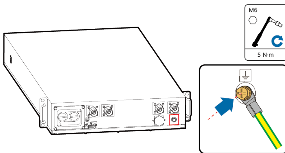
Abbildung 6-11 Anschließen des PE-Kabels
