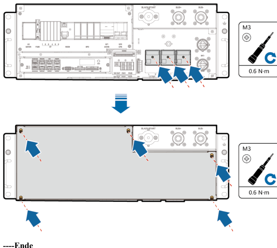
Abbildung 7-6 Einbau der Kabelschutzabdeckung und der Wartungsfachabdeckung
