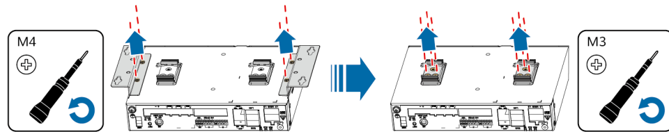
Abbildung 17-4 Entfernen der Umwandlungsklammern vom neuen SmartLogger
