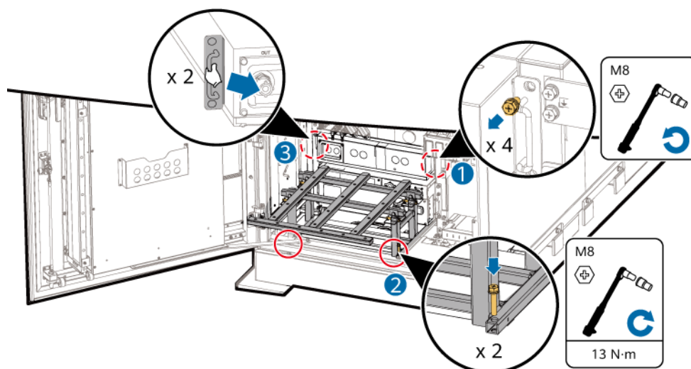
Abbildung 6-7 Verschieben des DCDC in die Vorrichtung
