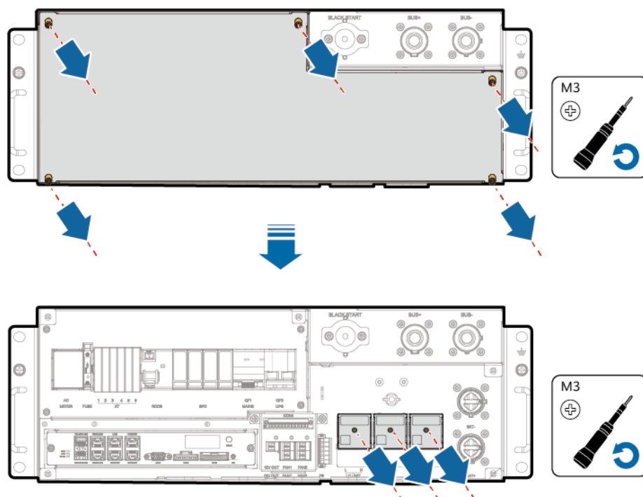
Abbildung 7-2 Entfernen der Wartungsfachabdeckung und der Kabelschutzabdeckung
