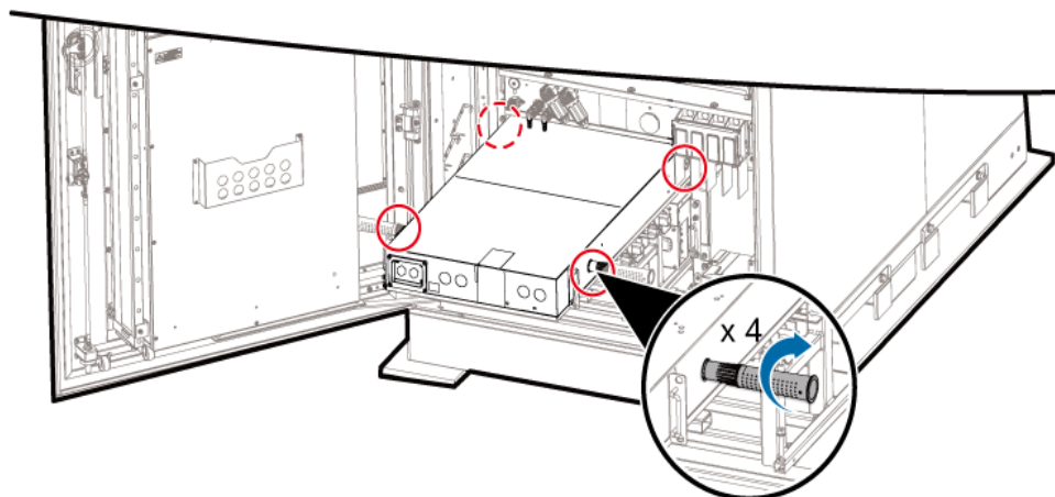
Abbildung 6-8 Installieren der Hebegriffe
