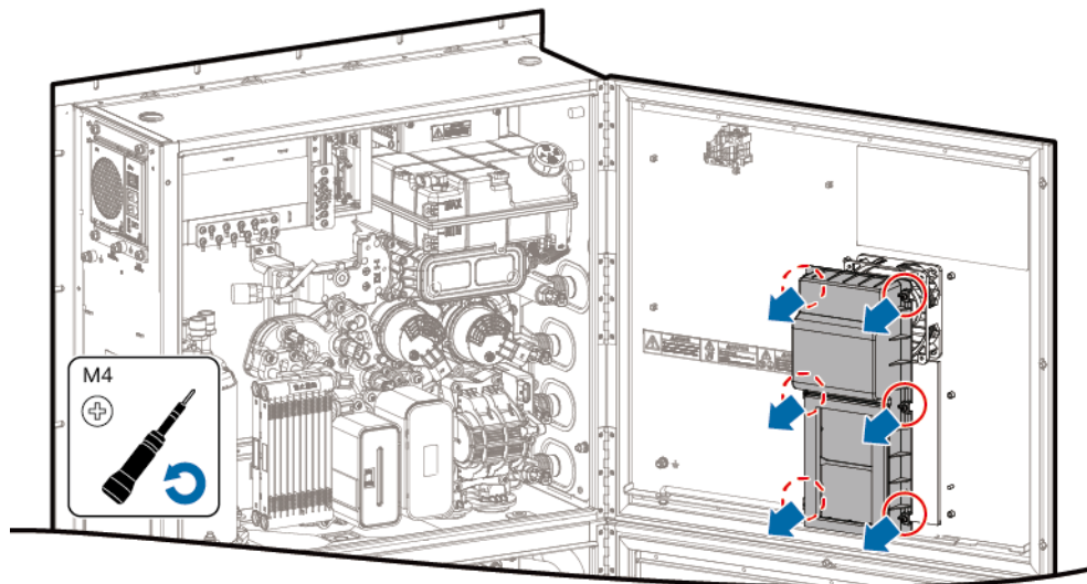
Abbildung 8-9 Entfernen der Schutzabdeckung des Entfeuchtungslüfters
