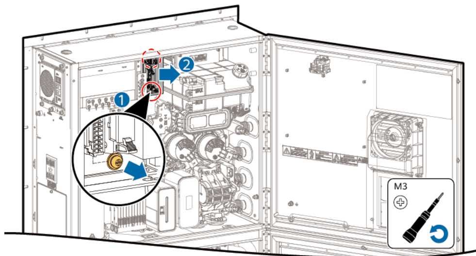
Abbildung 8-21 Entfernen der defekten Hauptsteuerungs-Backplane
