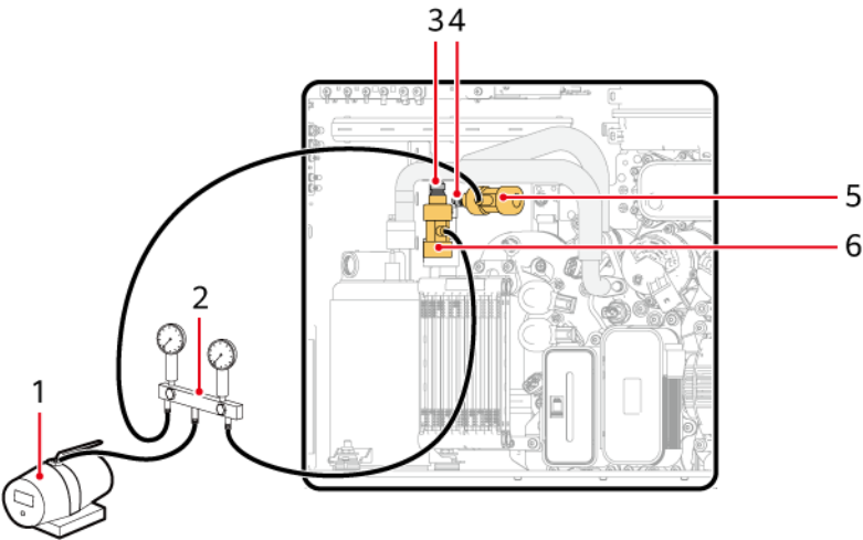
Abbildung 19-20 Vakuumieren
