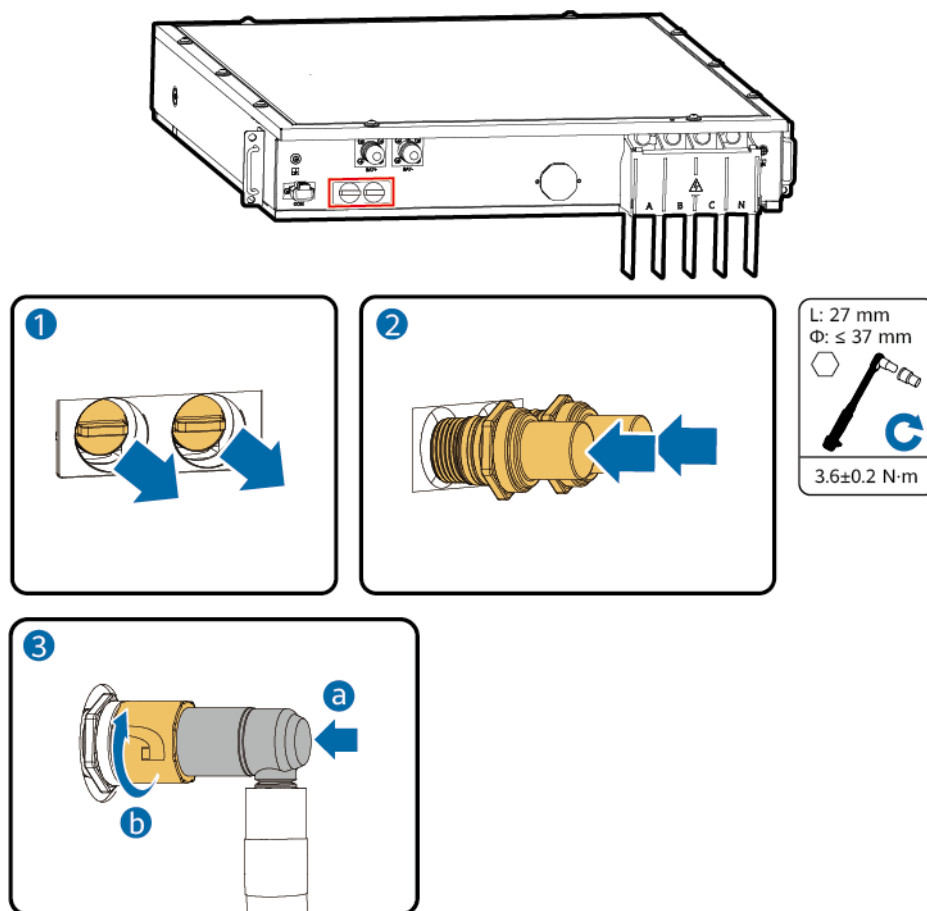
Abbildung 5-15 Anschließen des Absperrventils
