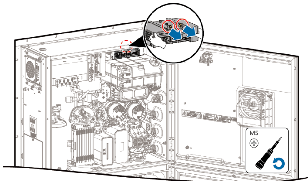
Abbildung 8-29 Entfernen der Befestigungen der Filterplatte
