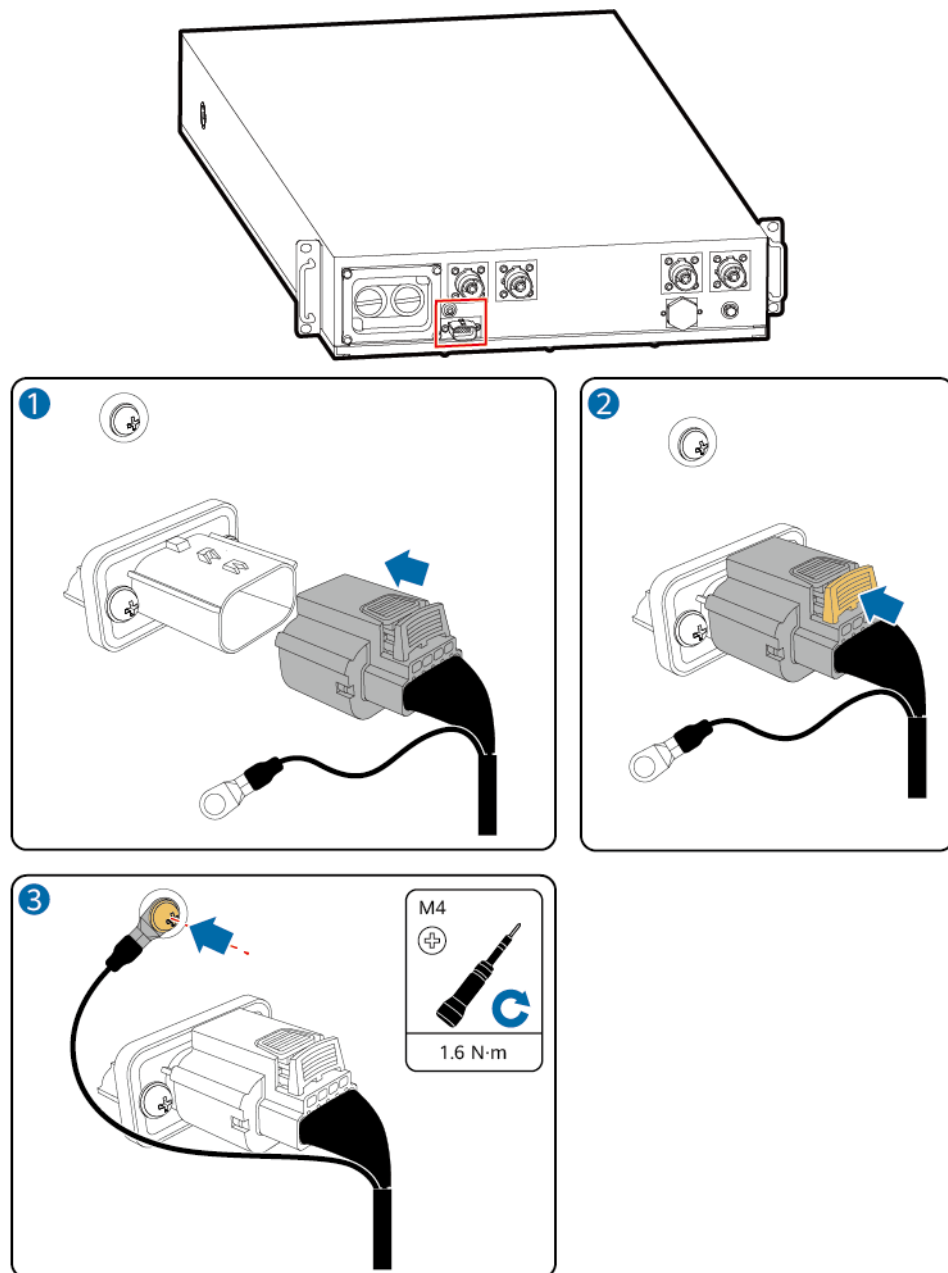
Abbildung 6-14 Anschließen der Kommunikationsklemme
