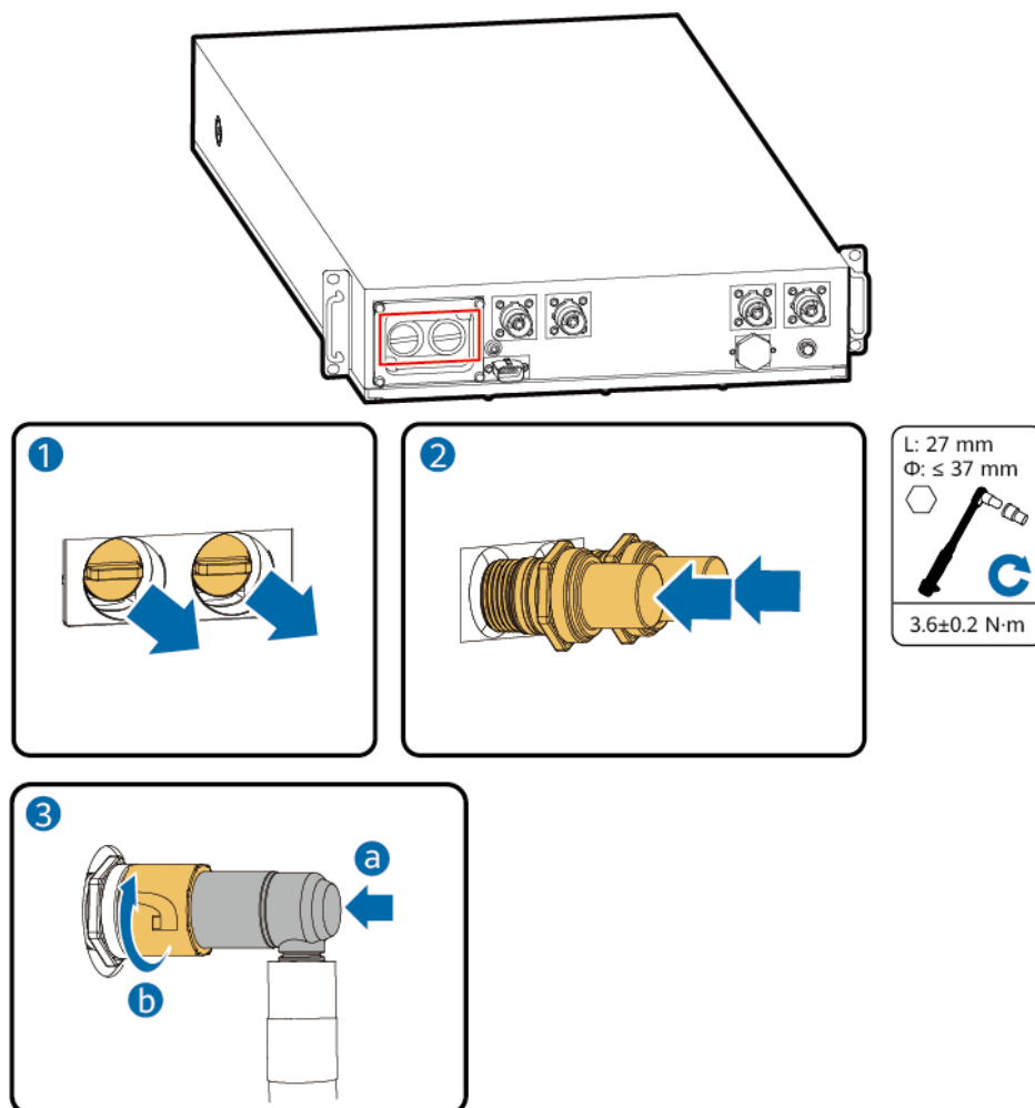
Abbildung 6-13 Anschließen des Absperrventils
