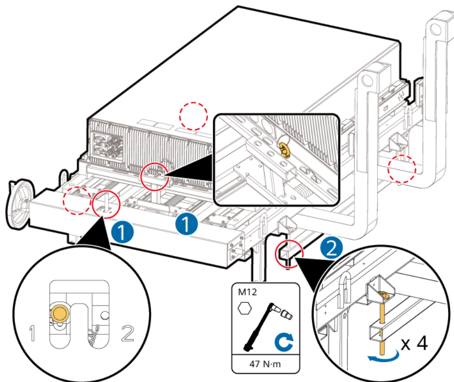
Abbildung 4-17 Befestigen des Akkupacks an der Packvorrichtung (2)
