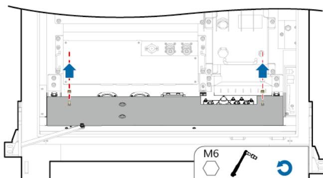
Abbildung 14-2 Entfernen des Ablenkblechs der Kabel
