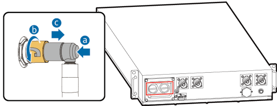
Abbildung 6-5 Trennen der Buchse des Absperrventils vom Stecker
