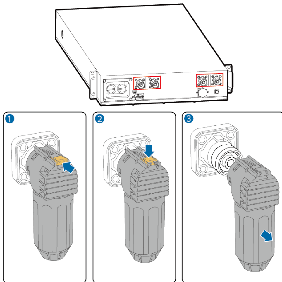
Abbildung 6-3 Methode 2 zum Entfernen der Leistungsklemme
