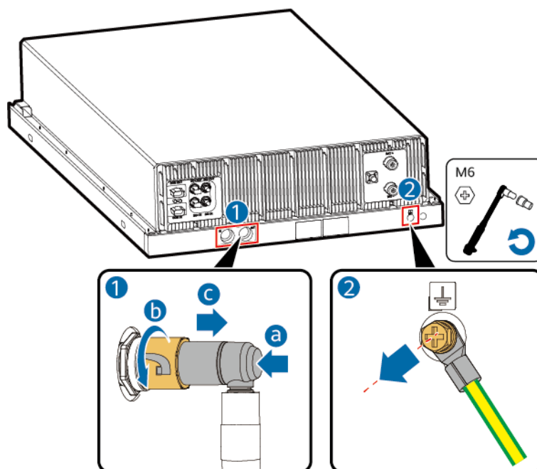
Abbildung 4-8 Entfernen des Absperrventils und des PE-Kabels
