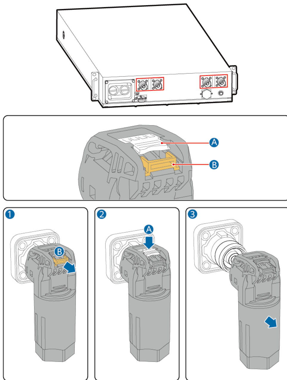
Abbildung 6-2 Methode 1 zum Entfernen der Leistungsklemme
