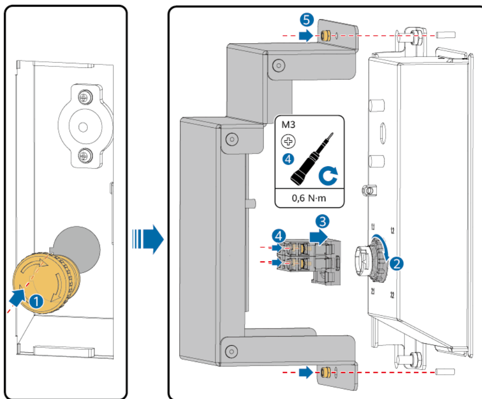
Abbildung 13-3 Installieren des Notausschalters
