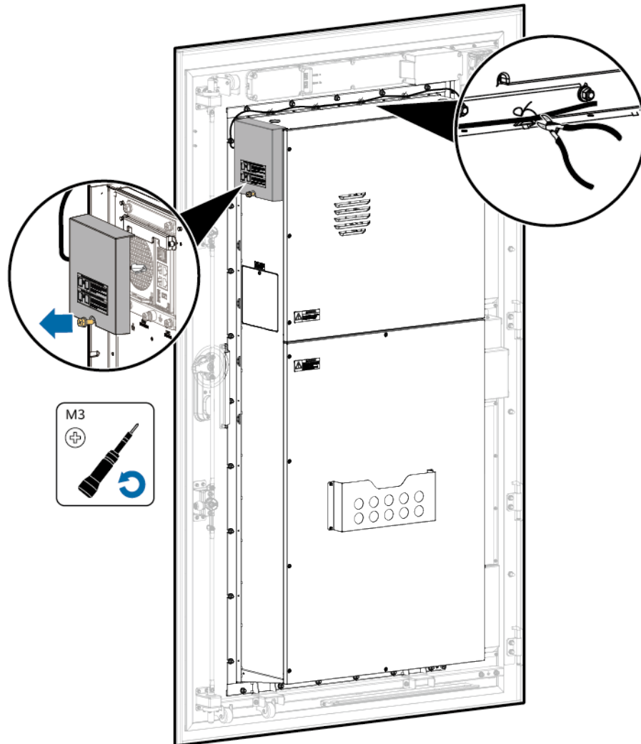
Abbildung 8-3 Entfernen des Kommunikationskabels
