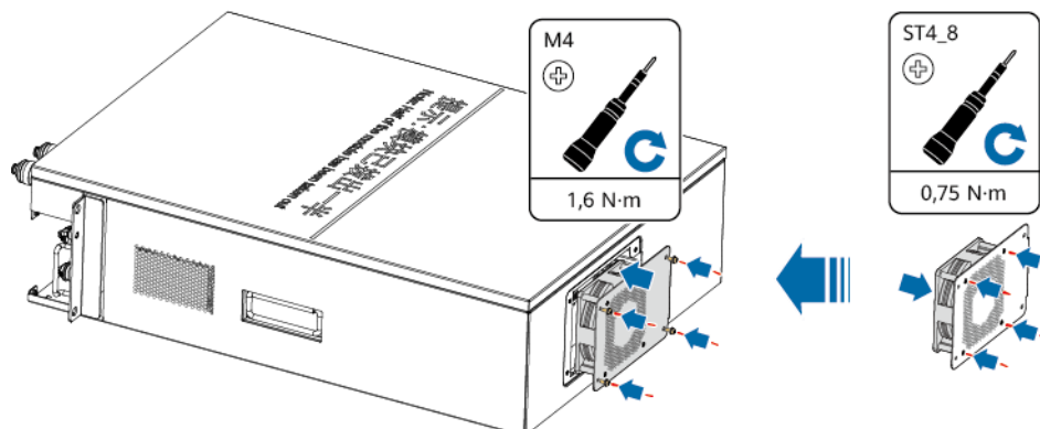
Abbildung 7-26 Installieren des neuen RCM-Lüfters
