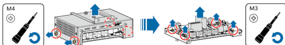
Abbildung 8-30 Entfernen der defekten Filterplatte
