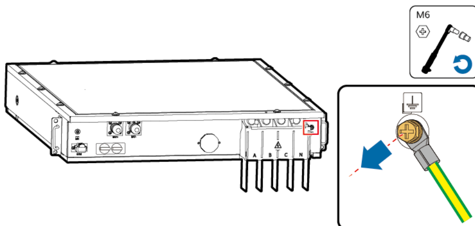
Abbildung 5-7 Entfernen des PE-Kabels
