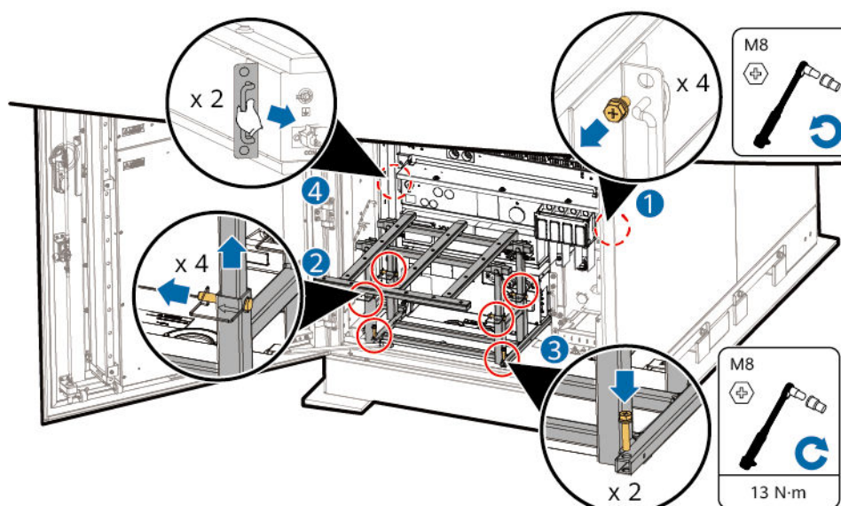
Abbildung 5-8 Verschieben des PCS in die Vorrichtung
