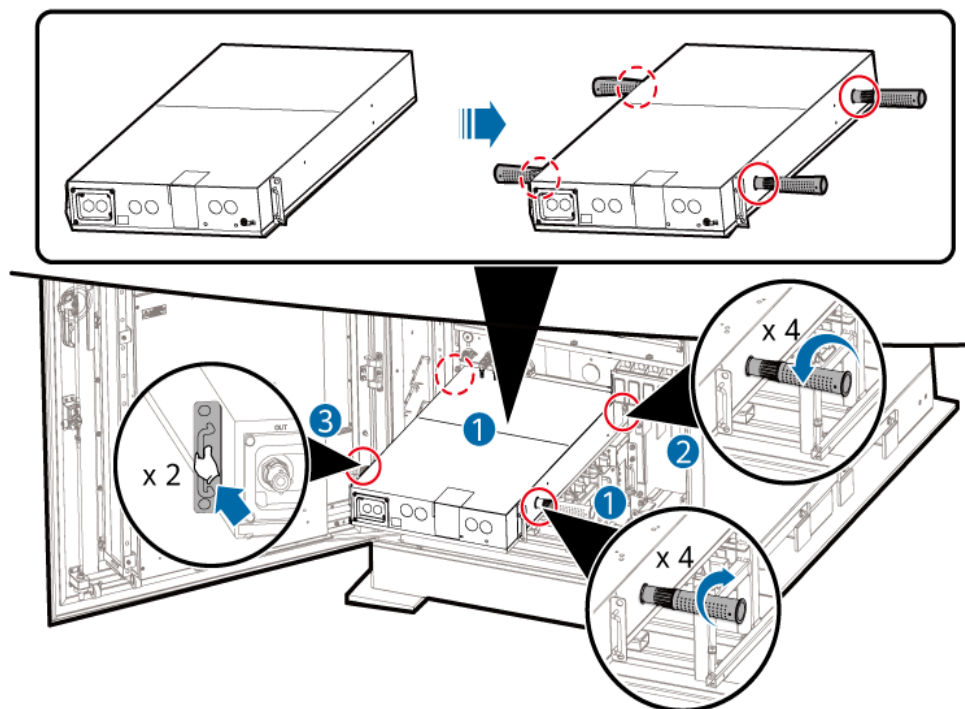
Abbildung 6-9 Schieben des DCDC
