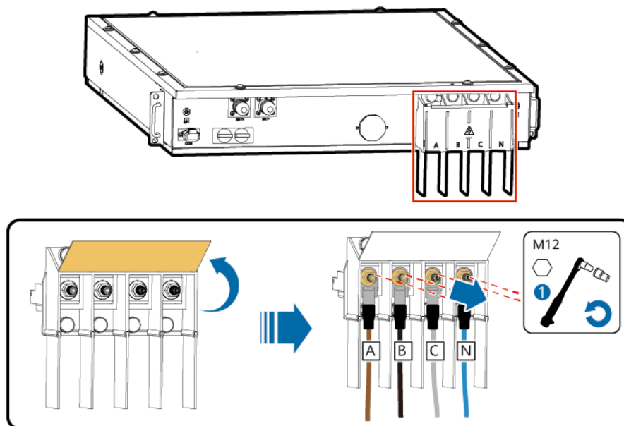
Abbildung 5-2 Entfernen des AC-Stromkabels
