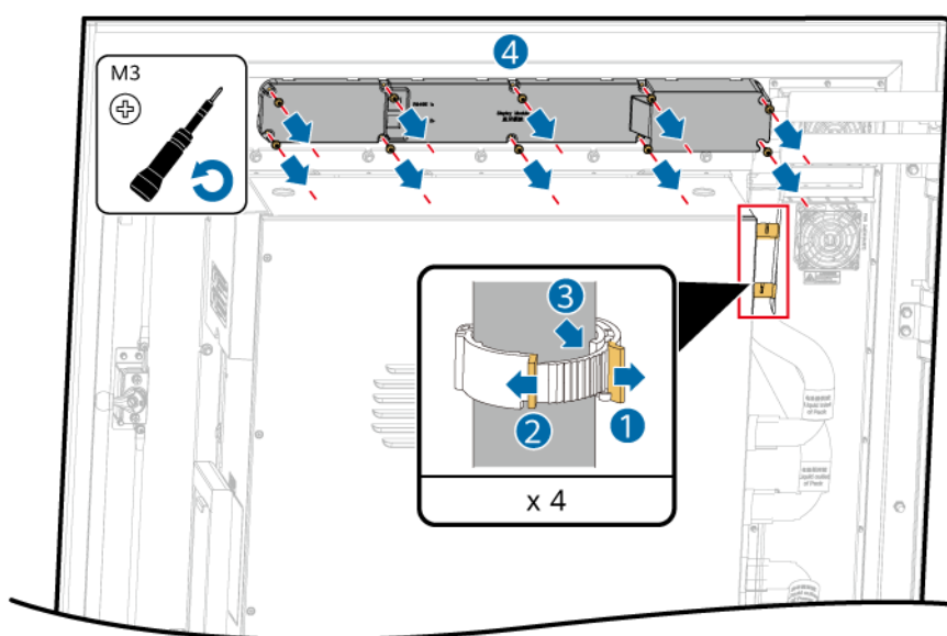
Abbildung 10-8 Entfernen der hinteren Abdeckung des Anzeigemoduls
