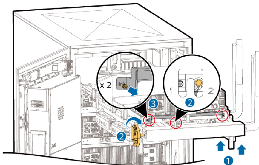
Abbildung 4-15 Entnehmen des Akkupacks
