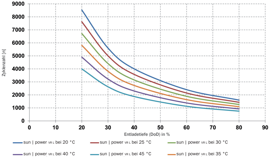
Abb. 7-10: Zykluslebensdauer einer sun | power VR L in Abhängigkeit von der Entladetiefe und der Temperatur
