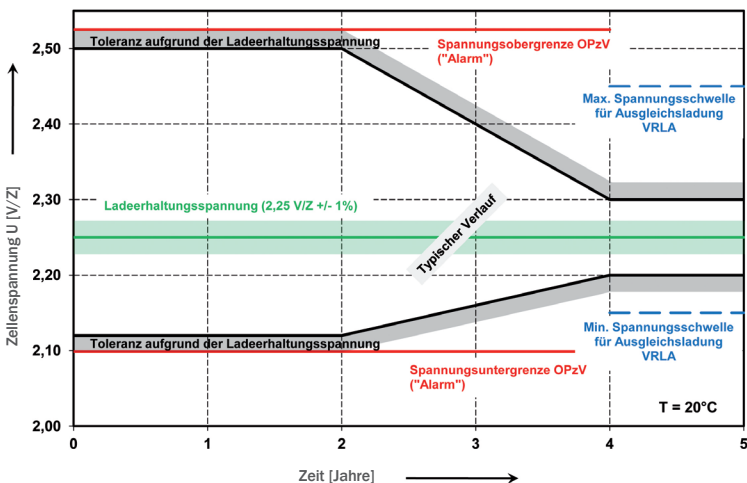
Abb. 6-4: Tendenzieller Verlauf der Ladeerhaltungsspannung über Gebrauchsdauer bei Gel-Batterien
