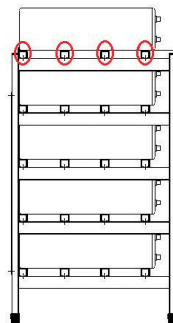
Zellen 12 OPzV 1500 Ah bis 24 OPzV 3000 Ah
