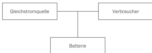
Abb. 6-2: Bereitschaftsparallelbetrieb
