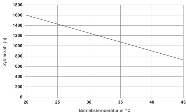
Abb. 7-9: Tendenzielle Haltbarkeit in Zyklen einer sun | power VR L (OPzV solar.power) als Funktion der Umgebungstemperatur
