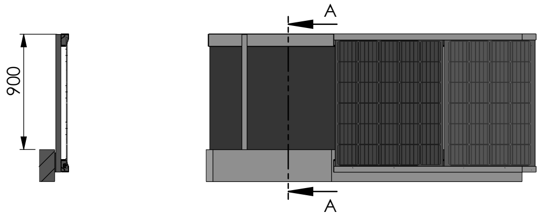
A-A (1 : 30)
