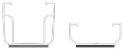
Kurzprofil C24 mit EPDM 385 mm
