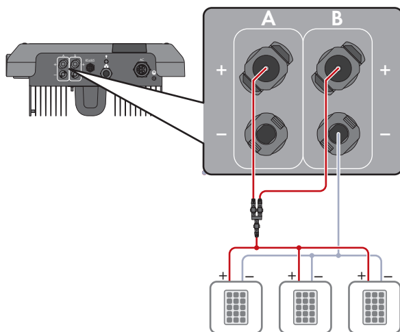
Figura 11: Panoramica del collegamento nel collegamento in parallelo degli ingressi CC A e B
