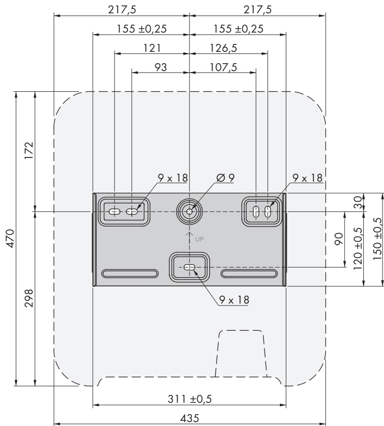
Figura 7: Posizione dei punti di fissaggio(Misure in mm/in)
