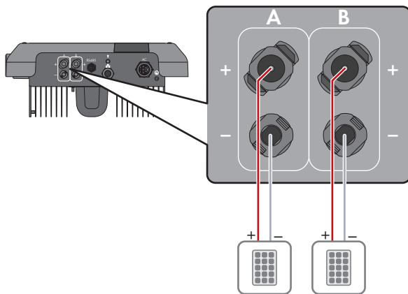
Figura 10: Panoramica del collegamento nel funzionamento normale
