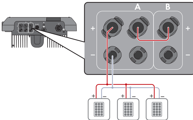
Figure 11 : Vue d'ensemble du raccordement en montage en parallèle des entrées DC A et B
