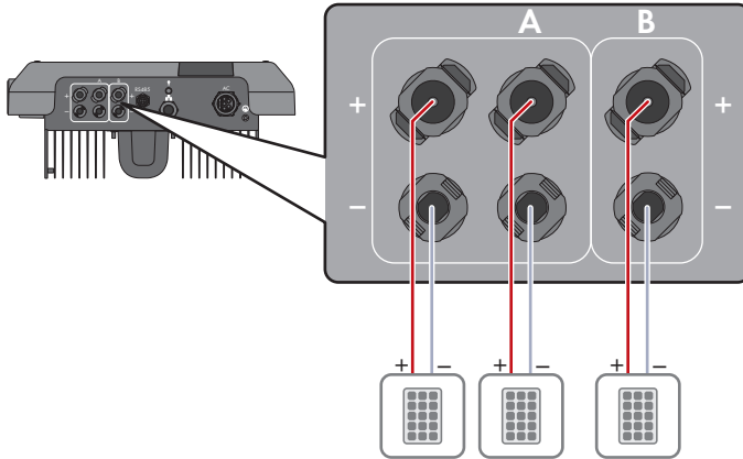
Figure 10 : Vue d'ensemble du raccordement en fonctionnement normal
