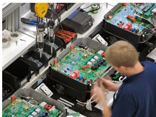
Endmontage von Wechselrichtern
