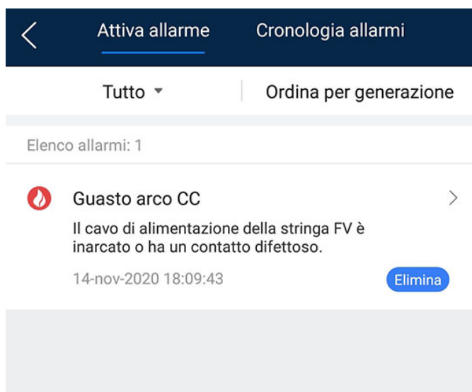
Figura 7-16 Gestione allarmi
