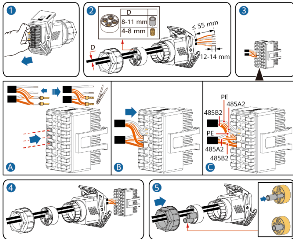
Figura 5-32 Installazione del cavo
