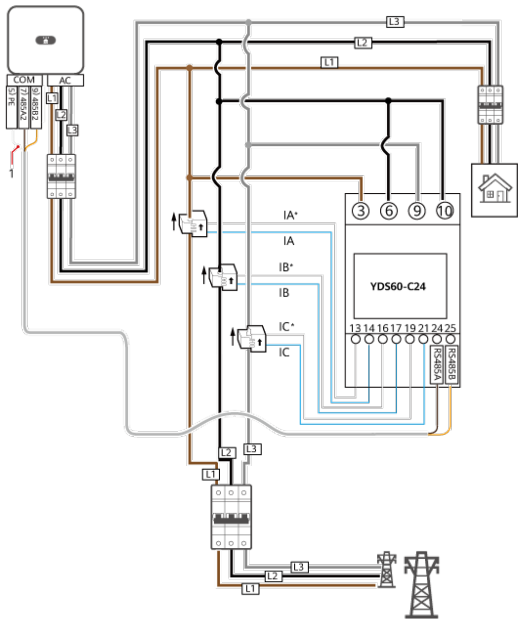
Figura 5-24 YDS60-C24 trifase, connessione via cavo a tre fili (rete Smart Dongle)
