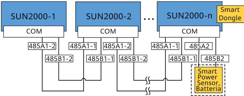
Figura 5-19 Rete Smart Dongle (il riquadro tratteggiato indica i componenti opzionali)
