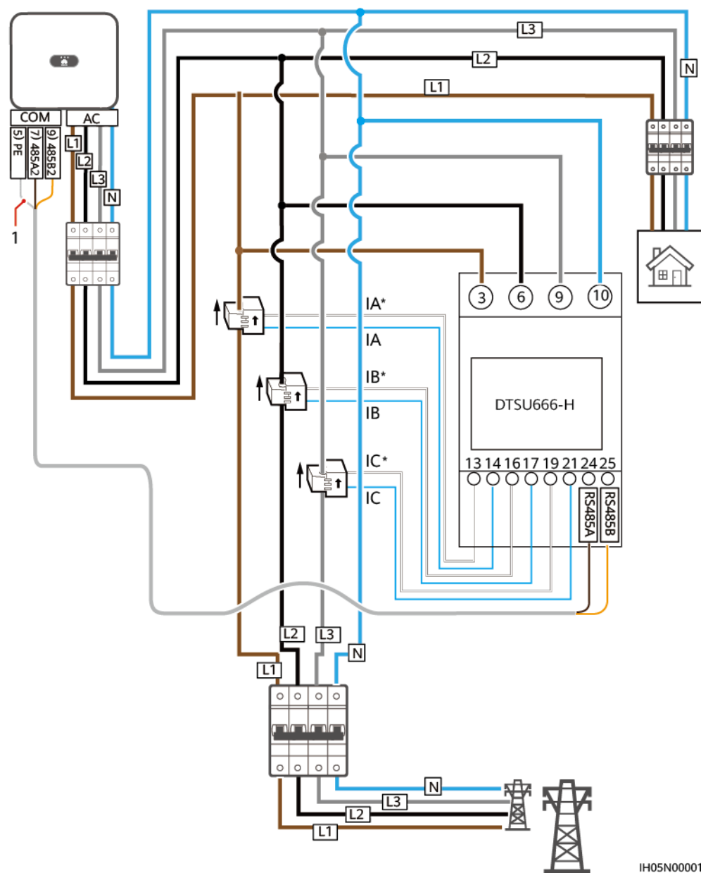
Figura 5-24 Collegamento dei cavi (Trifase a quattro fili)
