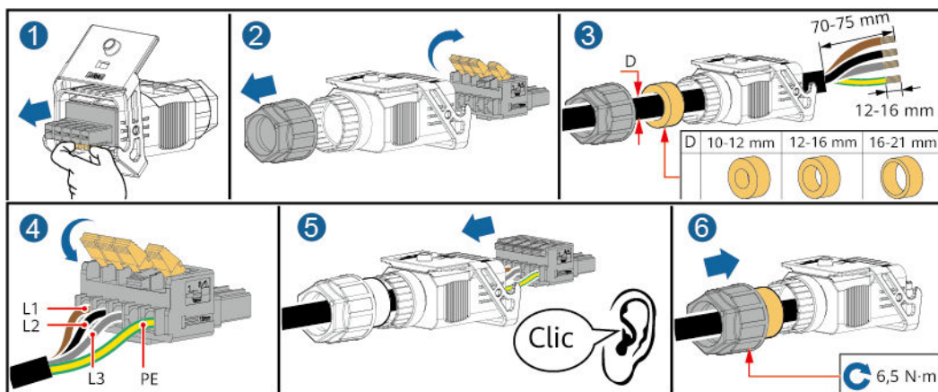
Figura 5-6 Cavo a quattro anime (L1, L2, L3 e PE)
