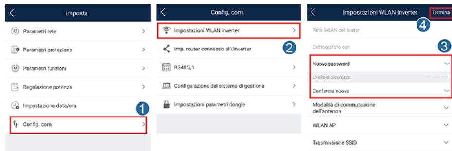
Figura C-4 Reimpostazione della password WLAN
