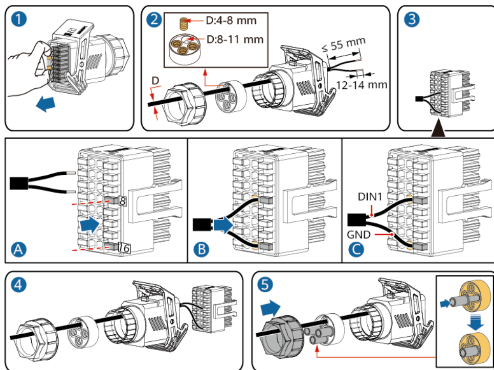
Figura 5-32 Installazione del cavo
