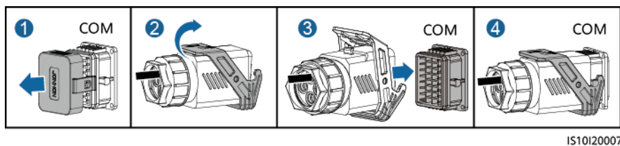
Figura 5-31 Fissaggio del connettore del cavo di segnale
