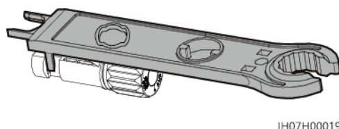
Figura 5-14 Rimozione dei connettori CC
