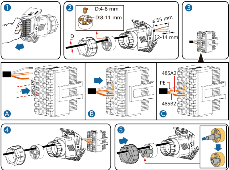
Figura 5-25 Installazione del cavo
