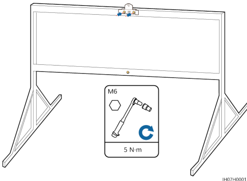
Figura 4-15 Fissaggio della staffa di montaggio
