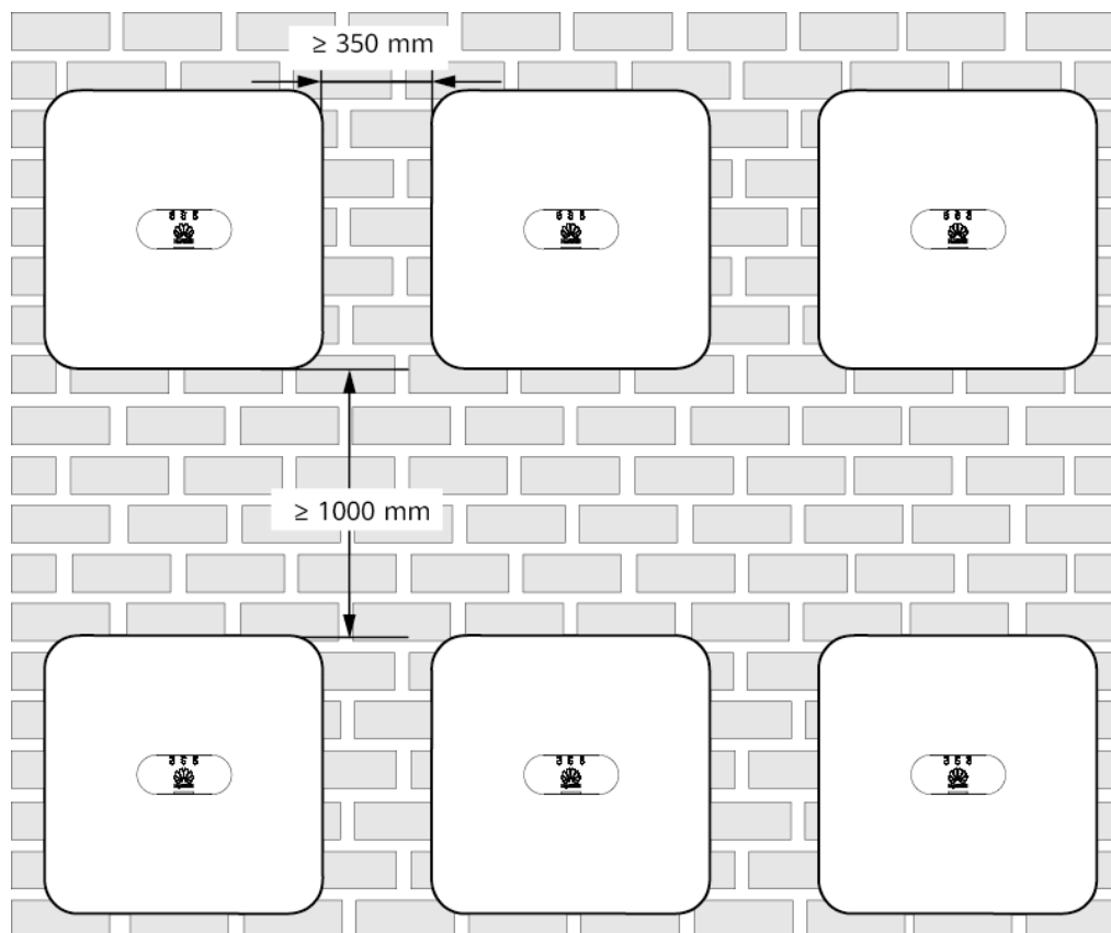
Figura 4-5 Installazione impilata (non consigliata)
