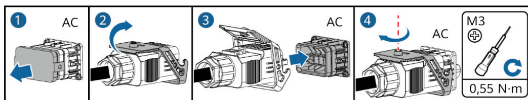
Figura 5-9 Fissaggio del connettore CA
