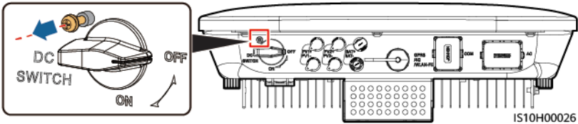
Figura 6-1 Rimozione della vite di bloccaggio da un interruttore CC
