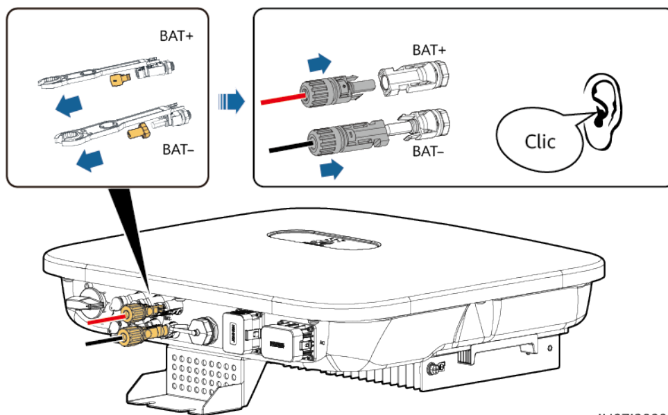
Figura 5-15 Collegamento dei cavi della batteria
