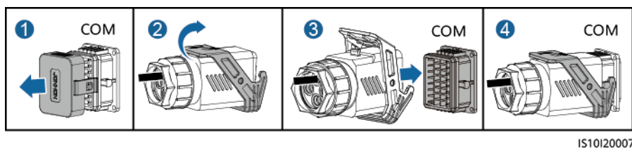
Figura 5-26 Fissaggio del connettore del cavo di segnale
