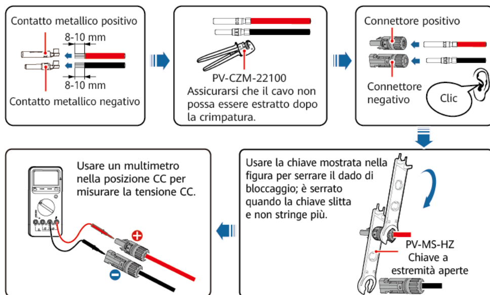
Figura 5-13 Installazione dei cavi di alimentazione di ingresso CC
