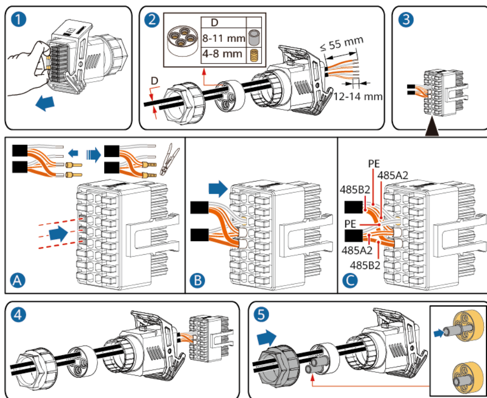
Figura 5-27 Installazione del cavo
