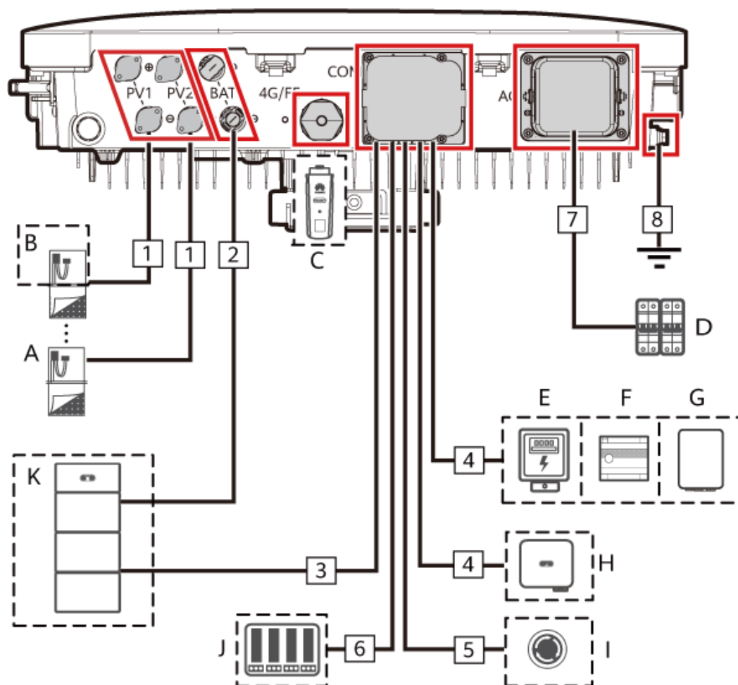
Figure 5-1 Connexions des câbles de l'onduleur (les cases en pointillé indiquent des composants facultatifs)
