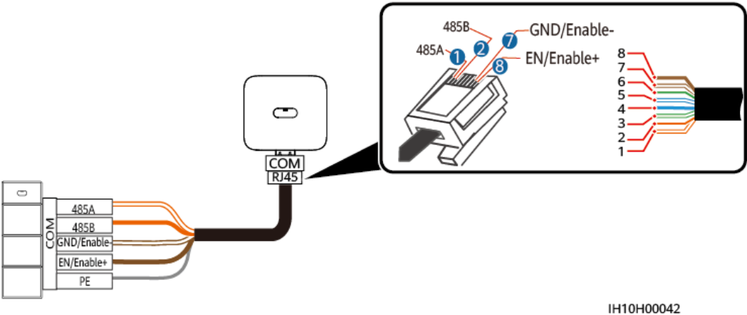
Figure 5-41 Connexion des câbles
