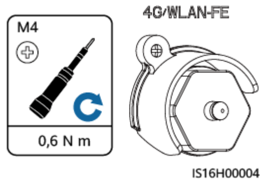
Figure 5-46 Installation des composants antivol du Smart Dongle
