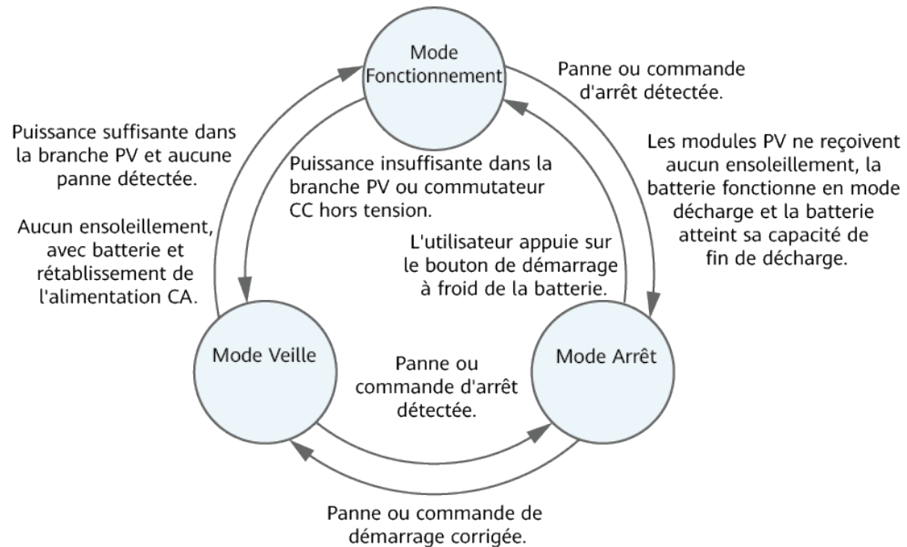
Figure 2-6 Modes de fonctionnement
