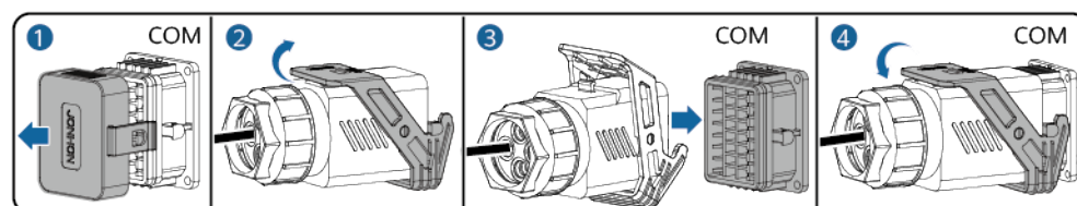
Figure 5-43 Fixation du connecteur du câble de signal
