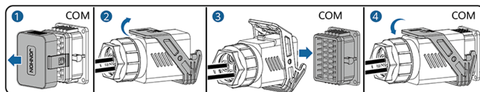
Figure 5-26 Fixation du connecteur du câble de signal
