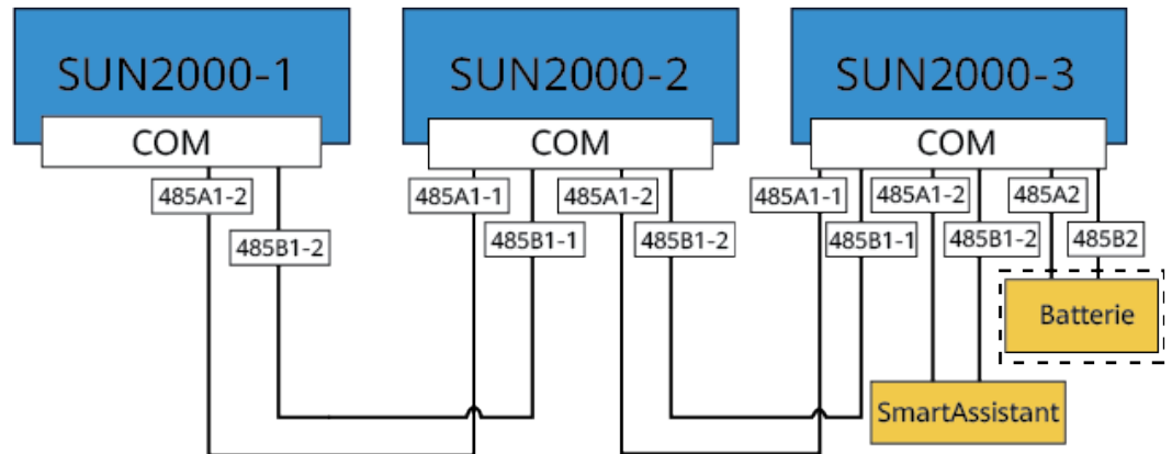
Figure 5-23 Mise en réseau du SmartAssistant (les composants dans les encadrés en pointillé sont facultatifs)
