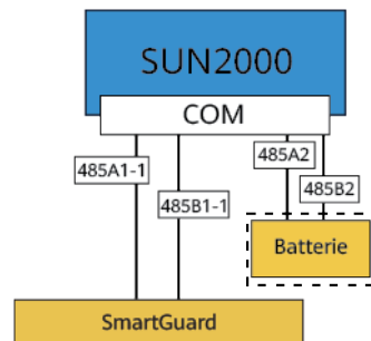
Figure 5-24 Mise en réseau du SmartGuard (les composants dans les encadrés en pointillé sont facultatifs)
