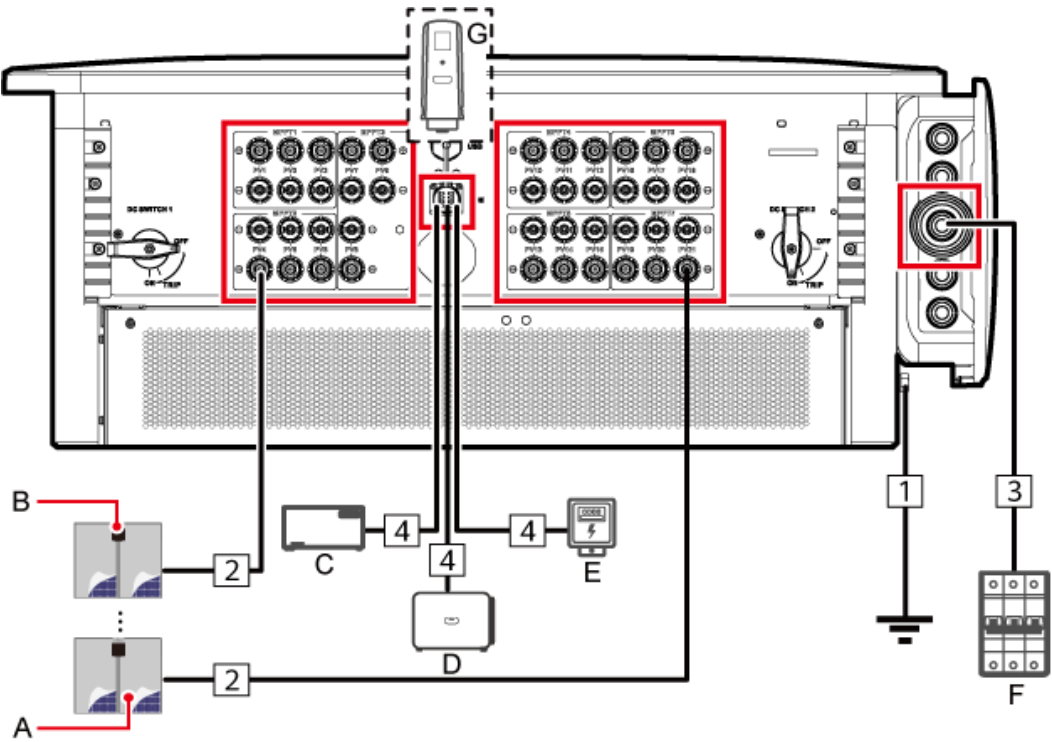
Figure 5-1 Connexions de câbles (configurez les composants dans la zone en pointillés selon les exigences applicables)
