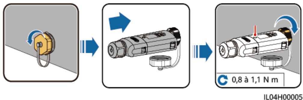
Figure 5-20 Installation du Smart Dongle WLAN-FE (SDongleA-05 pour le scénario de communication WLAN)
