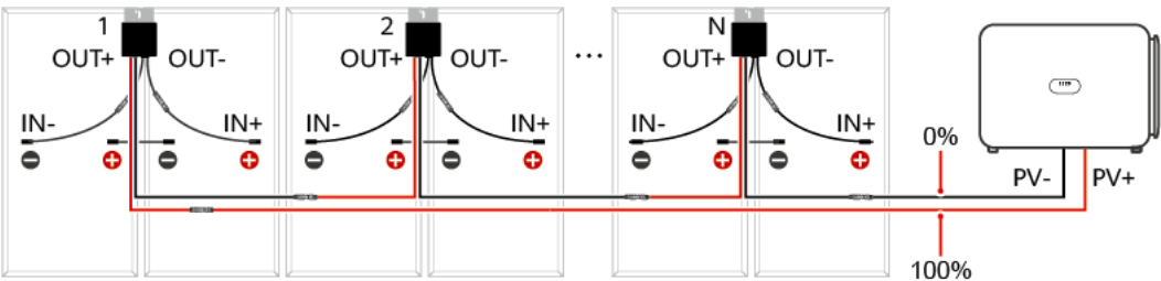
Figure 8-16 Définition du pourcentage de la localisation de court-circuit
