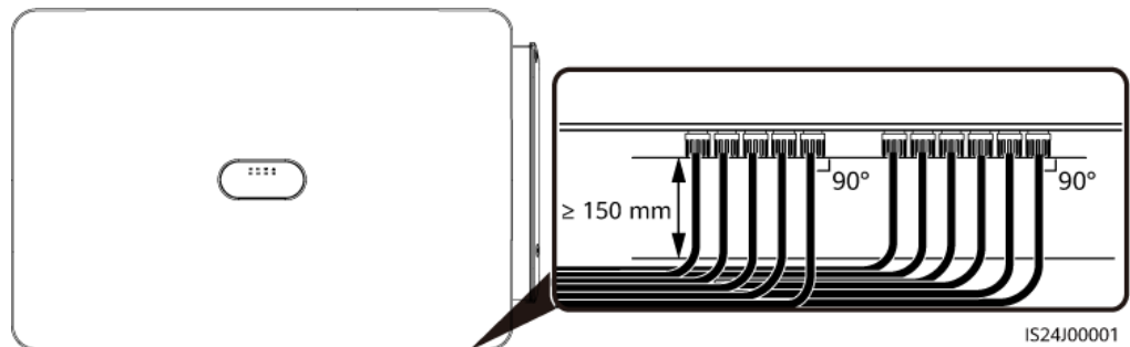
Figure 5-13 Exigences en matière de câblage d'alimentation d'entrée CC
