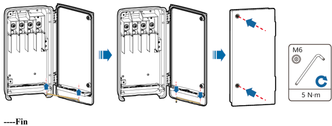
Figure 5-9 Fermeture d'une porte
