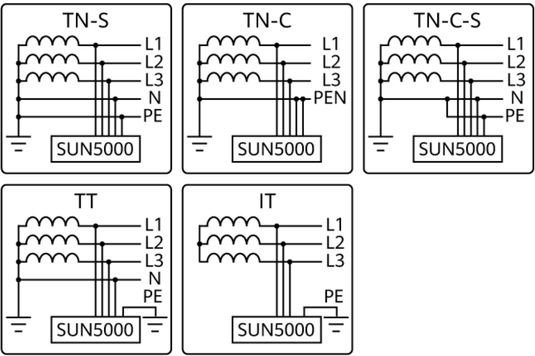
Figure 2-6 Systèmes de mise à la terre
