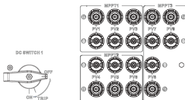
Figure 5-11 Terminaux CC contrôlés par DC SWITCH 1
