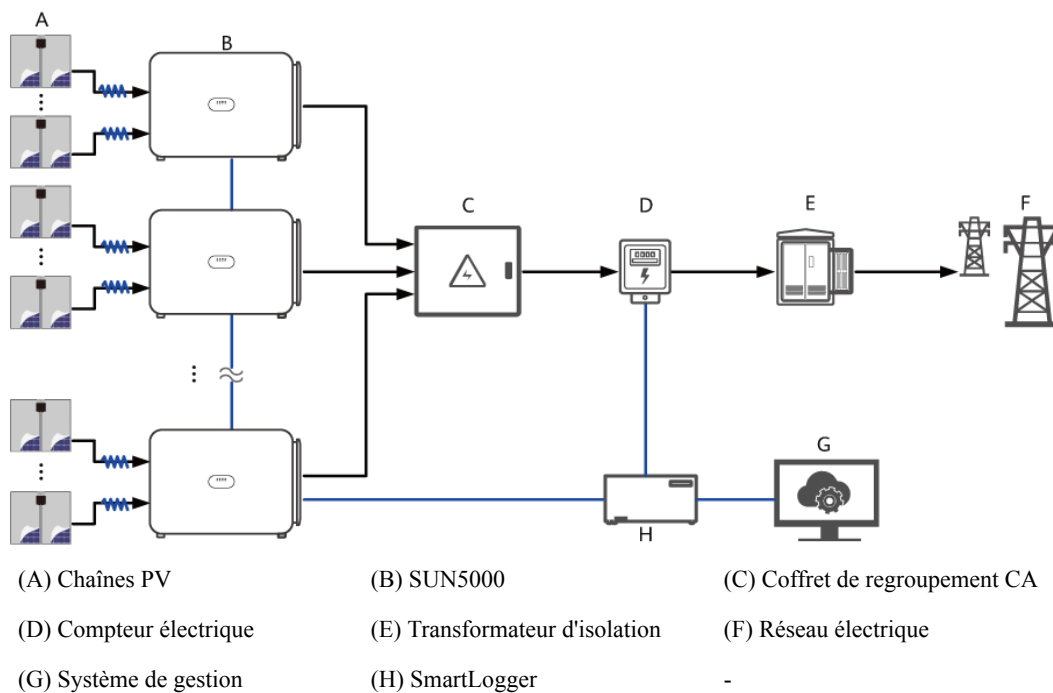
Figure 2-2 Application de mise en réseau RS485 (SmartLogger)
