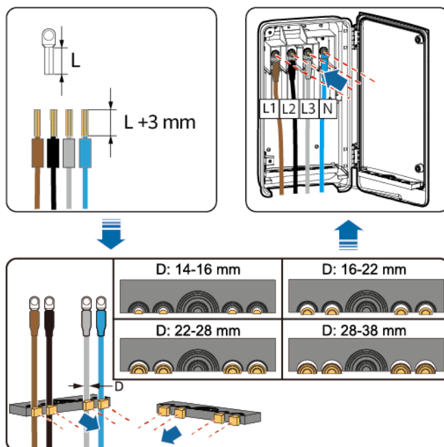
Figure 5-7 Connexion de câble monoconducteur
