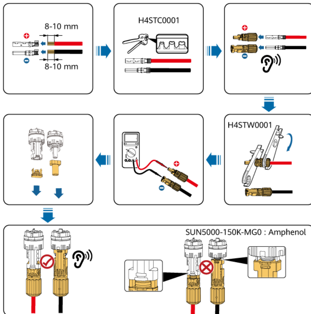
Figure 5-15 Connexion des câbles d'alimentation d'entrée CC (Amphenol)
