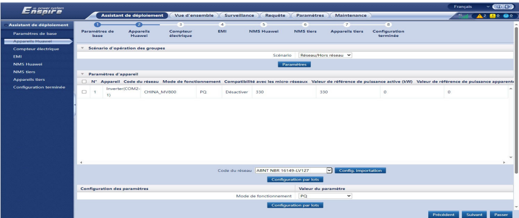
Figure 7-4 Paramétrage du code du réseau
