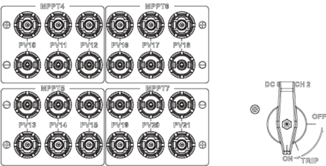
Figure 5-12 Terminaux CC contrôlés par DC SWITCH 2
