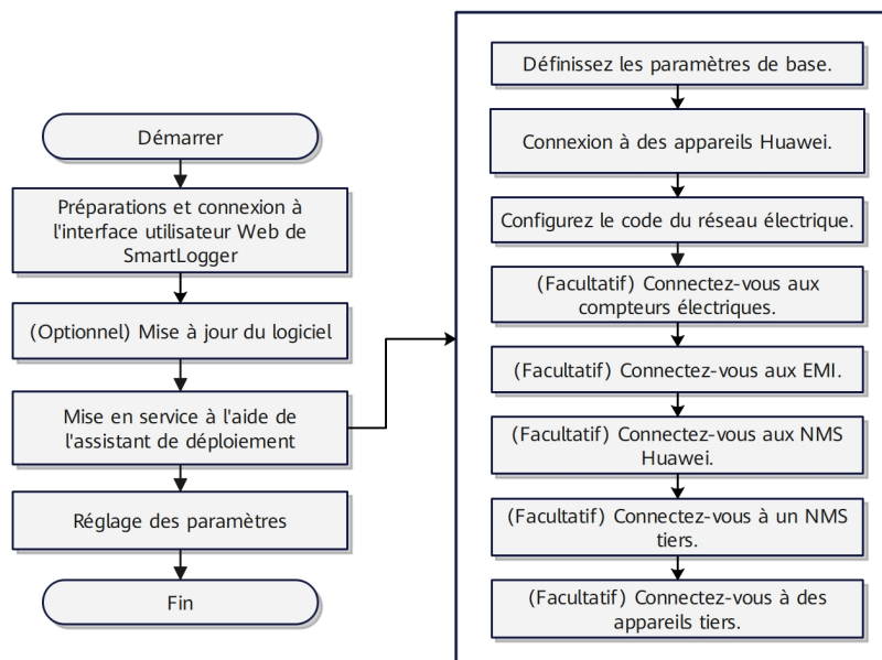
Figure 7-1 Processus de mise en service sur l'interface utilisateur Web SmartLogger
