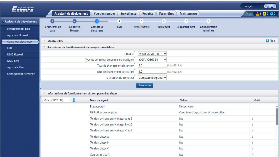
Figure 7-5 Connexion à des compteurs électriques
