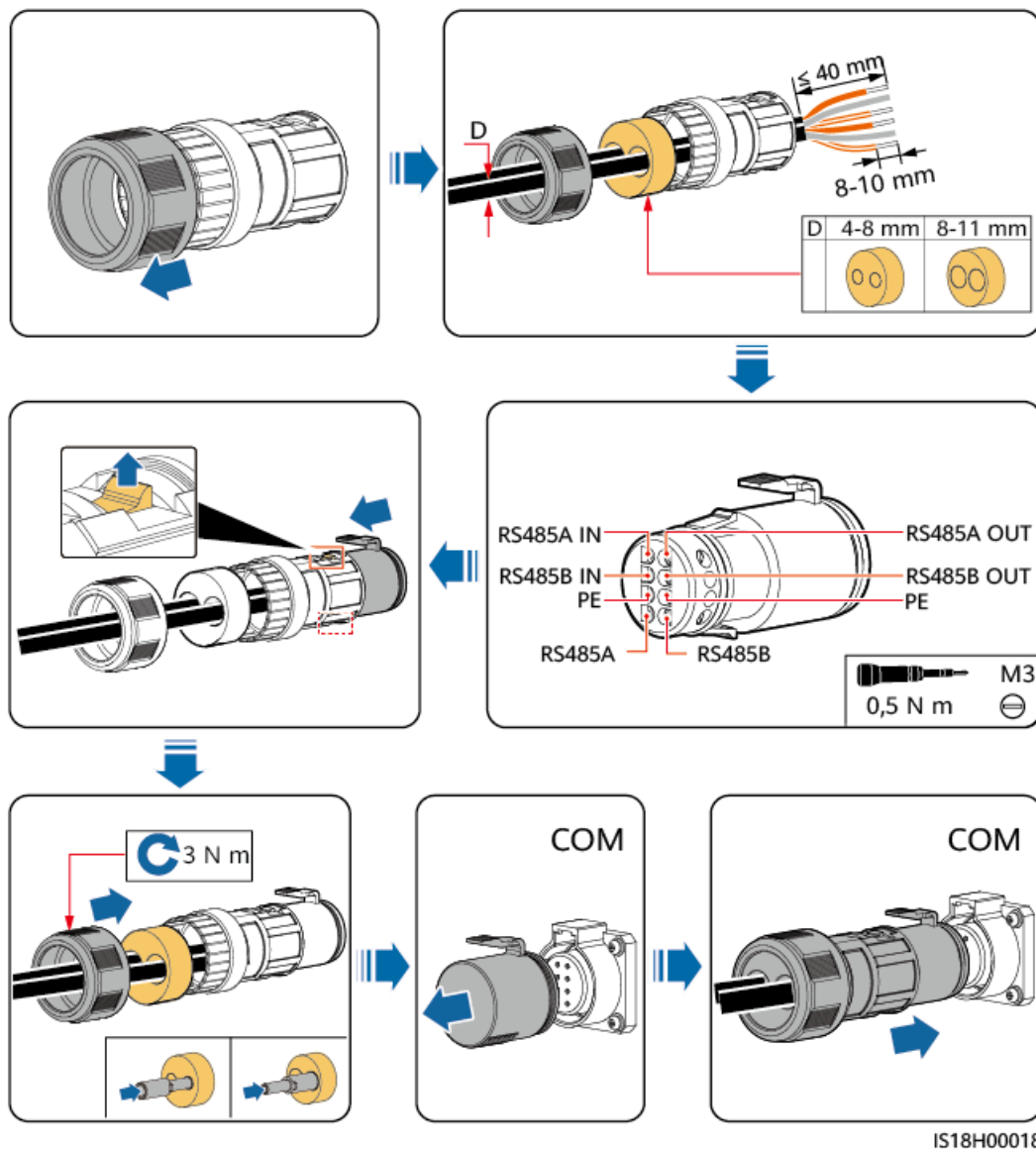
Figure 5-18 Connexion des câbles de communication
