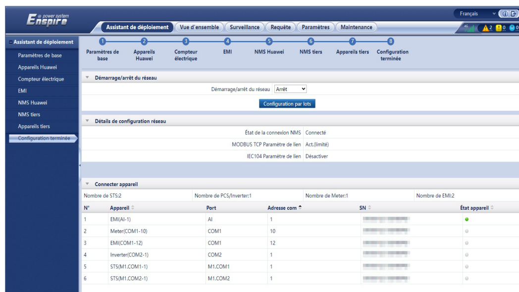
Figure 7-10 Fin de la configuration
