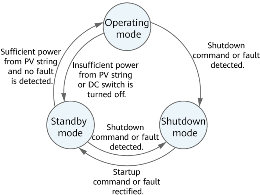
Figure 2-10 Modes de fonctionnement
