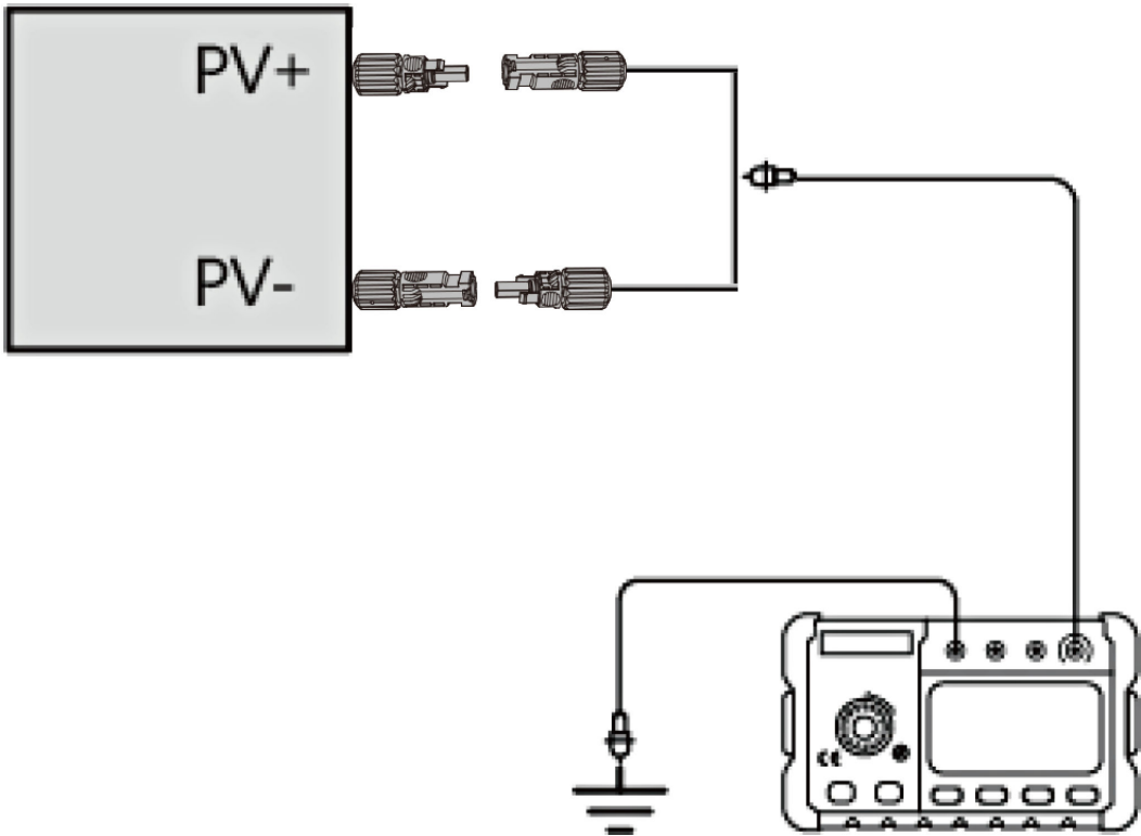
Figure 5-10 Test de la résistance d'isolation
