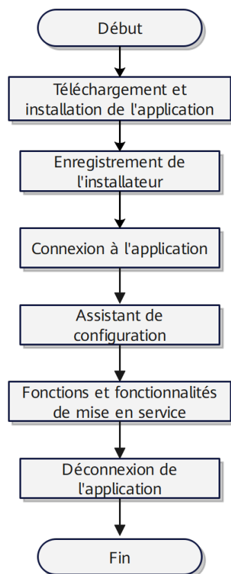
Figure 7-2 Processus de mise en service sur l'application FusionSolar
