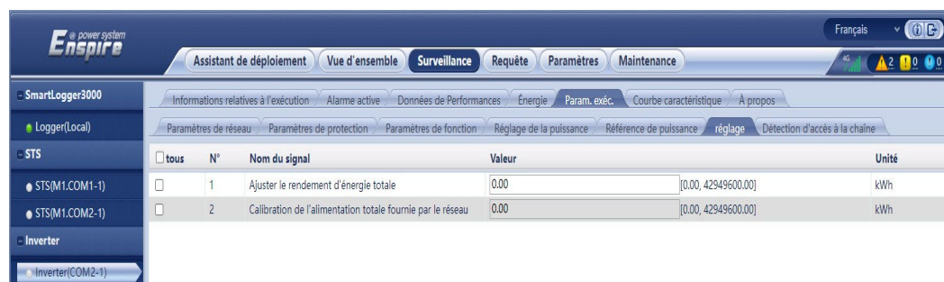
Figure 7-11 Réglage des paramètres de fonctionnement
