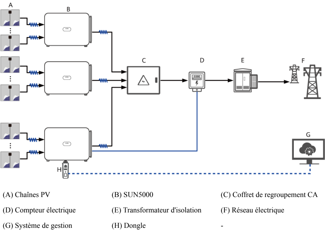
Figure 2-5 Application de mise en réseau du MBUS (Dongle)
