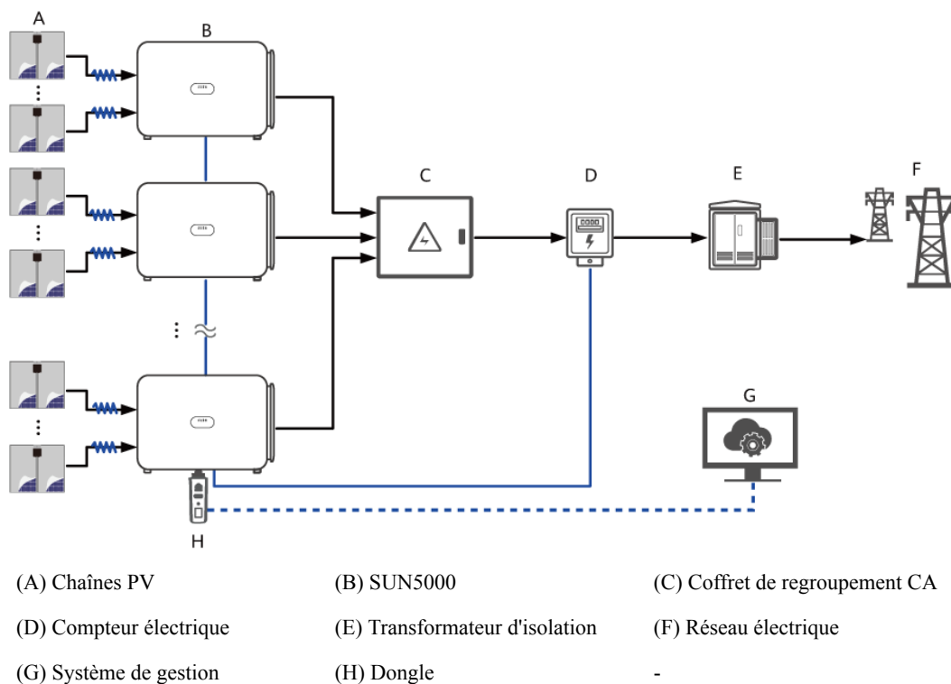
Figure 2-3 Application de mise en réseau RS485 (Dongle)
