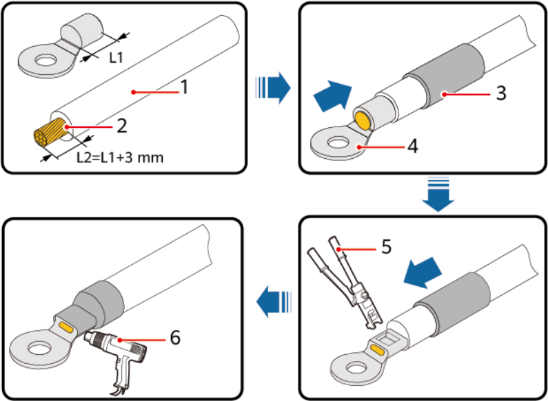
Figure E-2 Sertissage d'une borne OT
