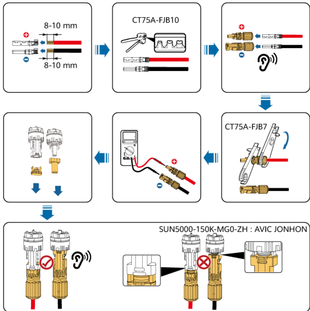
Figure 5-14 Connexion des câbles d'alimentation d'entrée CC(AVIC JONHON)
