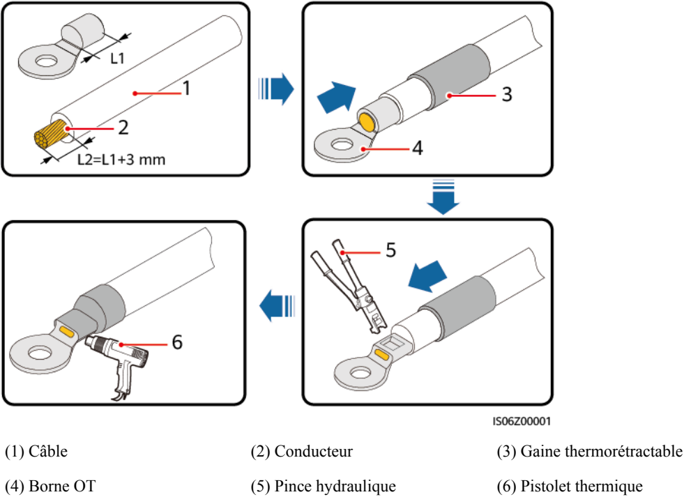
Figure E-2 Sertissage d'une borne OT
