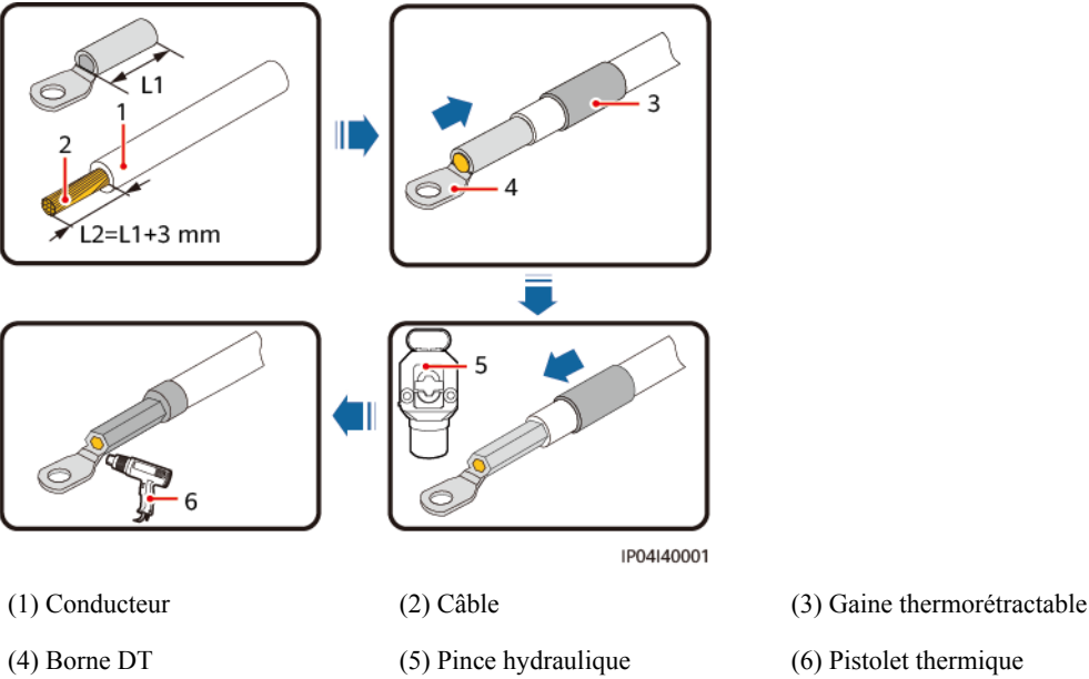
Figure E-3 Sertissage d'une borne DT
