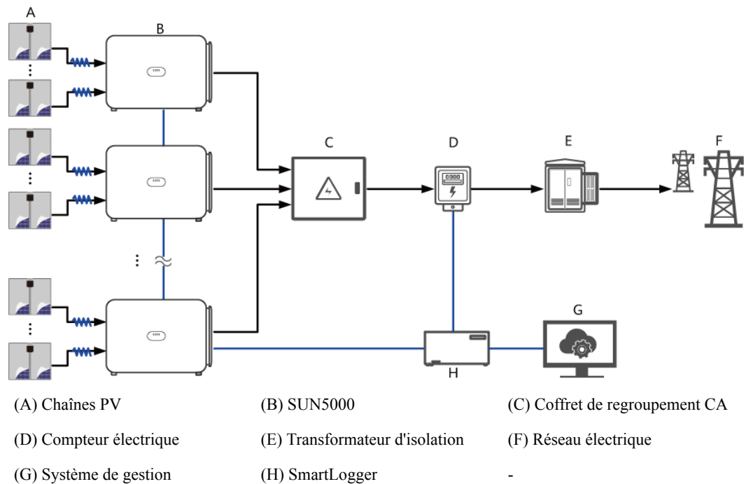
Figure 2-2 Application de mise en réseau RS485 (SmartLogger)
