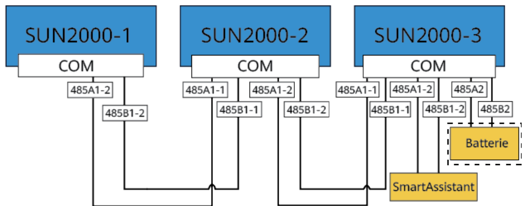
Figure 5-19 Mise en réseau SmartAssistant (les composants dans les encadrés en pointillé sont facultatifs)
