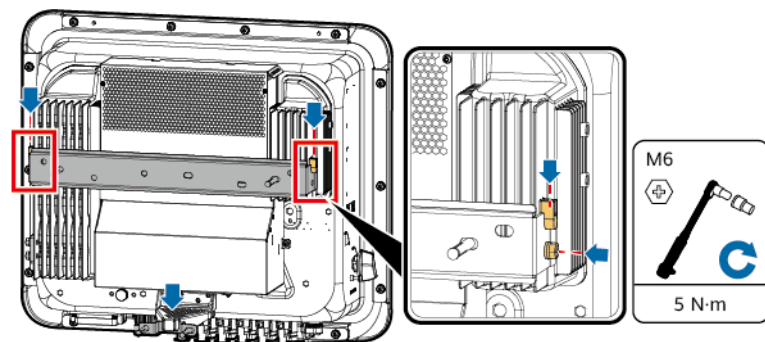
Figure 4-8 Installation de l'onduleur
