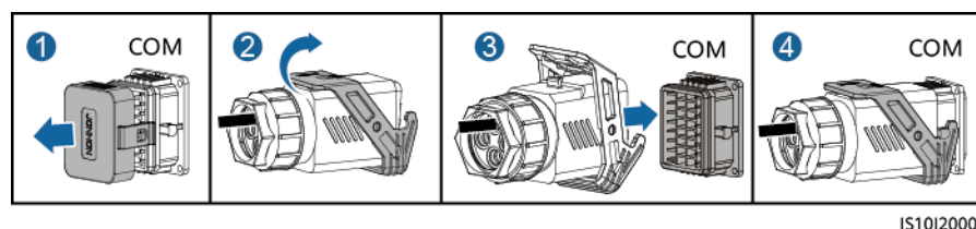
Figure 5-27 Fixation du connecteur du câble de signal
