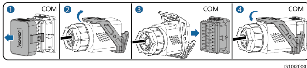
Figure 5-41 Fixation du connecteur du câble de signal
