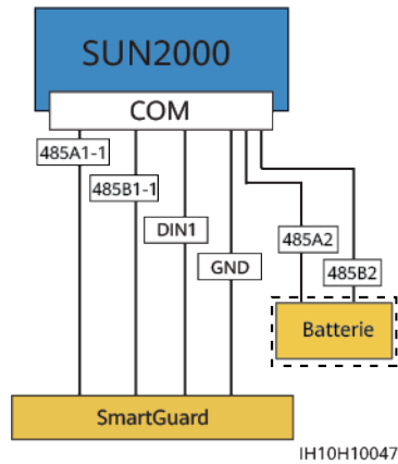
Figure 5-20 Mise en réseau SmartGuard (les composants dans les encadrés en pointillés sont facultatifs)
