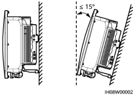
Figure 4-5 Angle d'installation
