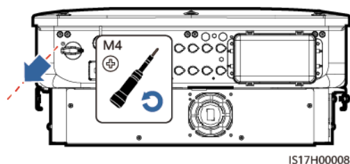
Abbildung 6-1 Entfernen der DC SWITCH-Sicherungsschraube
