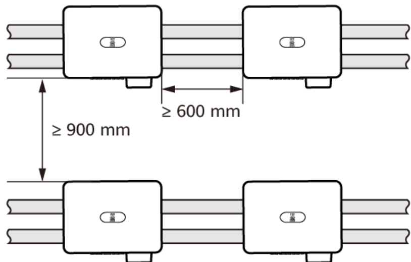
Abbildung 4-7 Gestapelte Installation auf Stützen (empfohlen)
