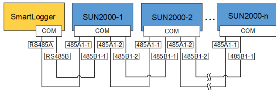
Abbildung 5-21 SmartLogger-Vernetzung
