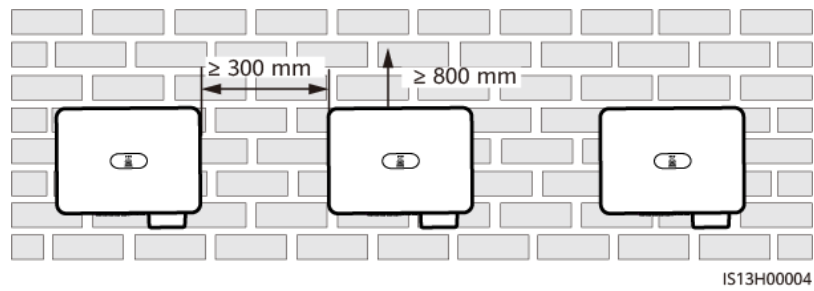
Abbildung 4-3 Horizontale Installation (empfohlen)
