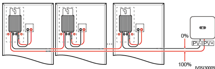
Abbildung K-2 Prozentsatz der Kurzschlusspositionen
