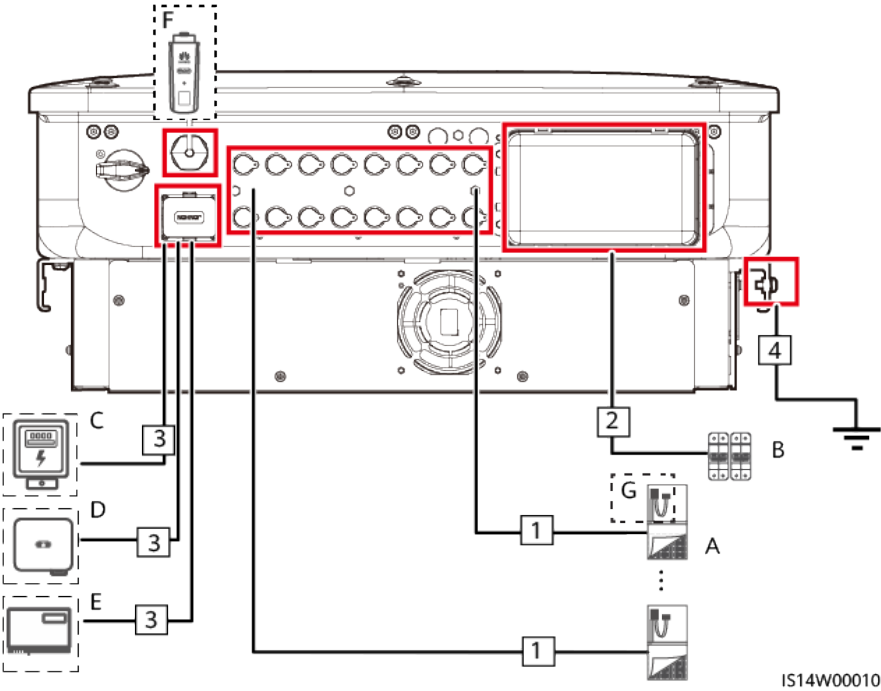
Abbildung 5-1 SUN2000-Kabelverbindungen (die Komponenten in gestrichelten Kästchen sind optional)
