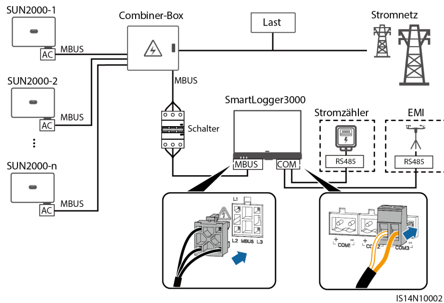
Abbildung 5-23 MBUS-Kommunikation (C&I-Szenario in China)
