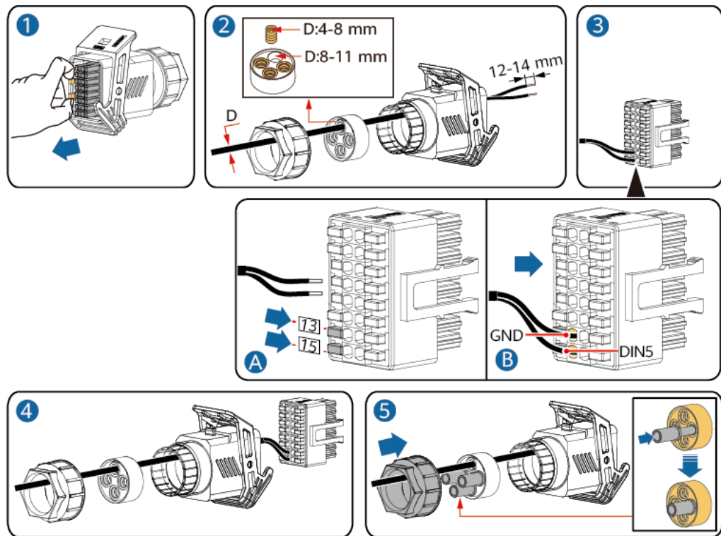
Abbildung 5-30 Installieren des Kabels
