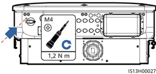
Abbildung 8-1 Montage der Sicherungsschraube des DC-Schalters
