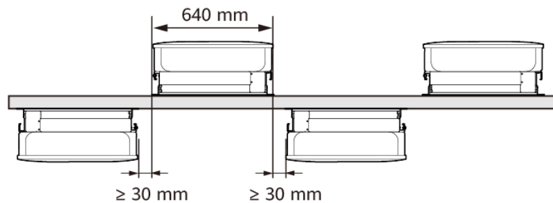
Abbildung 4-8 Versetzte Rücken-an-Rücken-Installation auf einer Stütze (empfohlen)
