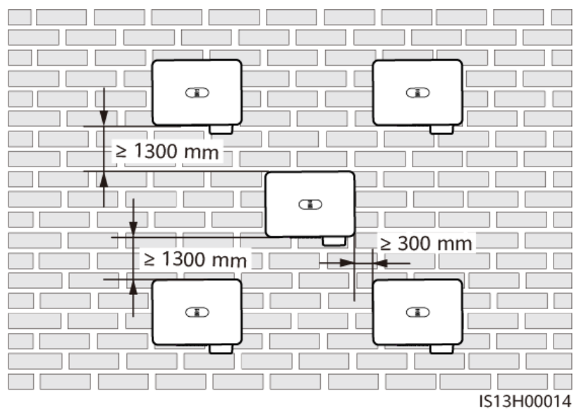
Abbildung 4-5 Dreischichtige Dreiecks-Installation (nicht empfohlen)
