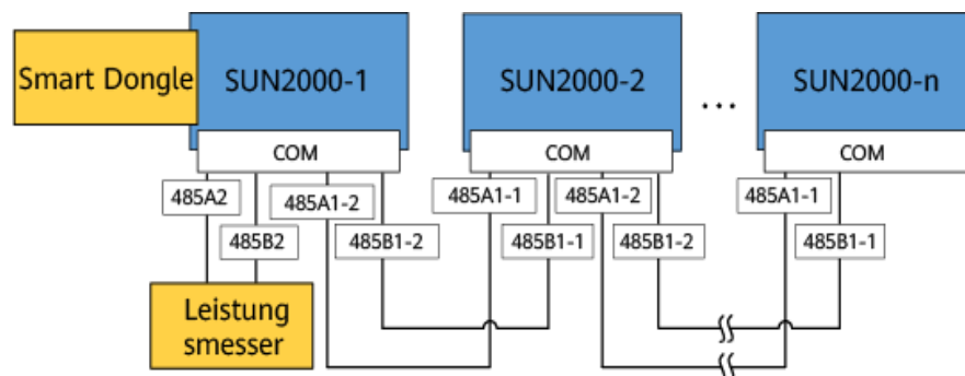
Abbildung 5-20 Smart Dongle-Vernetzung
