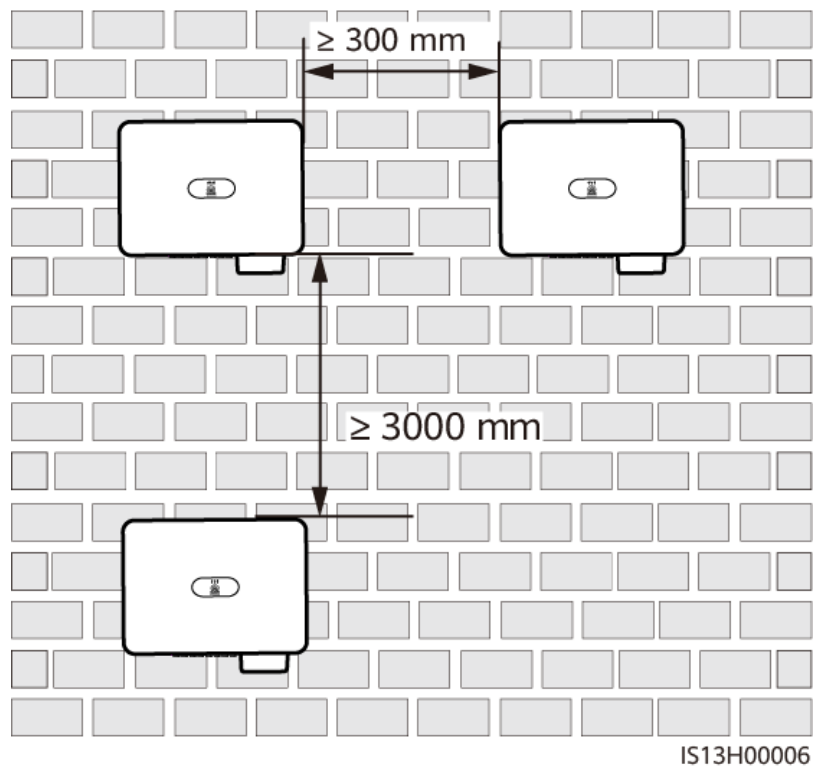
Abbildung 4-6 Gestapelte Installation an der Wand (nicht empfohlen)
