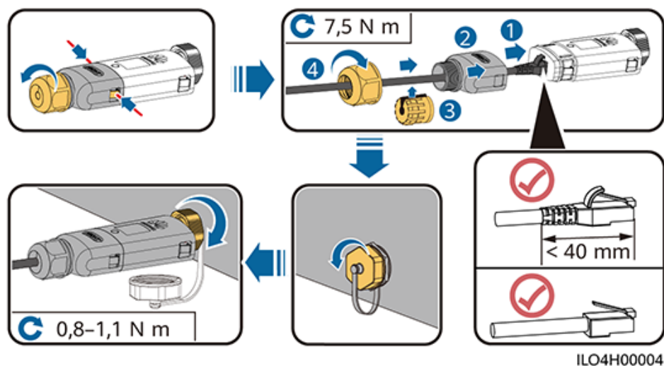
Abbildung 5-17 Anschließen des WLAN-FE Smart Dongle (FE-Kommunikation)
