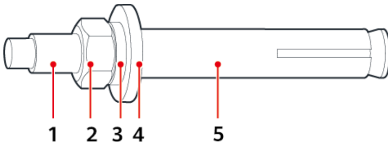
Abbildung 4-14 Struktur der Dehnschraube
