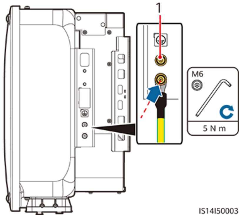
Abbildung 5-3 Anschließen eines PE-Kabels
