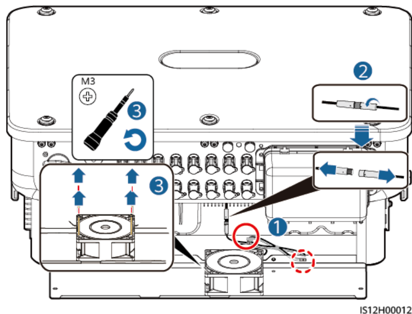
Abbildung 8-4 Entfernen des defekten Lüfters
