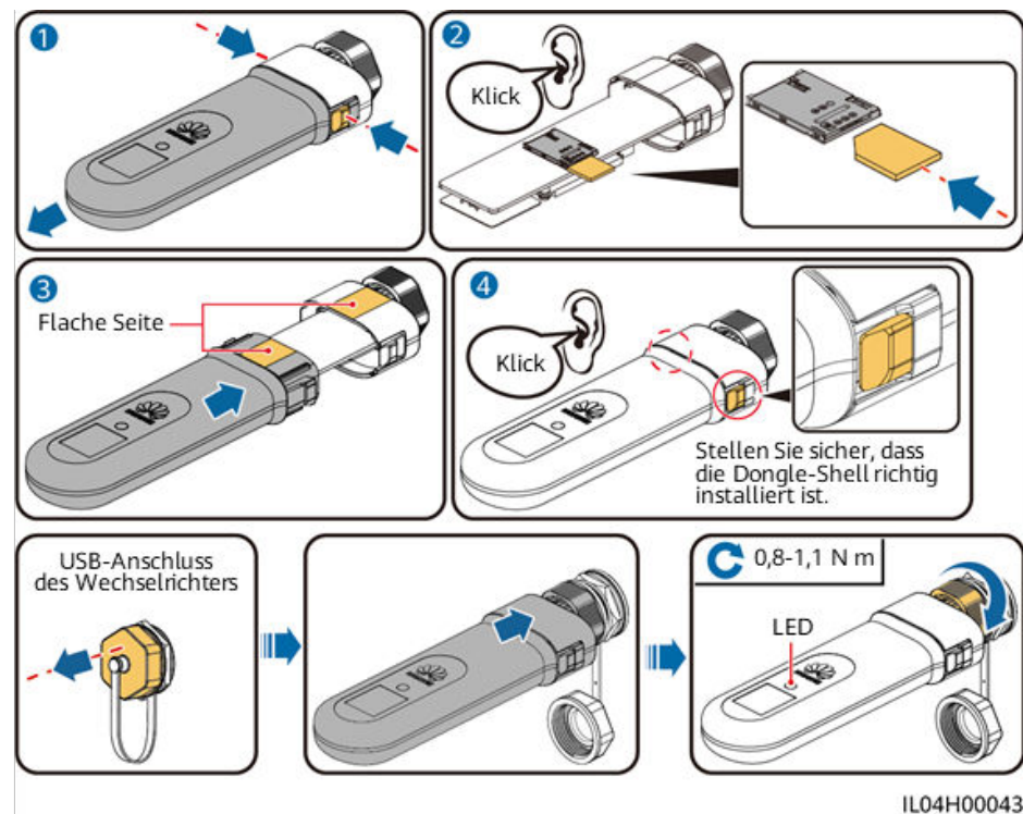
Abbildung 5-15 Installation des 4G Smart Dongle (SDongleB-06)
