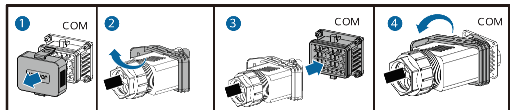
Abbildung 5-27 Sichern des Signalkabelsteckers
