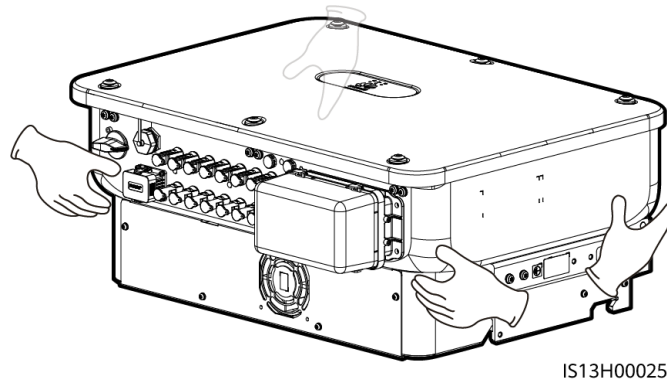
Abbildung 4-10 Transportieren des Wechselrichters
