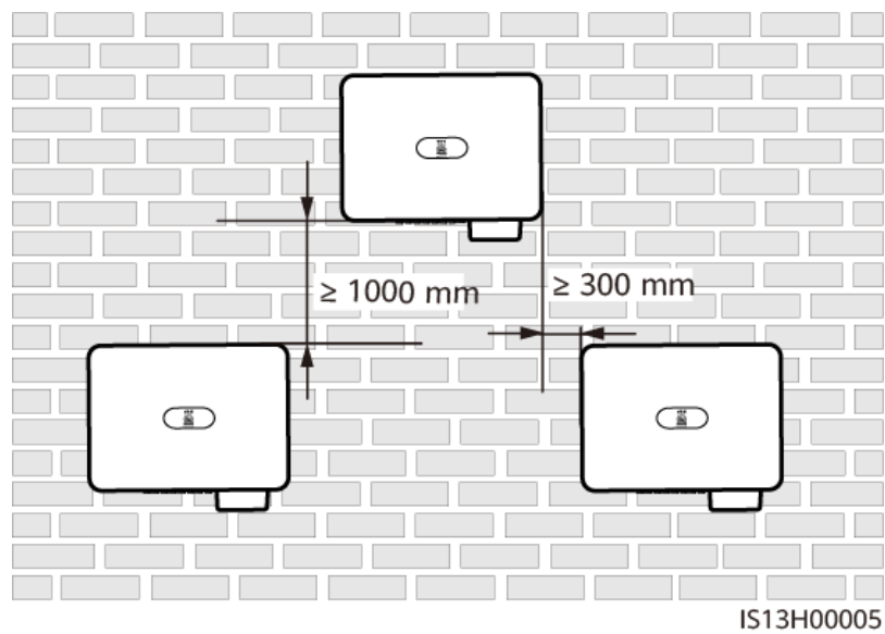
Abbildung 4-4 Zweischichtige Dreiecks-Installation (nicht empfohlen)
