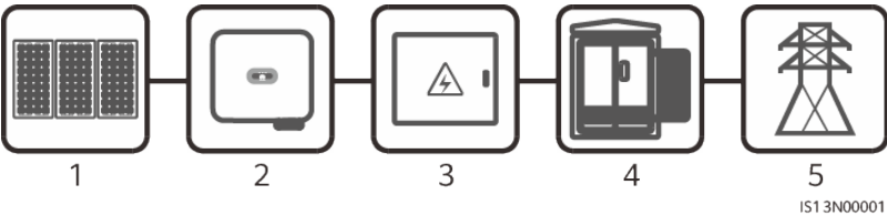
Abbildung 2-2 Vernetzungsanwendung – Szenario mit einem einzelnen Wechselrichter
