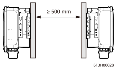
Abbildung 4-9 Rücken-an-Rücken-Installation auf Stützen (nicht empfohlen)
