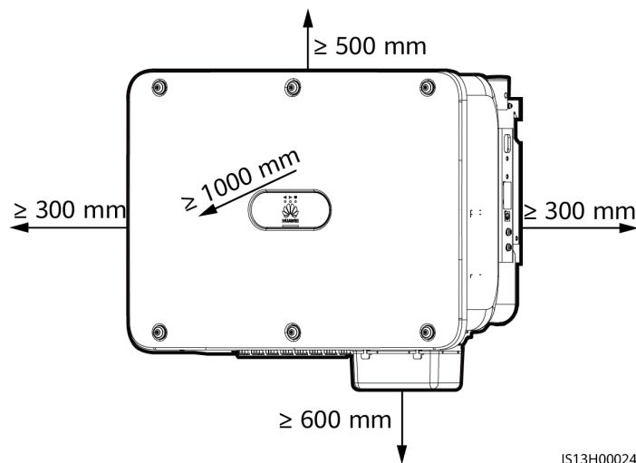
Abbildung 4-2 Abstände
