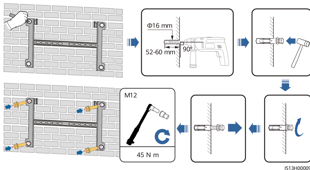
Abbildung 4-15 Einsetzen einer Dehnschraube
