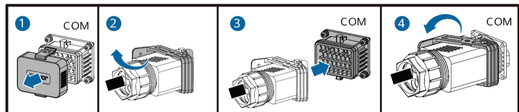
Abbildung 5-31 Sichern des Signalkabelsteckers
