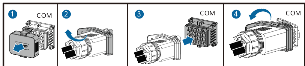
Abbildung 5-25 Sichern des Signalkabelsteckers
