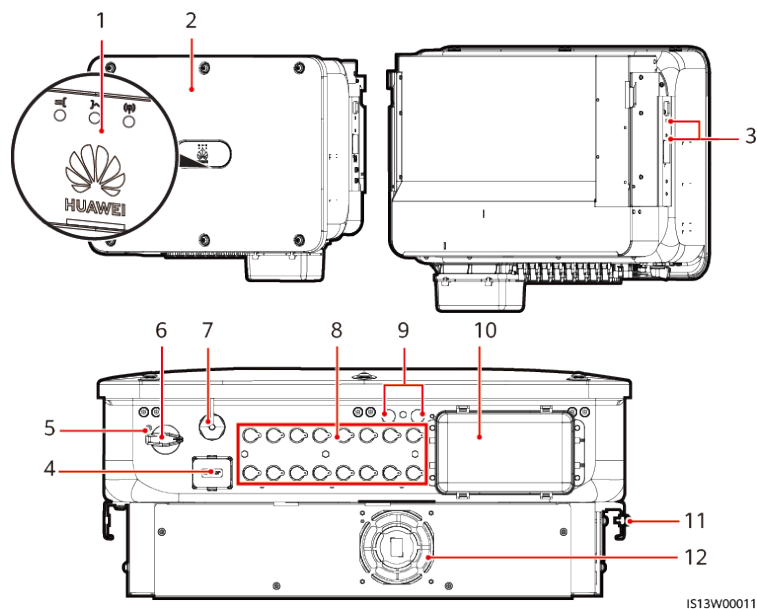
Abbildung 2-4 Erscheinungsbild
