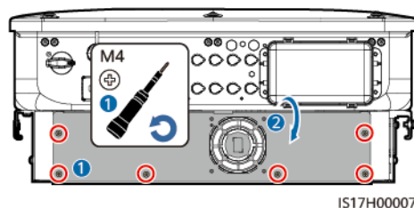
Abbildung 8-3 Entfernen der Schrauben von der Lüftermontageplatte
