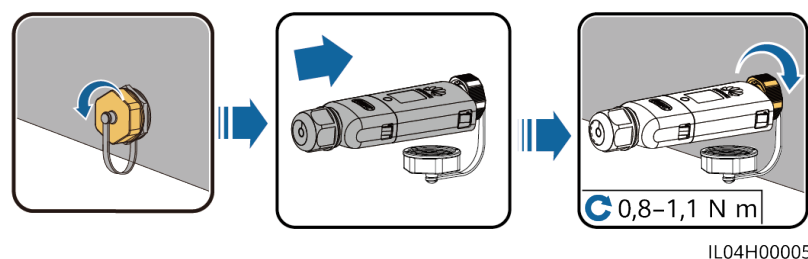
Abbildung 5-16 Anschließen des WLAN-FE Smart Dongle (WLAN-Kommunikation)
