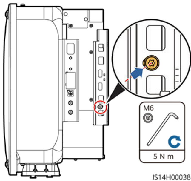
Abbildung 4-18 Anziehen der Muttern
