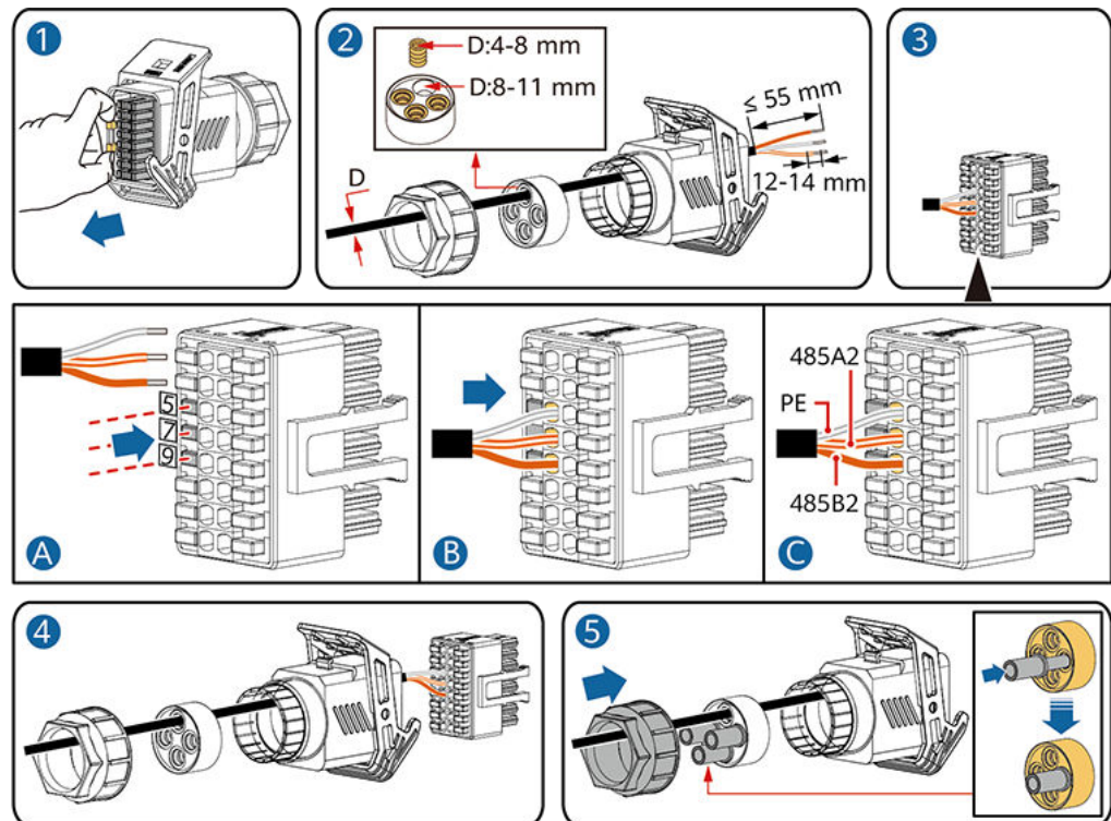
Abbildung 5-26 Installieren des Kabels
