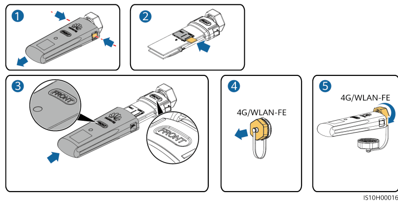
Abbildung 5-14 Installation des 4G Smart Dongle (SDongleA-03)
