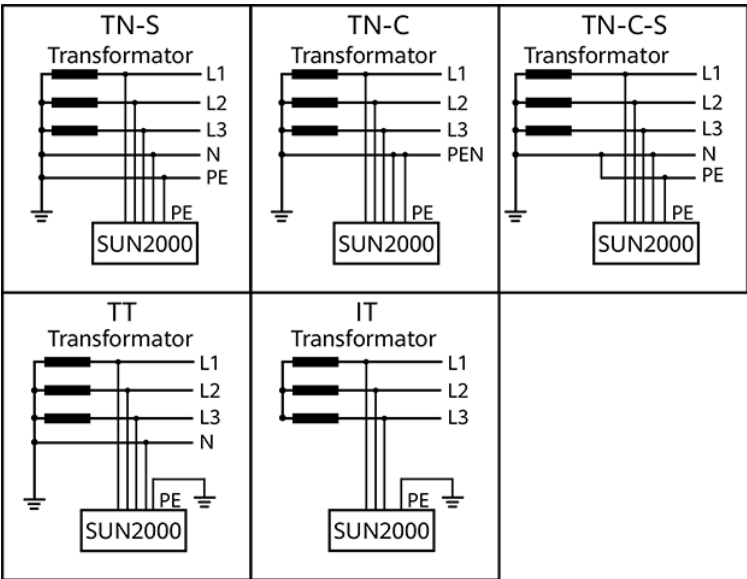
Abbildung 2-3 Erdungssysteme
