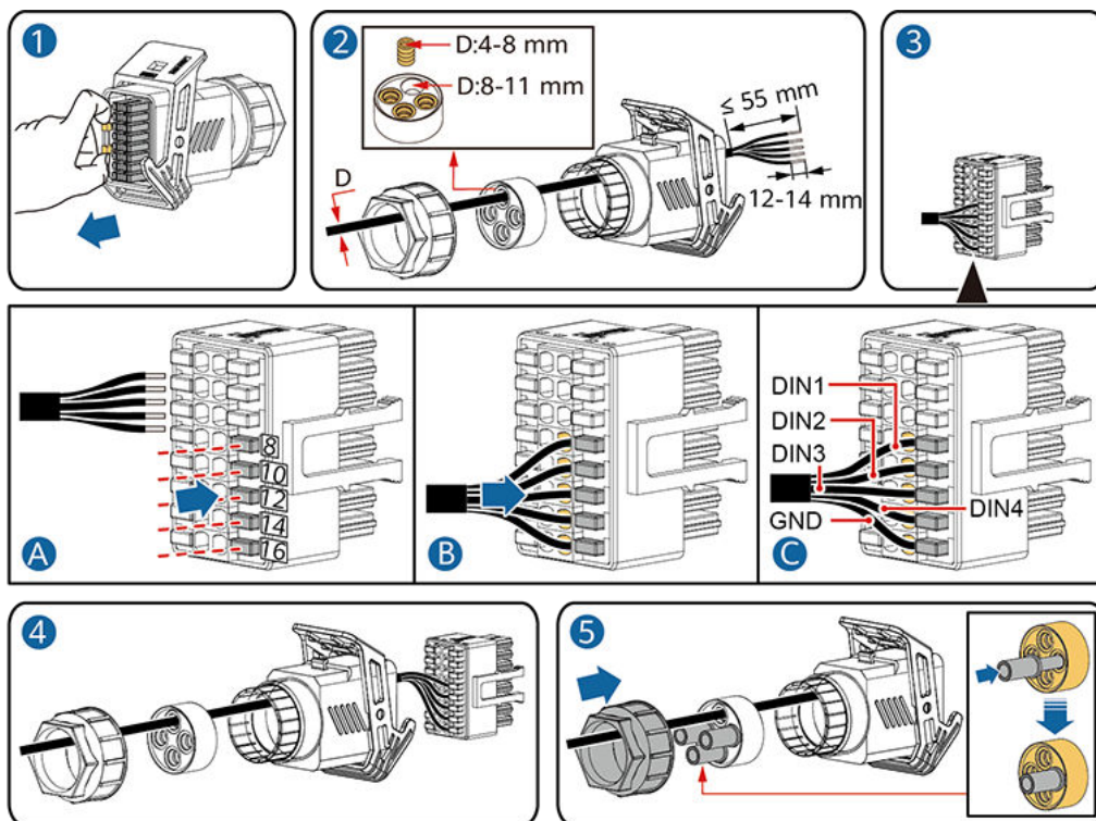
Abbildung 5-28 Anschließen des Kabels
