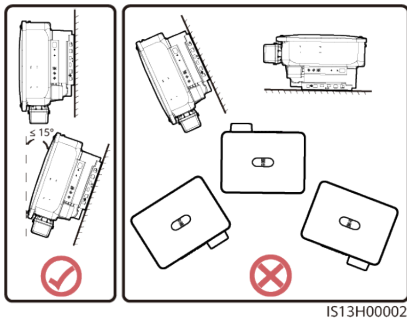
Abbildung 4-1 Installationswinkel
