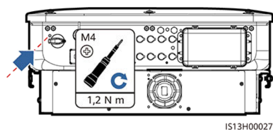
Abbildung 4-16 Montage der Sicherungsschraube des DC-Schalters
