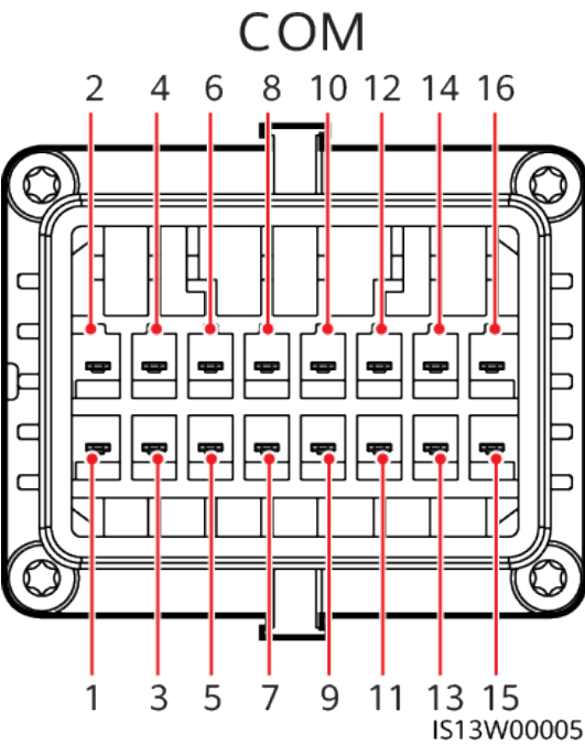
Abbildung 5-18 Pin-Belegung
