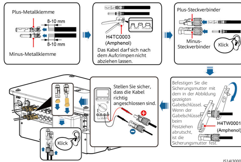
Abbildung 5-13 Anschließen der DC-Stromkabel
