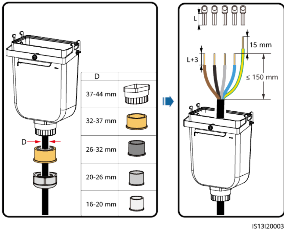
Abbildung 5-6 Abisolieren eines AC-Stromkabels (verwenden Sie beispielsweise ein fünfadriges Kabel)
