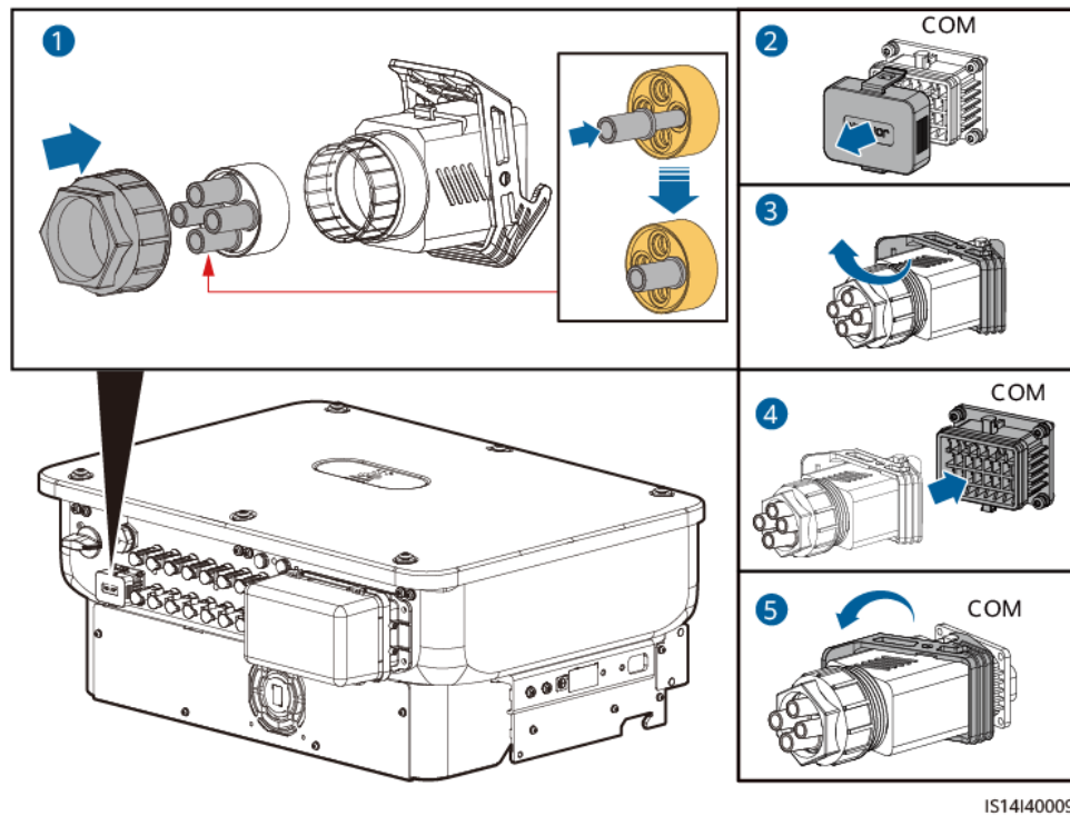
Abbildung 5-19 Anschließen des Signalkabelsteckverbinders
