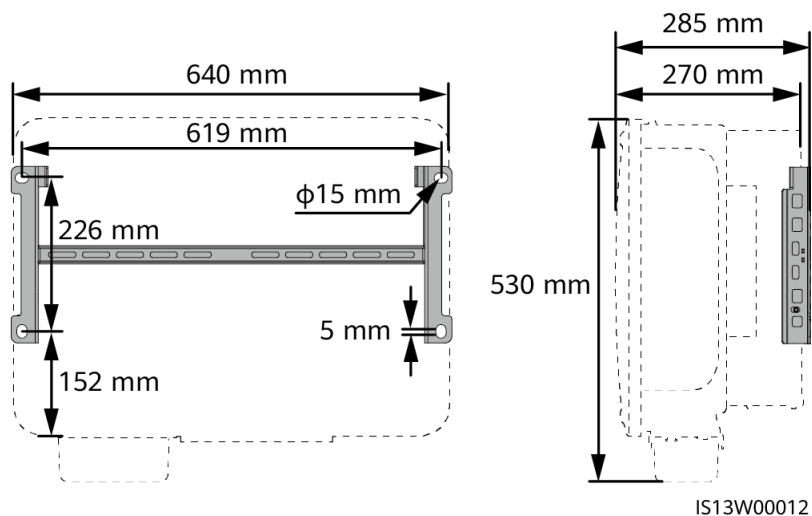
Abbildung 4-12 Abmessungen der Montagehalterung
