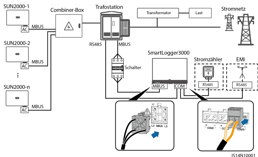
Abbildung 5-22 MBUS-Kommunikation (Großanlagen-Szenario)
