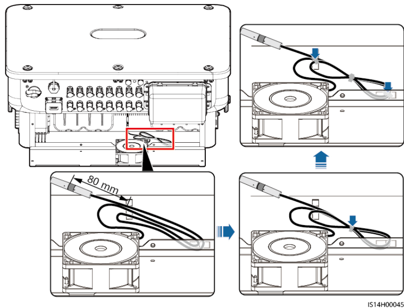
Abbildung 8-5 Binden der Kabel
