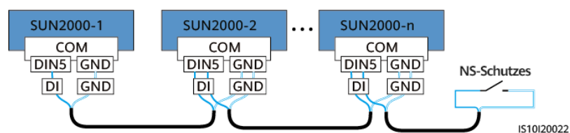
Abbildung I-1 Anschließen von kaskadierten Wechselrichtern an den NS-Schutzschalter
