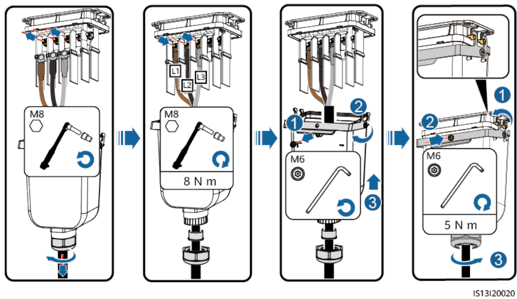
Abbildung 5-10 Dreiadriges Kabel (L1, L2 und L3)
