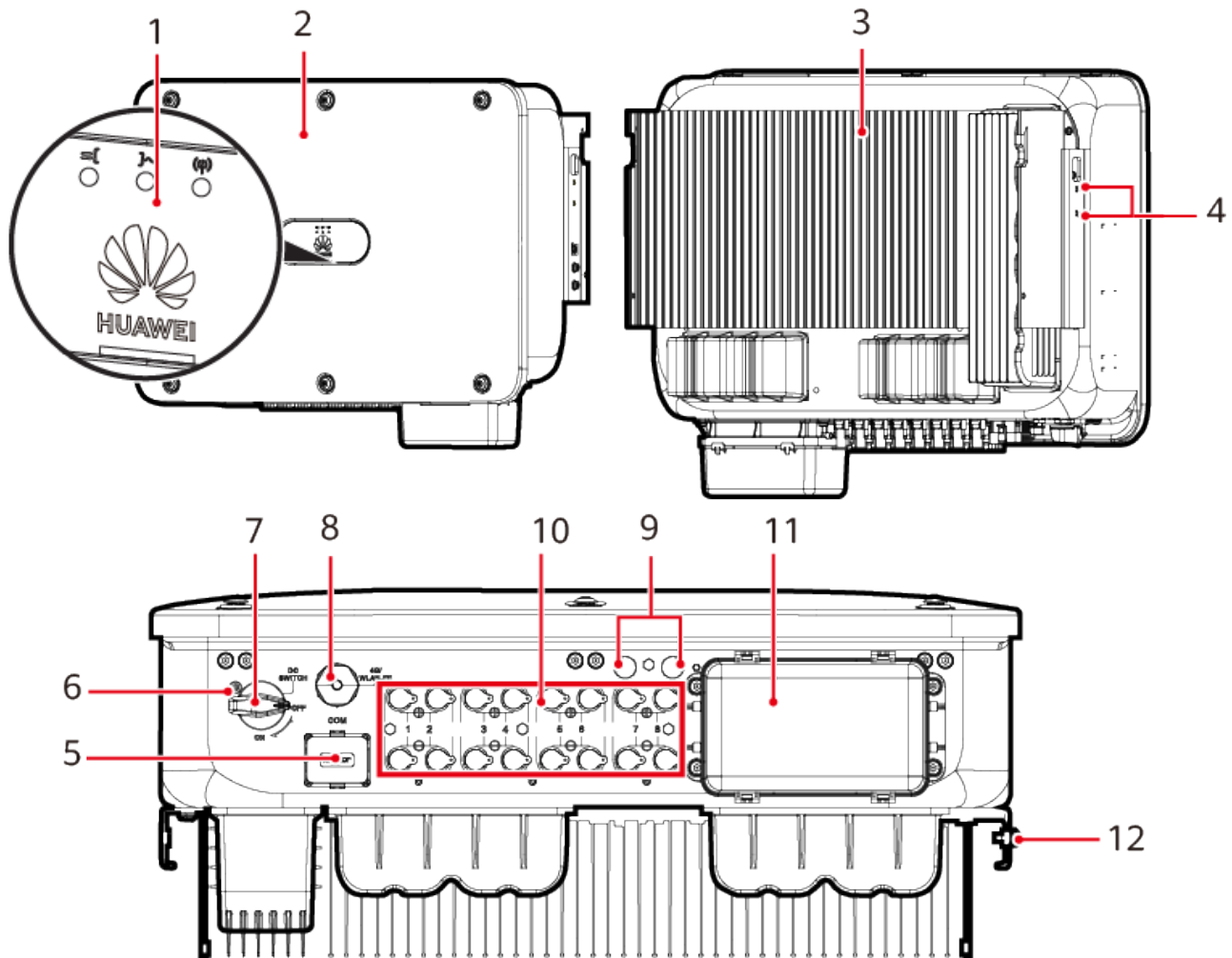
Abbildung 2-4 Erscheinungsbild
