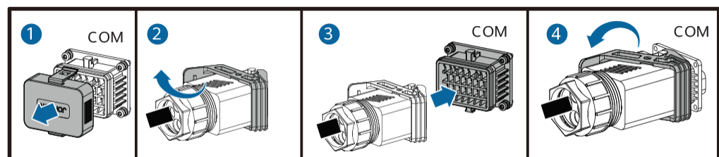
Abbildung 5-32 Sichern des Signalkabelsteckers
