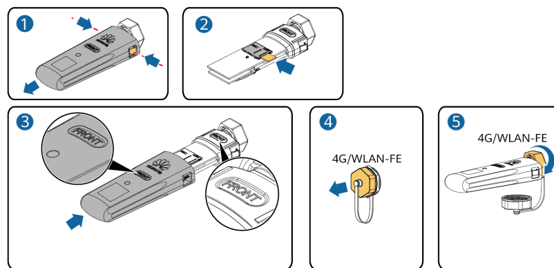
Abbildung 5-15 Installation des 4G Smart Dongle (SDongleA-03)
