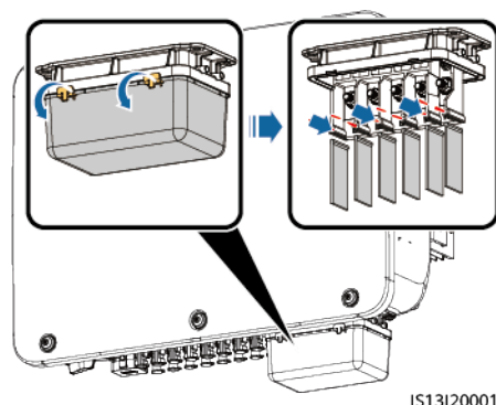
Abbildung 5-5 Entfernen der AC-Klemmenbox
