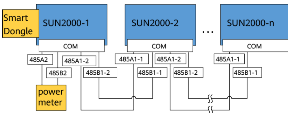
Abbildung 5-21 Smart Dongle-Netzwerkaufbau
