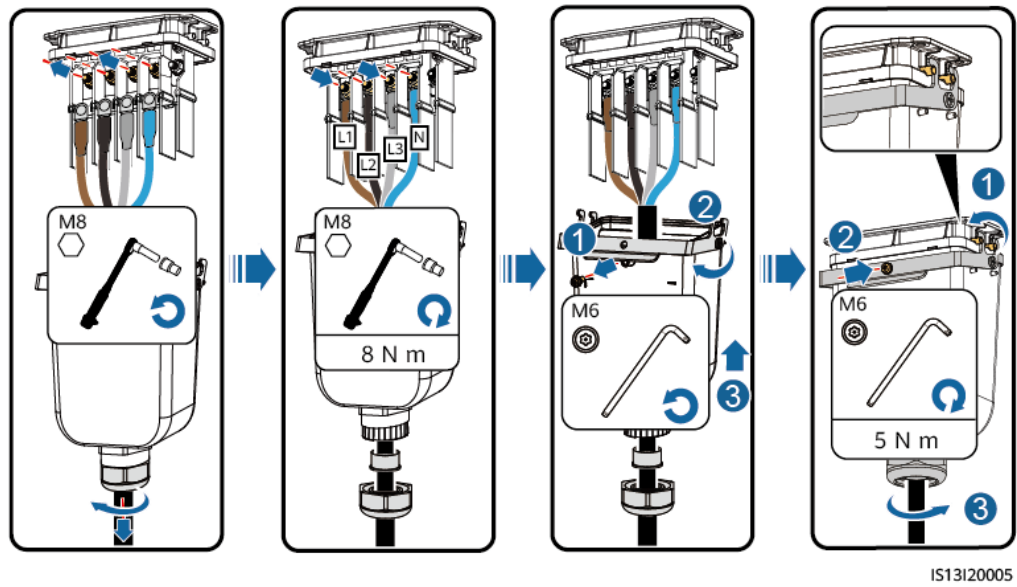
Abbildung 5-9 Vieradriges Kabel (L1, L2, L3 und N)
