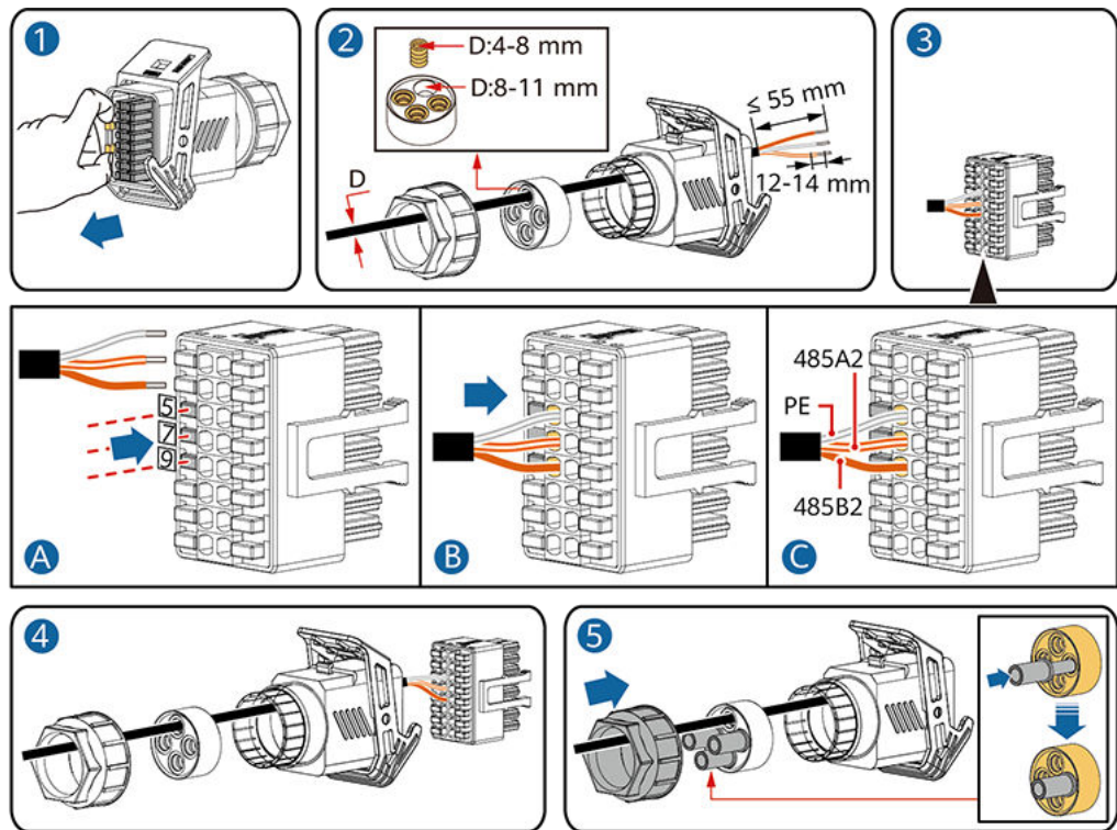
Abbildung 5-27 Installieren des Kabels
