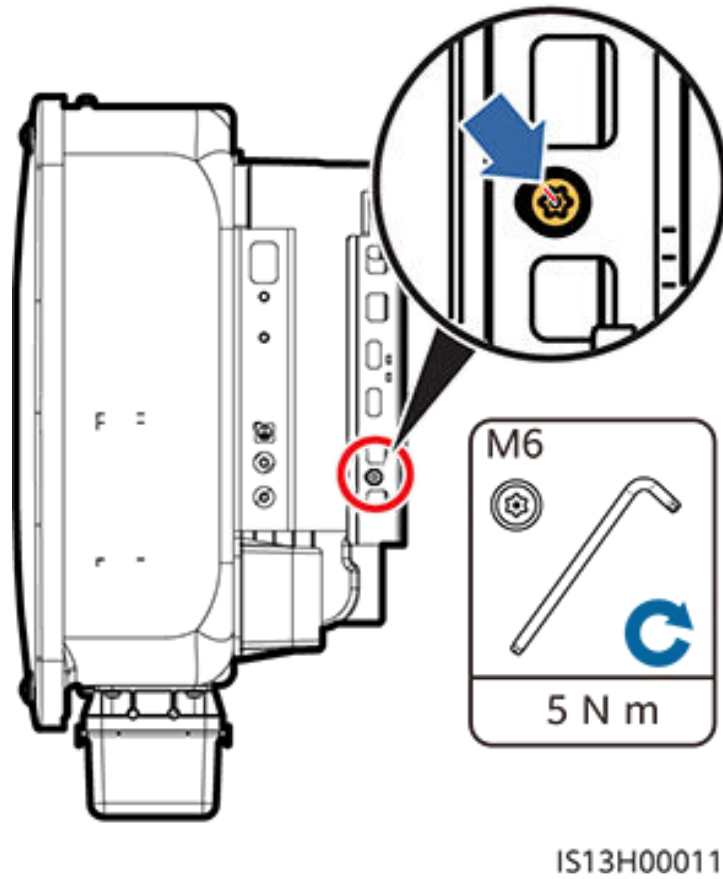
Abbildung 4-16 Festziehen der Schrauben
