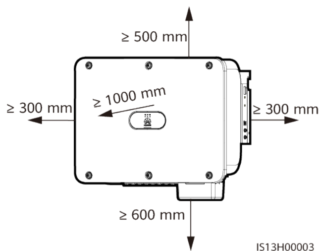
Abbildung 4-2 Abstände
