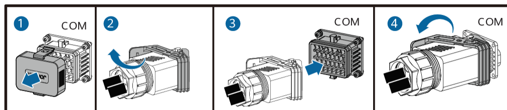
Abbildung 5-26 Sichern des Signalkabelsteckers
