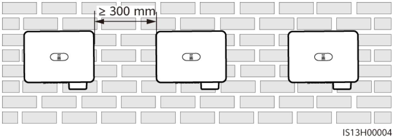
Abbildung 4-3 Horizontaler Montagemodus (empfohlen)
