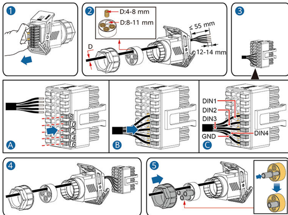
Abbildung 5-29 Anschließen des Kabels
