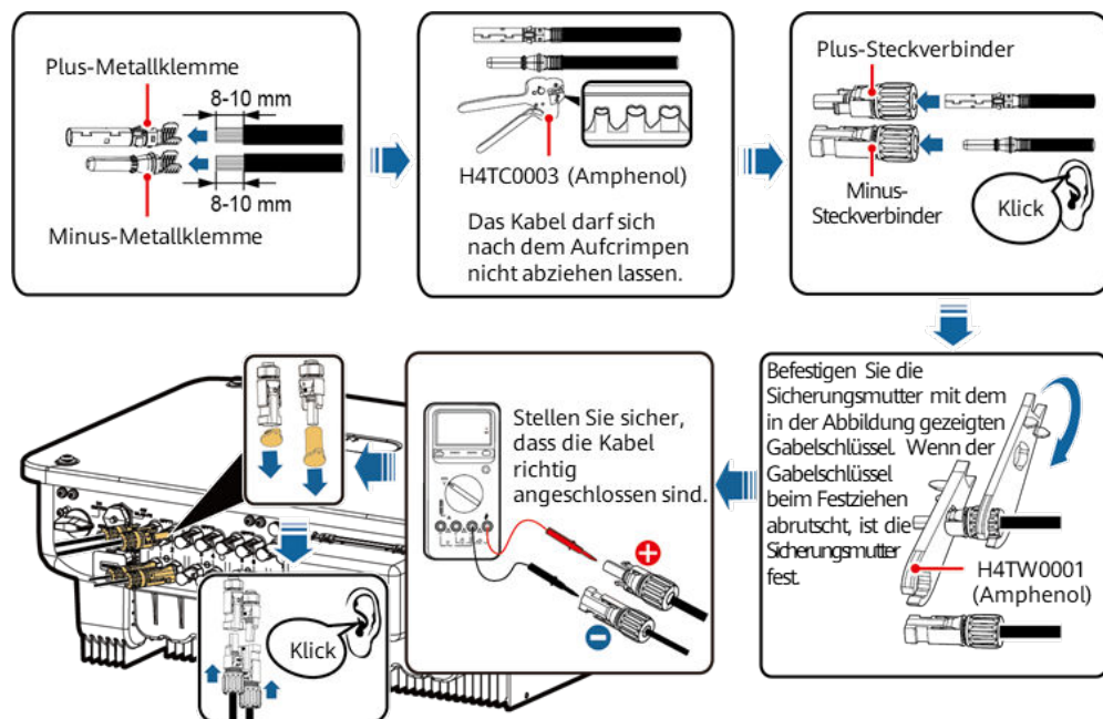
Abbildung 5-13 Anschließen der DC-Stromkabel
