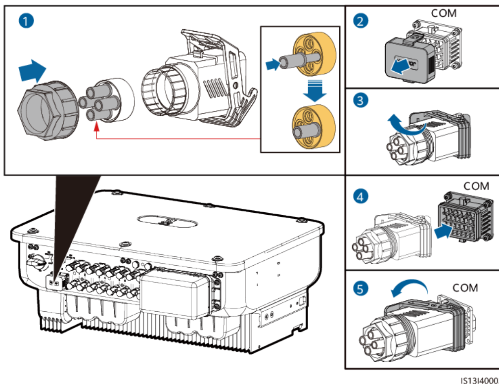
Abbildung 5-20 Anschließen des Signalkabelsteckers
