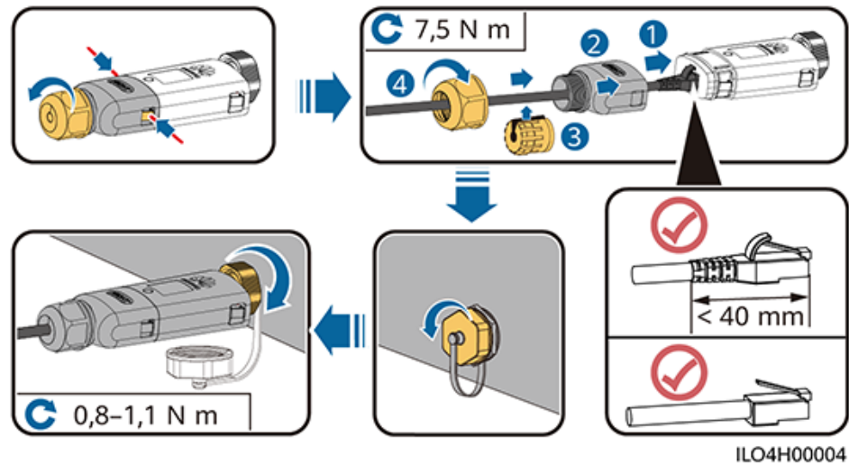
Abbildung 5-18 Anschließen des WLAN-FE Smart Dongle (FE-Kommunikation)
