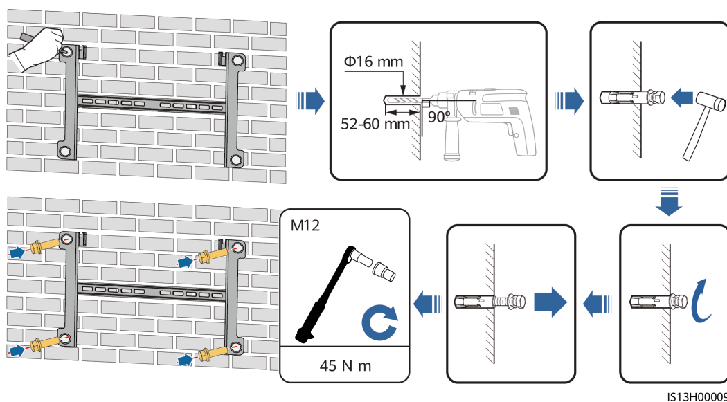
Abbildung 4-13 Einsetzen einer Dehnschraube
