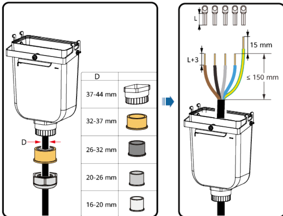
Abbildung 5-6 Abisolieren eines AC-Stromkabels (verwenden Sie beispielsweise ein fünfadriges Kabel)
