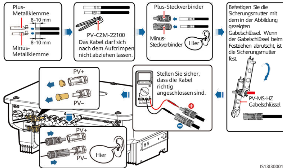
Abbildung 5-14 Anschließen der DC-Stromkabel
