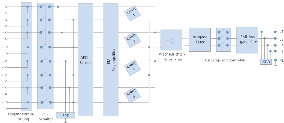
Abbildung 2-5 Schematisches Diagramm
