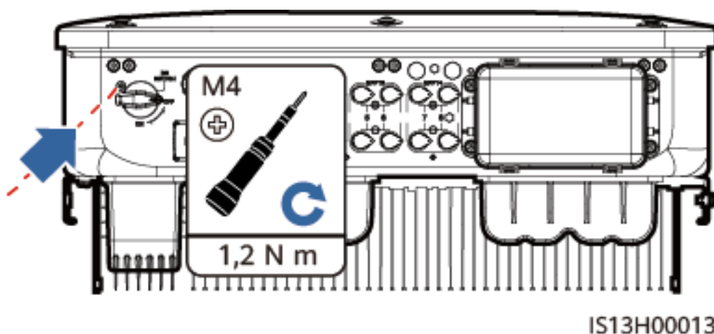
Abbildung 4-14 Montage der Sicherungsschraube des DC-Schalters
