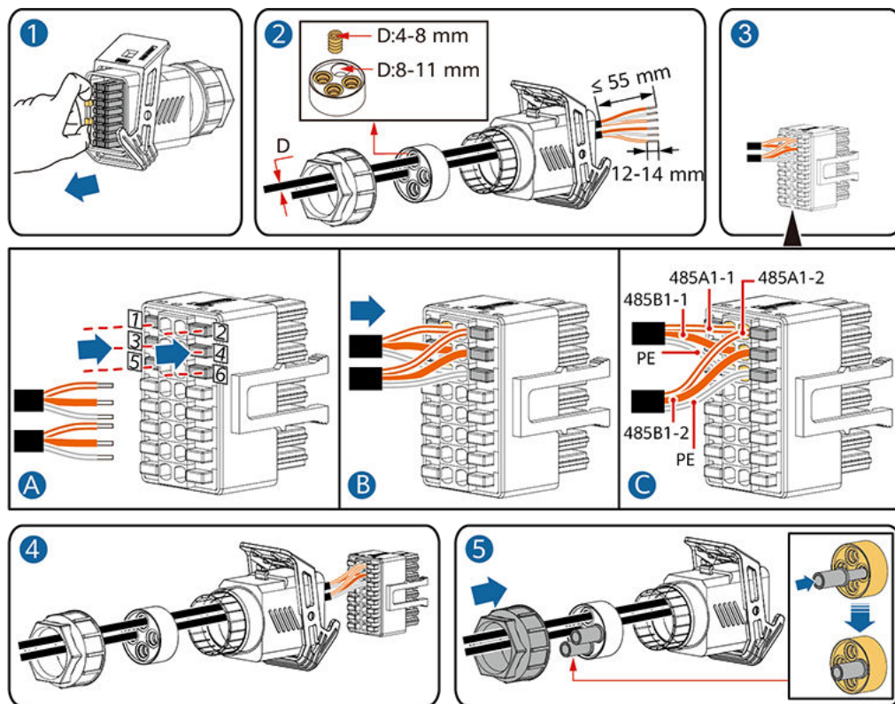
Abbildung 5-25 Anschließen des Kabels
