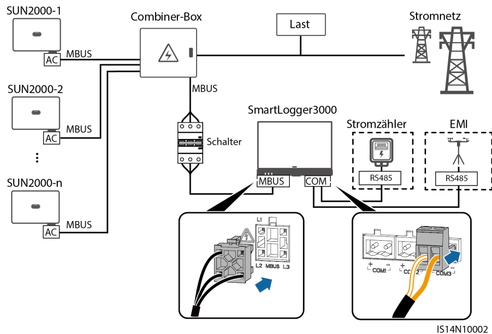
Abbildung 5-24 MBUS-Kommunikation (C&I-Szenario in China)
