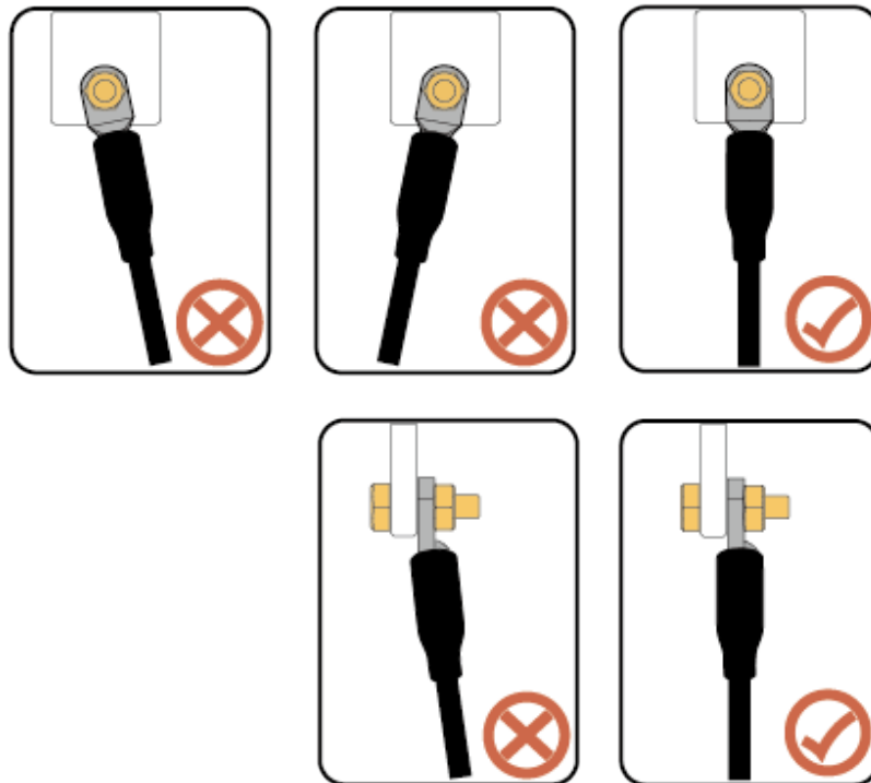
Abbildung 5-11 Verdrahtungsanforderungen
