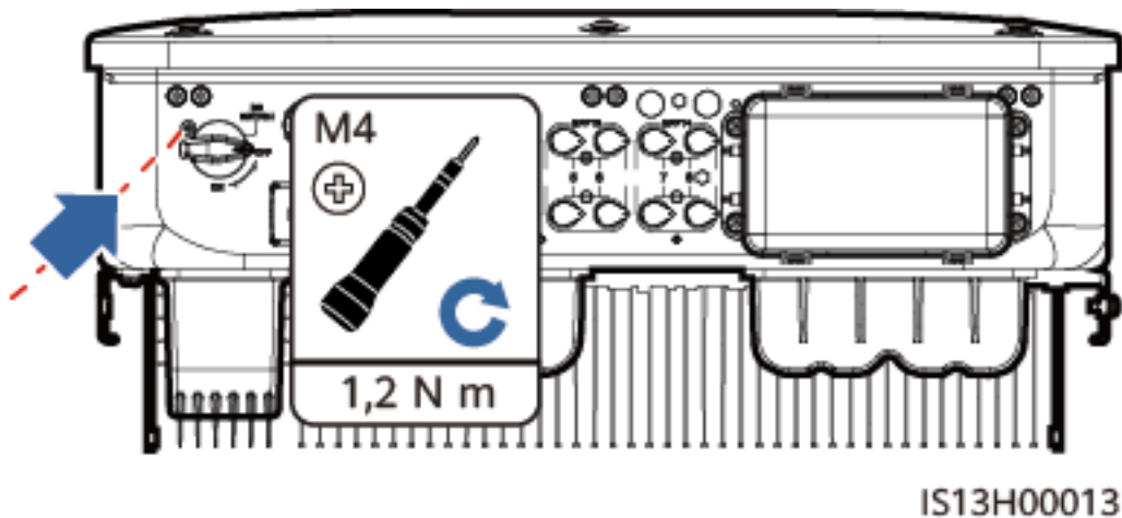
Abbildung 8-1 Montage der Sicherungsschraube des DC-Schalters
