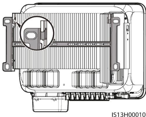
Abbildung 4-15 Montage des Wechselrichters
