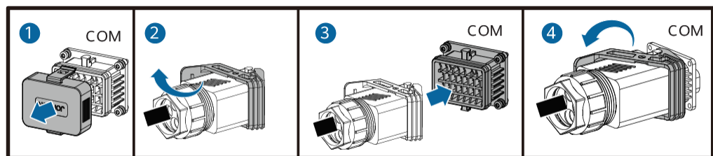
Abbildung 5-28 Sichern des Signalkabelsteckers
