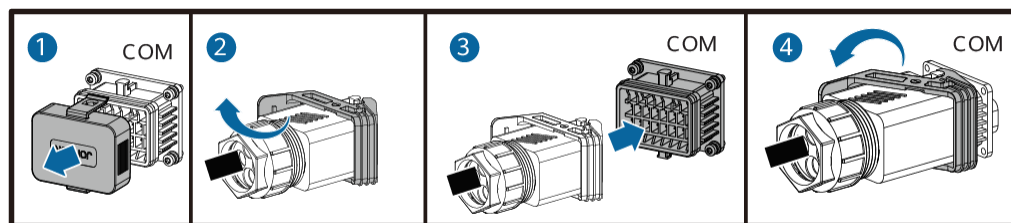
Abbildung 5-30 Sichern des Signalkabelsteckers
