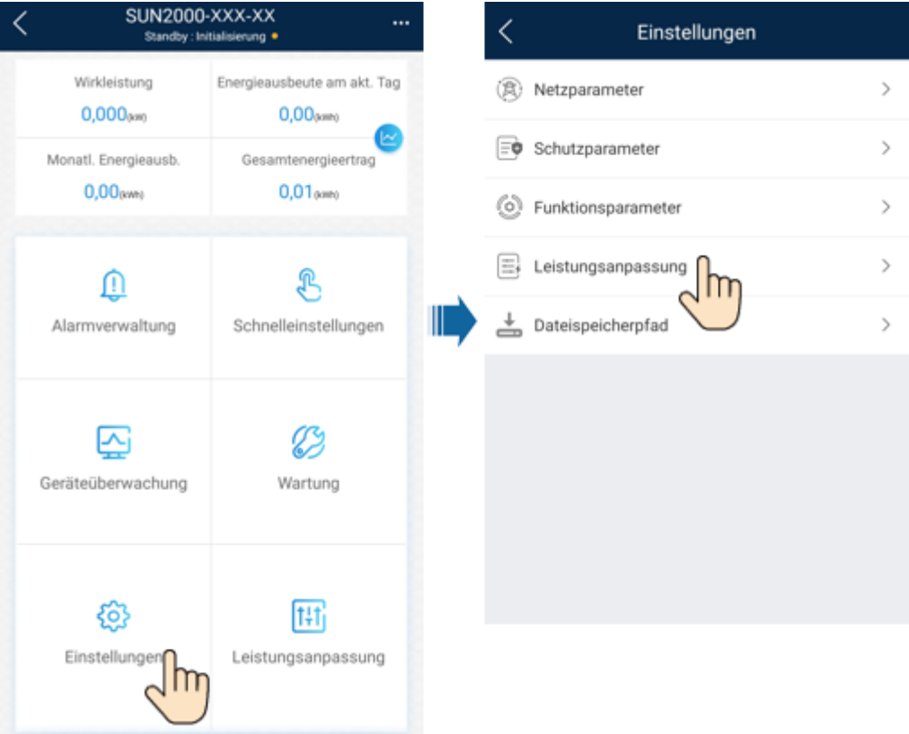
Abbildung 7-7 Scheinleistungssteuerung
