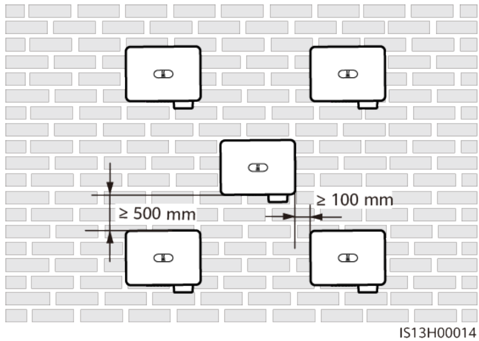
Abbildung 4-5 Dreischichtiger Dreiecksmontagemodus (nicht empfohlen)
