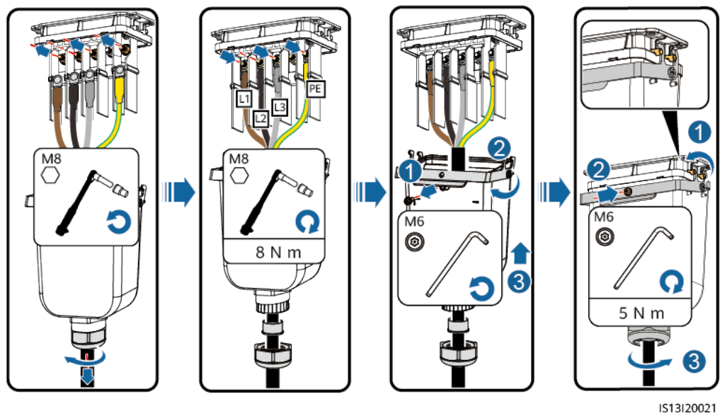
Abbildung 5-8 Vieradriges Kabel (L1, L2, L3 und PE)
