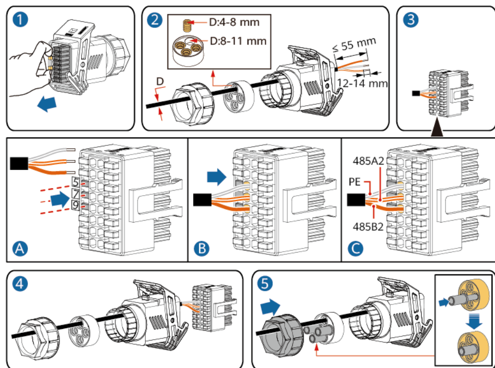
Abbildung 5-30 Kabelmontage
