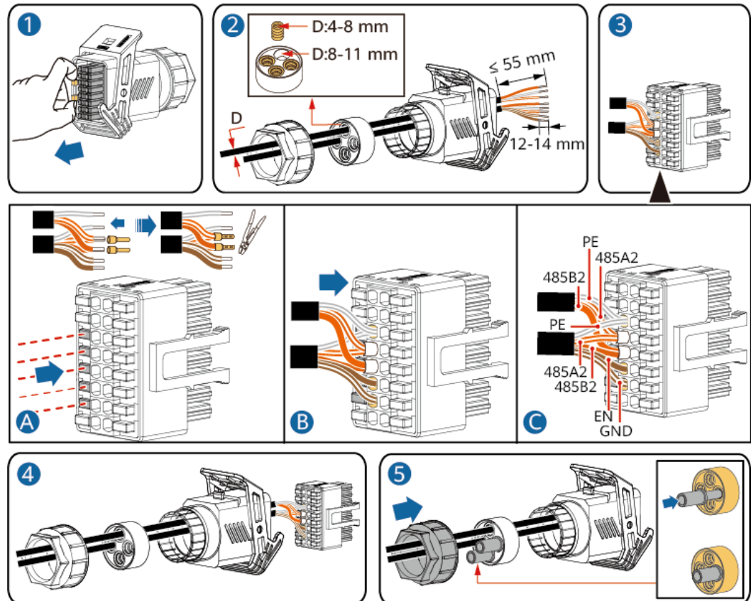
Abbildung 5-32 Kabelmontage
