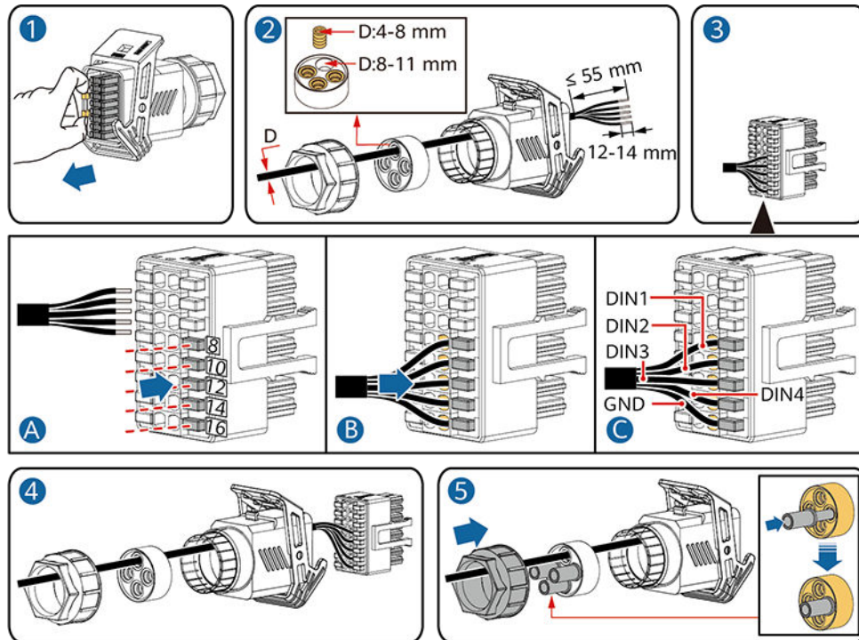
Abbildung 5-42 Kabelmontage
