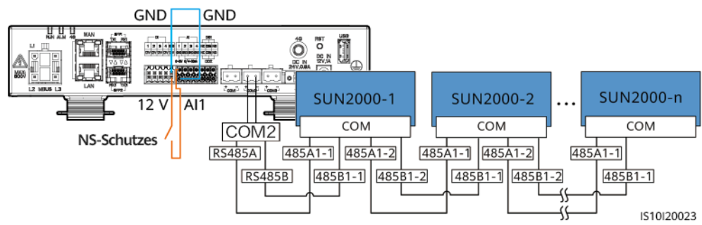
Abbildung 5-49 Anschließen des SmartLoggers an den NS-Schutzschalter
