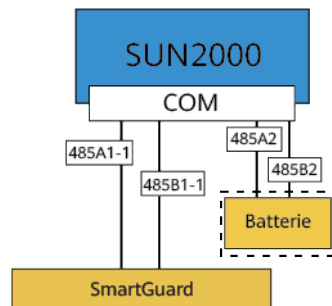
Abbildung 5-24 SmartGuard-Vernetzung (die Komponente im gestrichelten Kasten ist optional)
