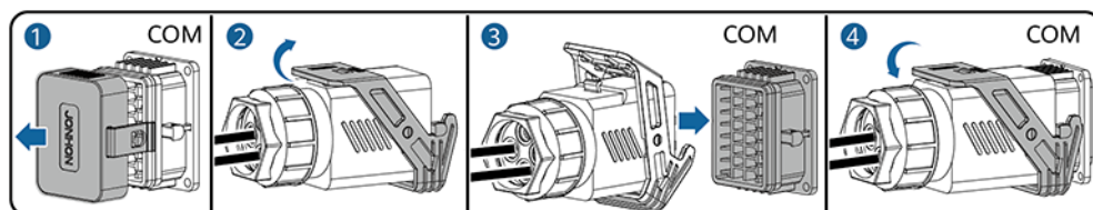
Abbildung 5-26 Sichern des Signalkabelanschlusses
