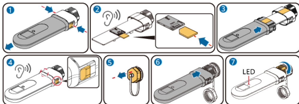
Abbildung 5-18 Installieren von 4G Smart Dongle (SDongleB-06)
