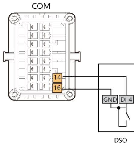
Abbildung 7-10 Kabelverbindungen
