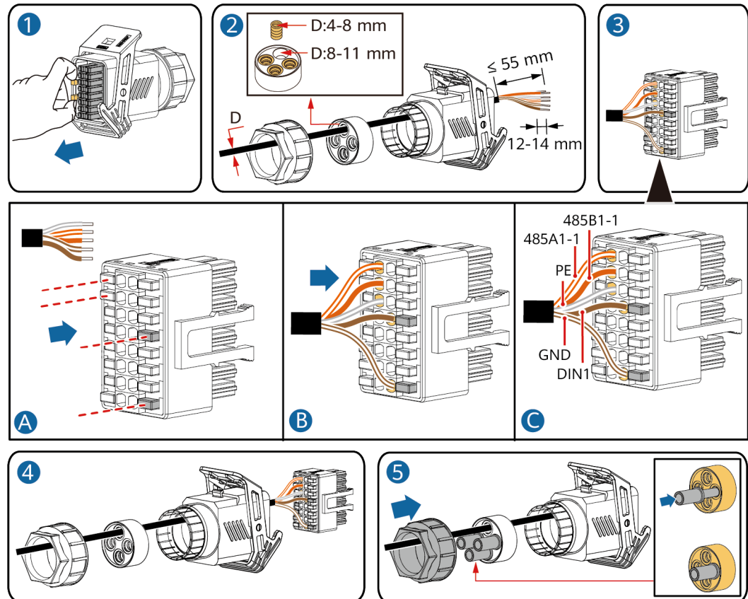
Abbildung 5-38 Kabelmontage
