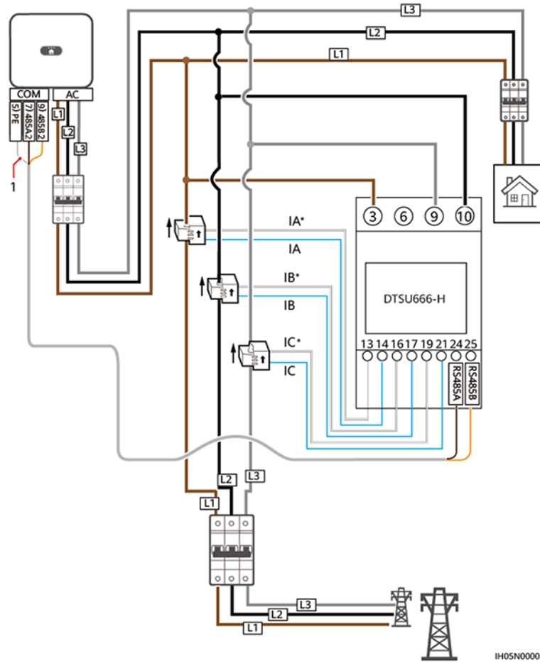
Abbildung 5-27 Dreiphasige, dreidrigige Kabelverbindung mit DTSU666-H (Smart Dongle- Vernetzung)
