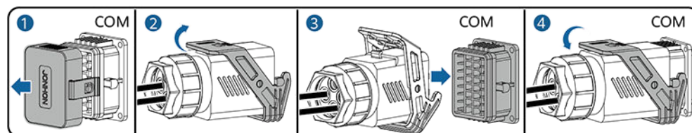
Abbildung 5-28 Sichern des Signalkabelanschlusses
