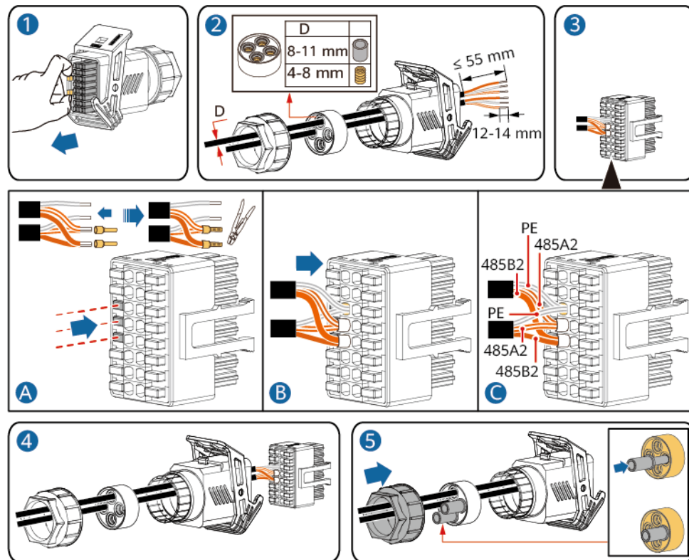
Abbildung 5-27 Kabelmontage
