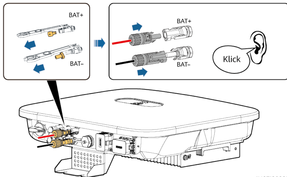
Abbildung 5-15 Anschließen der Akkukabel
