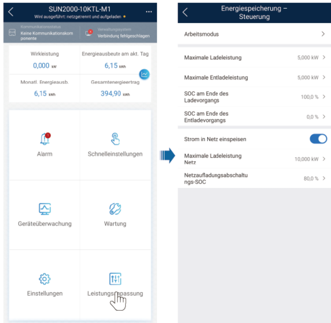
Abbildung 7-13 Einstellen der Akkusteuerungsparameter
