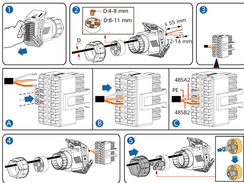
Abbildung 5-25 Kabelmontage
