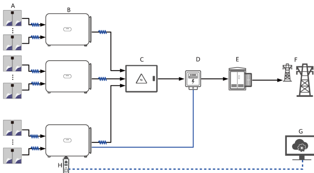
Abbildung 2-5 MBUS-Vernetzungsanwendung (Dongle)
