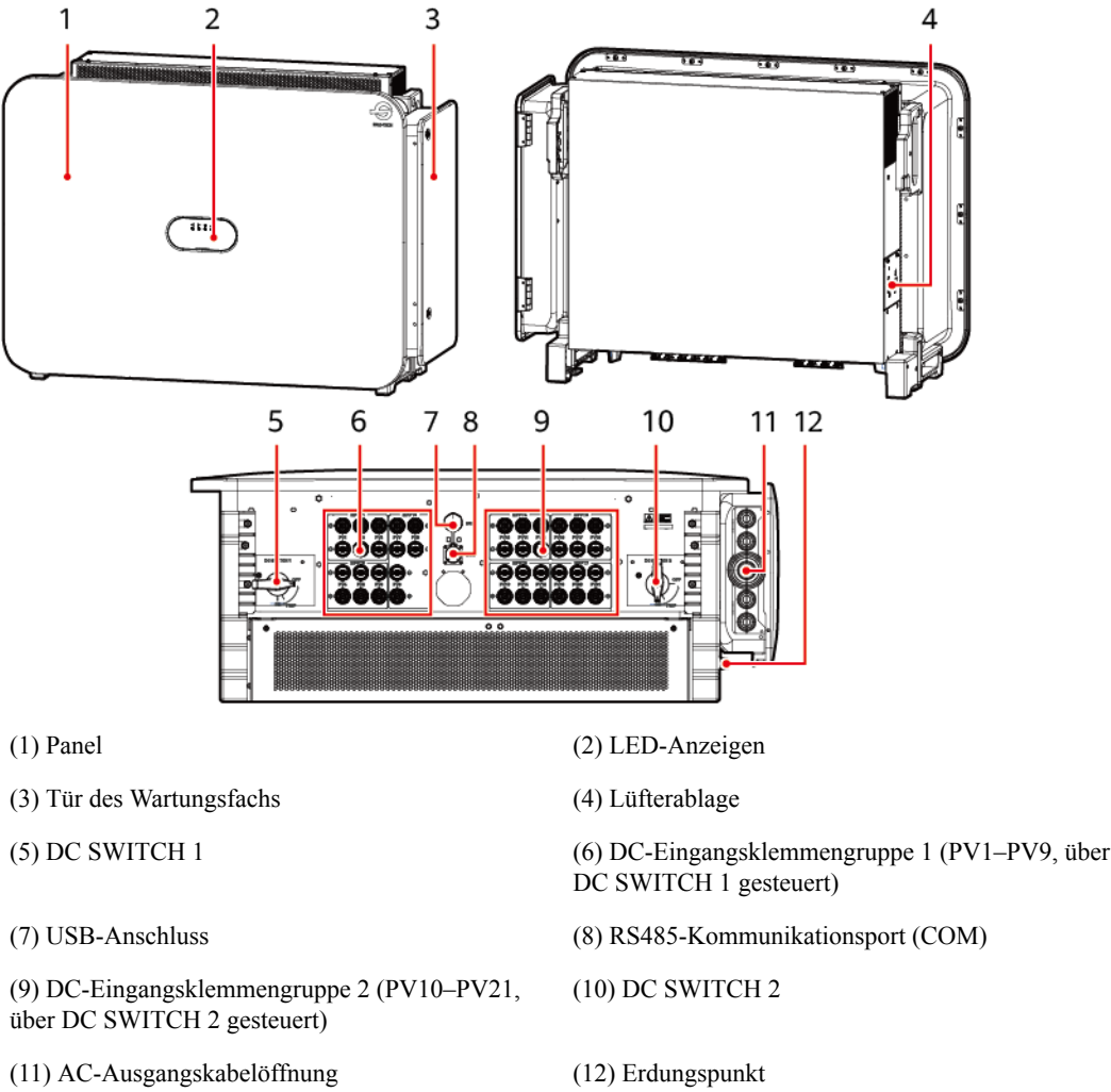
Abbildung 2-7 Erscheinungsbild
