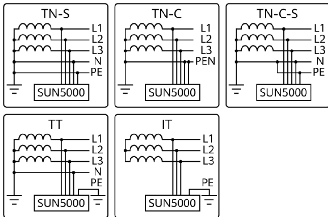
Abbildung 2-6 Erdungssysteme
