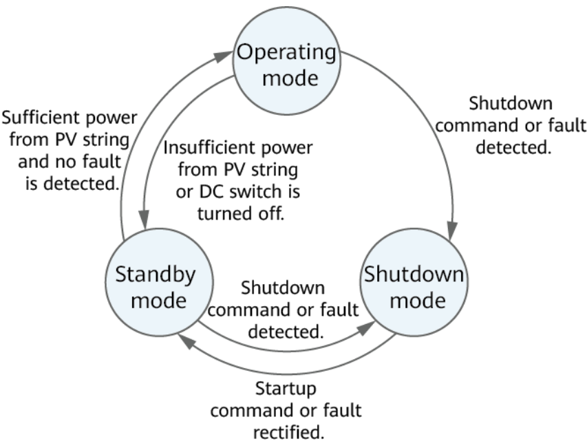
Abbildung 2-10 Arbeitsmodi
