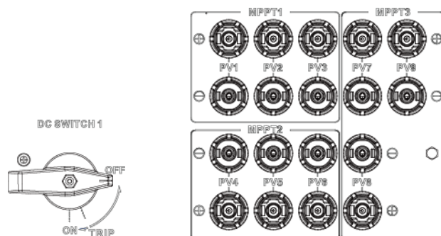
Abbildung 5-11 Durch DC SWITCH 1 gesteuerte DC-Klemmen
