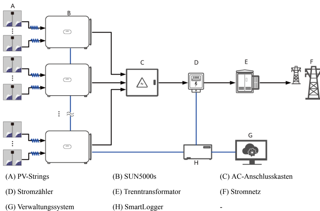
Abbildung 2-2 RS485-Vernetzungsanwendung (SmartLogger)
