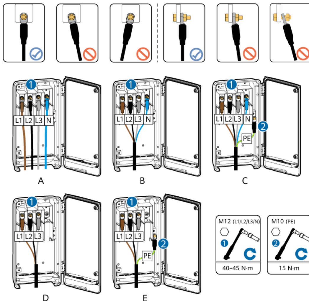
Abbildung 5-6 Kabelanschluss
