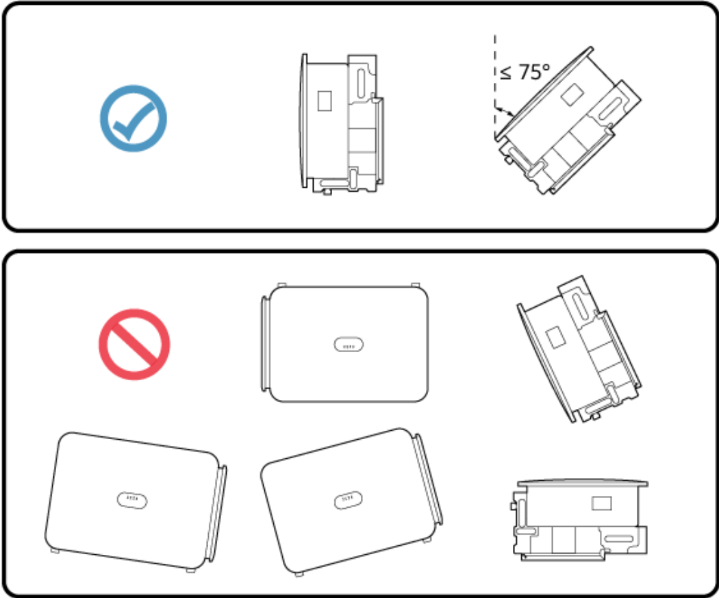
Abbildung 4-7 Installationswinkel
