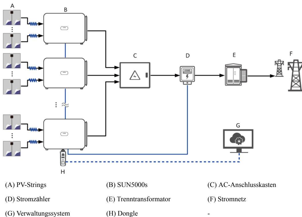
Abbildung 2-3 RS485-Vernetzungsanwendung (Dongle)
