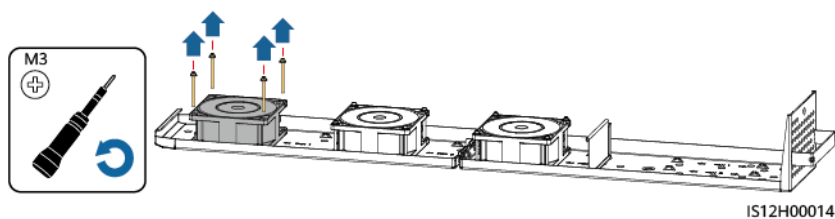
Abbildung 8-8 Entfernen eines Lüfters
