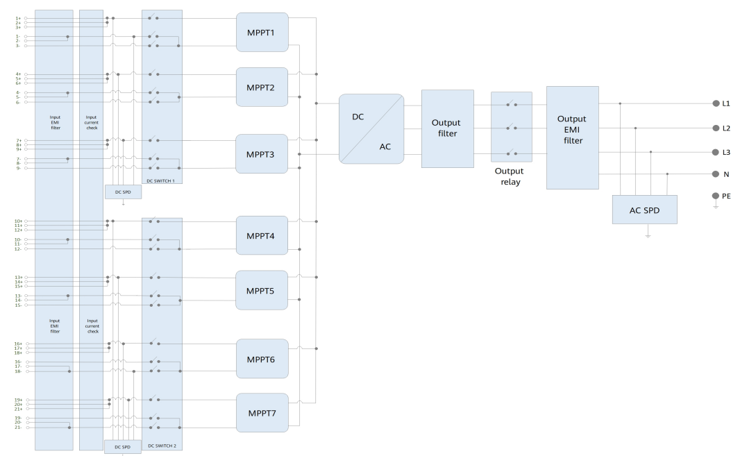
Abbildung 2-9 Stromlaufplan
