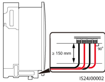
Abbildung 5-14 Anschließen der DC-Eingangsstromkabel (AVIC JONHON)
