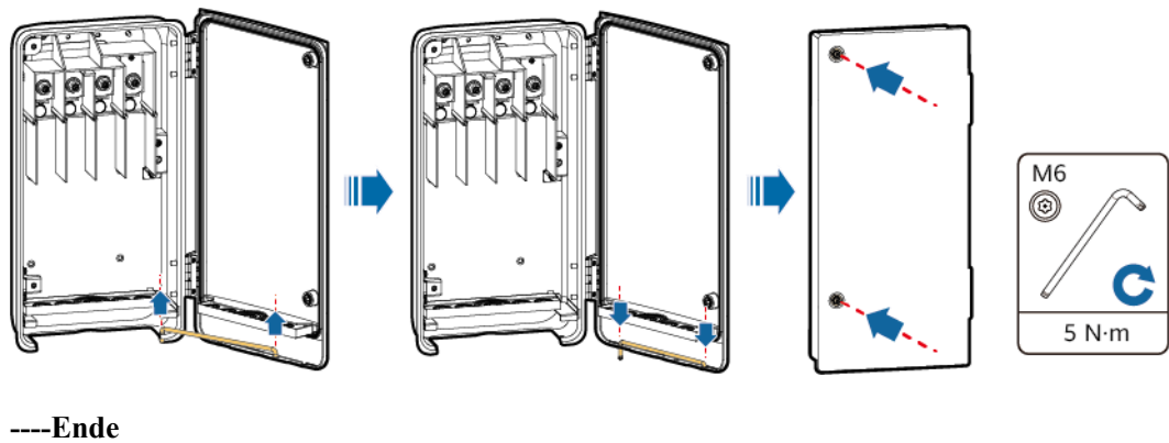
Abbildung 5-9 Schließen einer Tür
