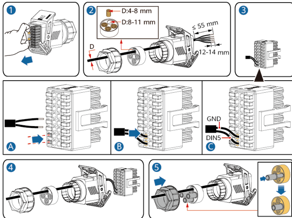
Abbildung 5-36 Kabelmontage
