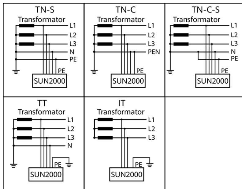
Abbildung 2-9 Unterstützte Stromnetze
