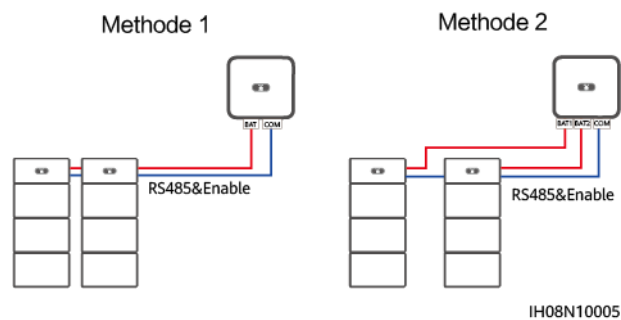
Abbildung 2-7 Anschluss des Wechselrichters an zwei Batterien
