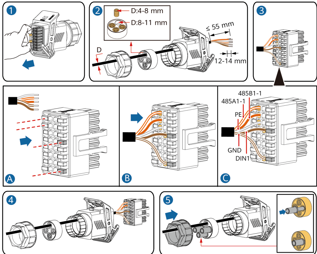
Abbildung 5-34 Kabelmontage
