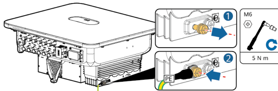
Abbildung 5-3 Anschließen des PE-Kabels
