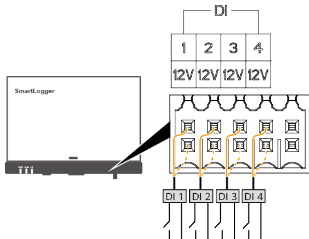
Abbildung 5-39 Kabelverbindungen (SmartLogger-Vernetzung)
