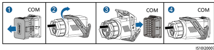
Abbildung 5-31 Sichern des Signalkabelsteckverbinders
