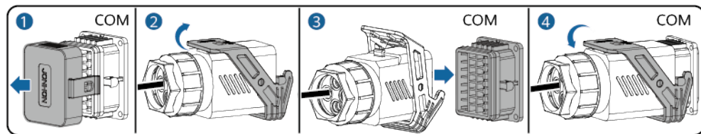
Abbildung 5-41 Sichern des Signalkabelsteckers
