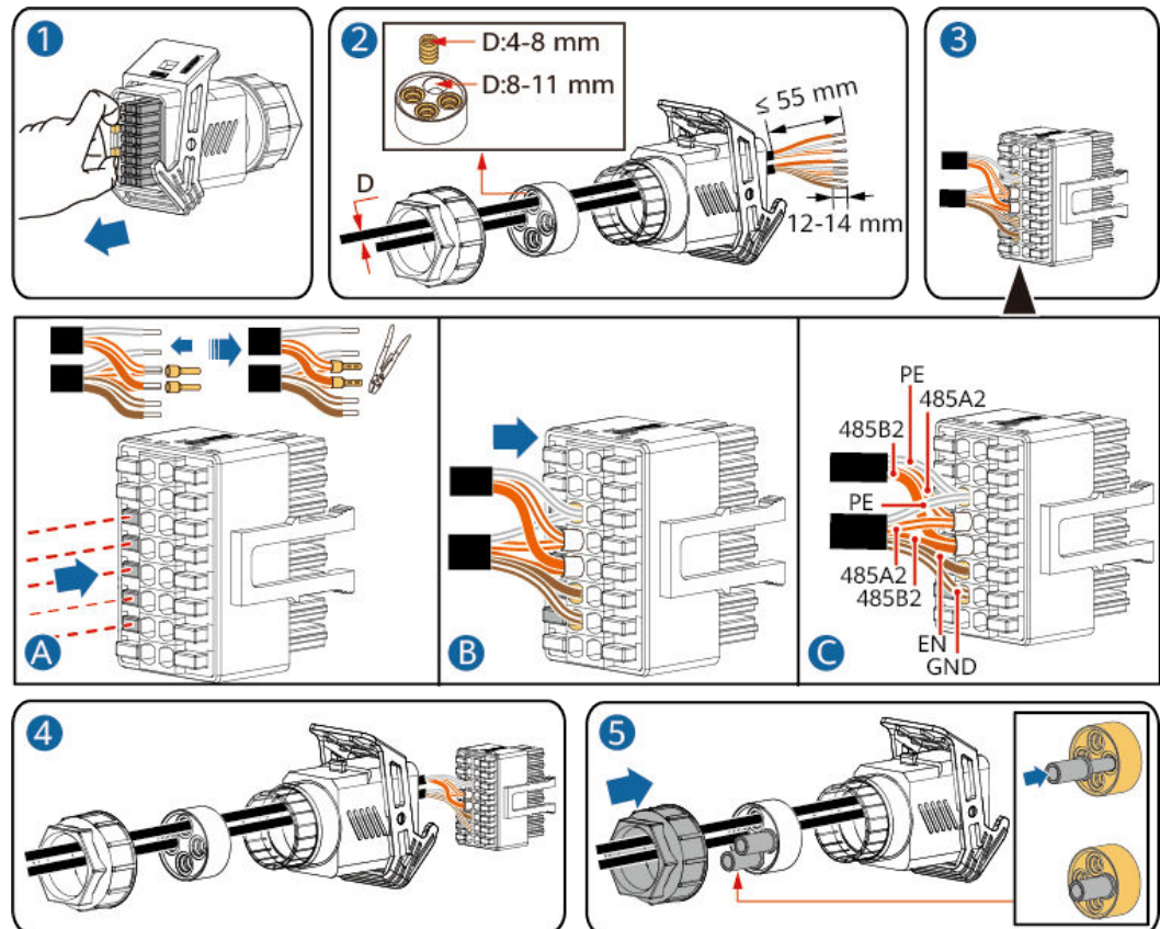
Abbildung 5-28 Installieren von Kabeln
