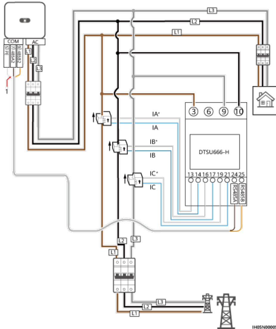
Abbildung 5-23 DTSU666-H dreiphasige dreiadrige Kabelverbindung (Smart Dongle-Vernetzung)
