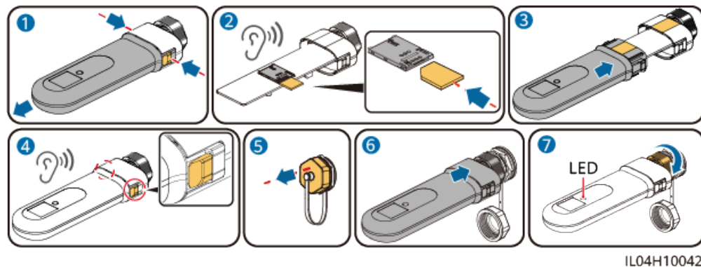
Abbildung 5-48 Installieren von 4G Smart Dongle (SDongleB-06)
