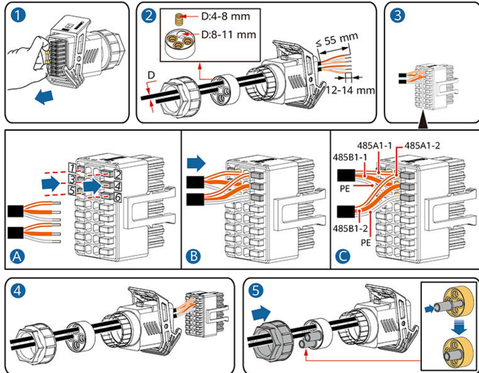
Abbildung 5-21 Kabelmontage
