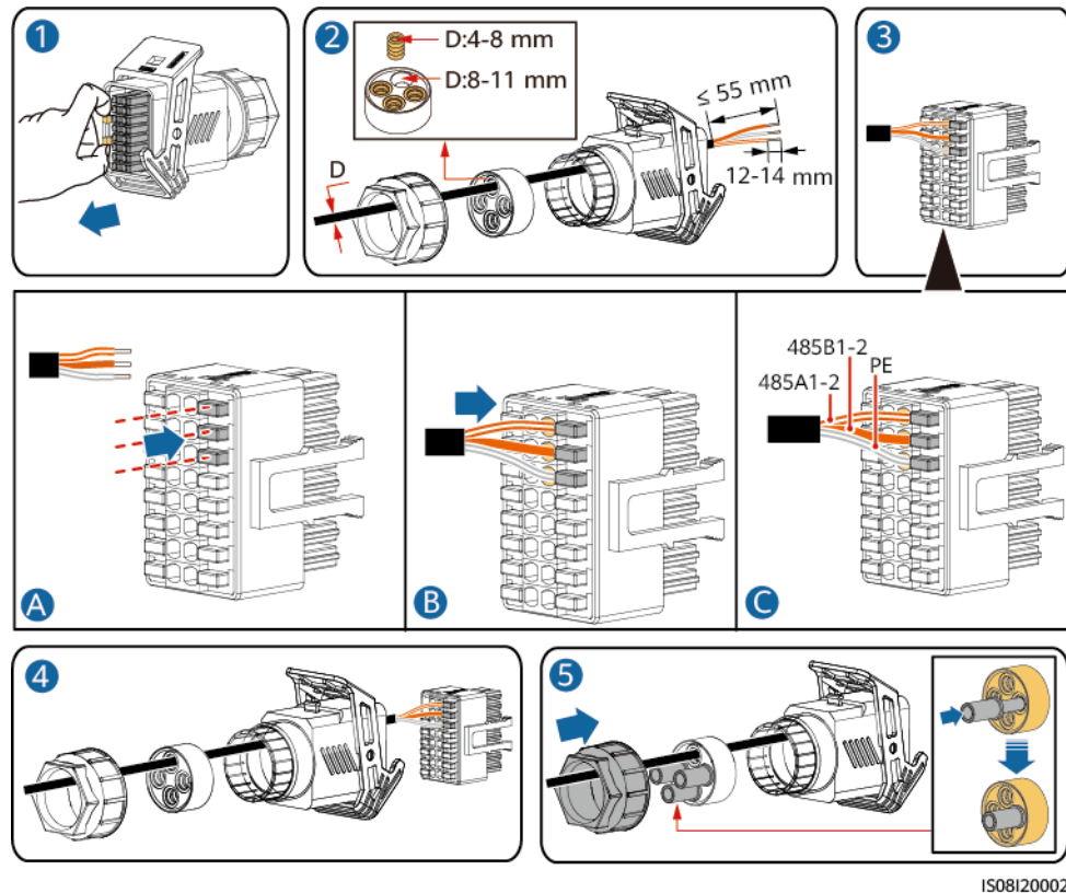
Abbildung 5-30 Kabelmontage
