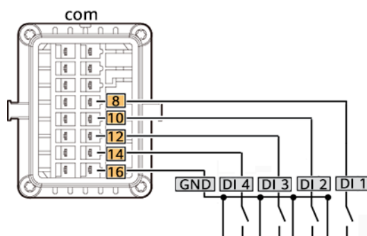
Abbildung 5-28 Kabelverbindung
