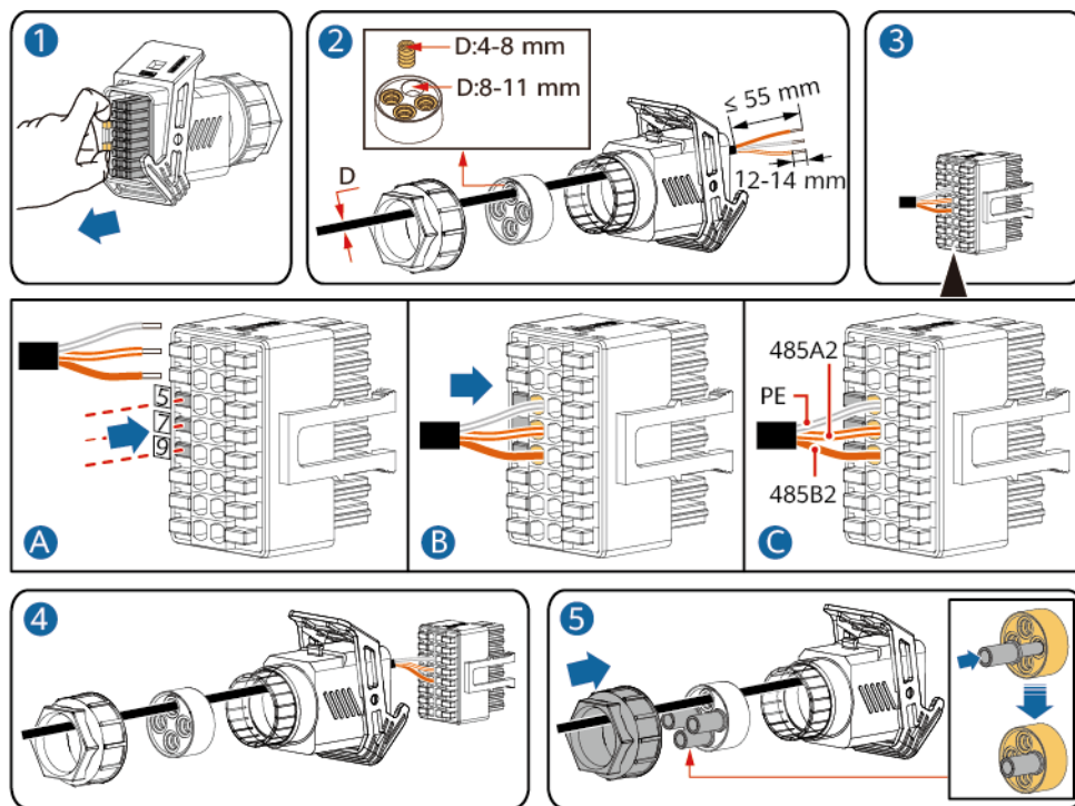
Abbildung 5-24 Kabelmontage
