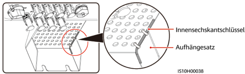
Abbildung 5-4 Innensechskantschlüssel
