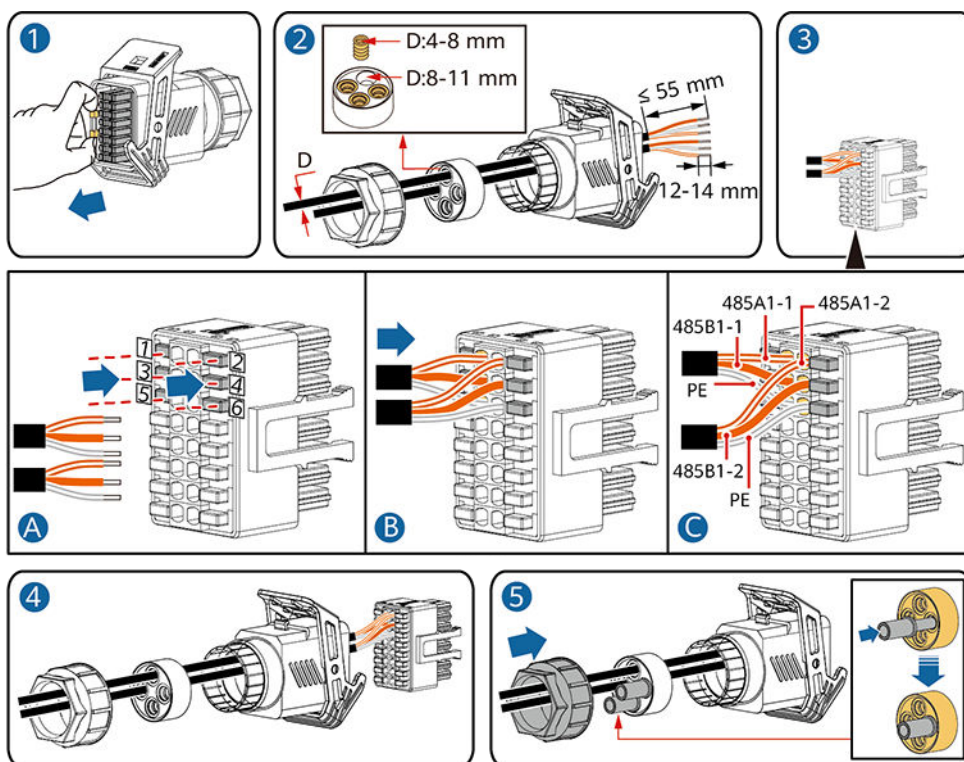
Abbildung 5-20 Kabelmontage
