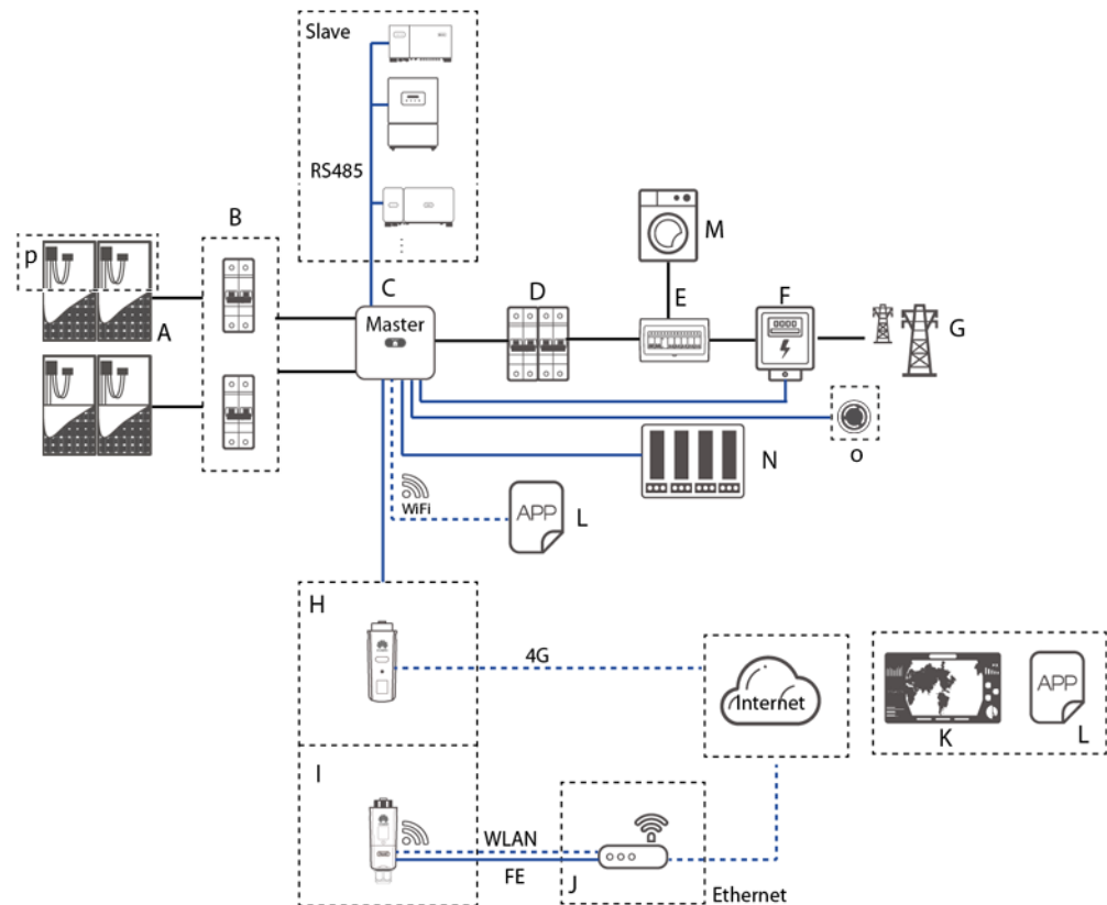
Abbildung 2-3 Netzerkanwendung – Szenario mit Kaskadierung von Wechselrichtern (optional in gestrichelten Kästchen)
