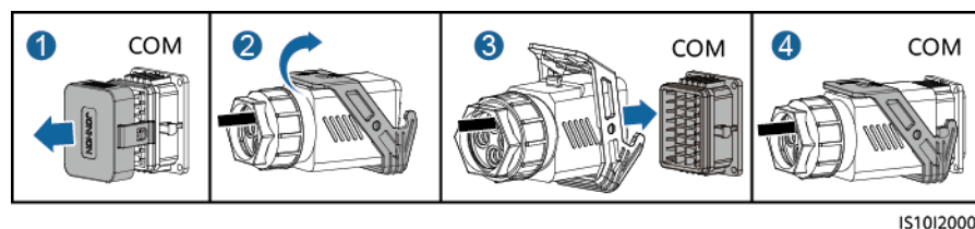
Abbildung 5-27 Sichern des Signalkabelanschlusses
