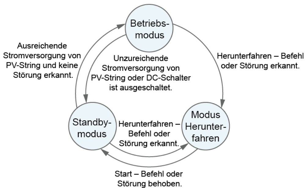
Abbildung 2-8 Arbeitsmodi
