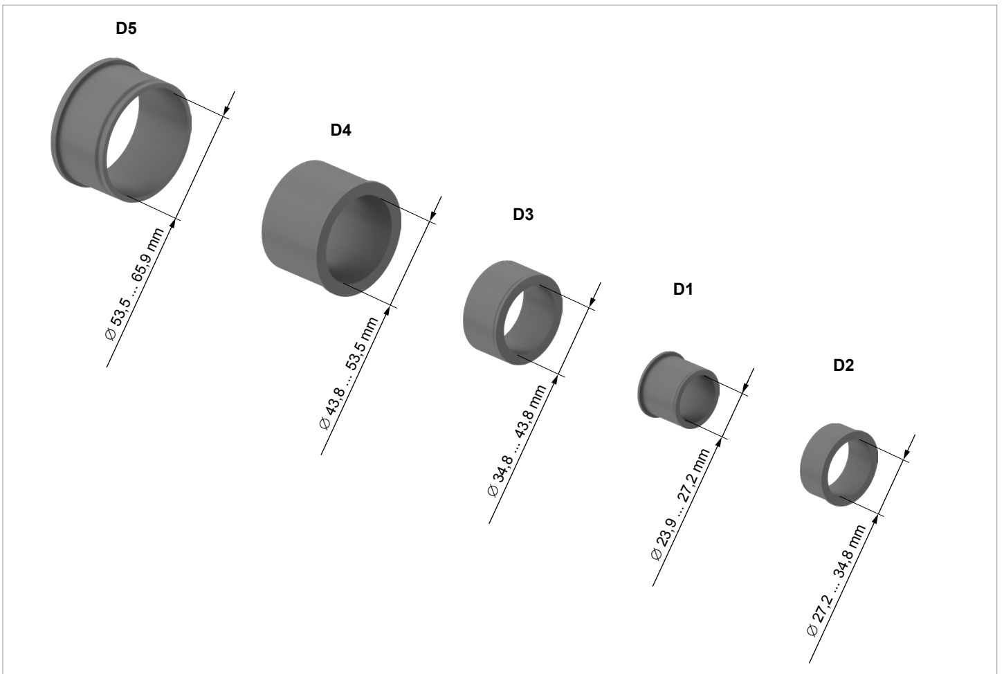
AC-Kabelverschraubung, Variante B: Abmessungen der Dichtungsringe
