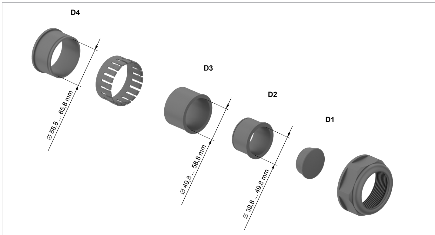
AC-Kabelverschraubung, Variante A: Übersicht der Teile und Abmessungen der Dichtungsringe
