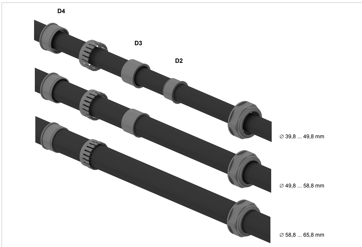
AC-Kabelverschraubung, Variante A: Zuordnung der Dichtungsringe zu den Kabeldurchmessern
