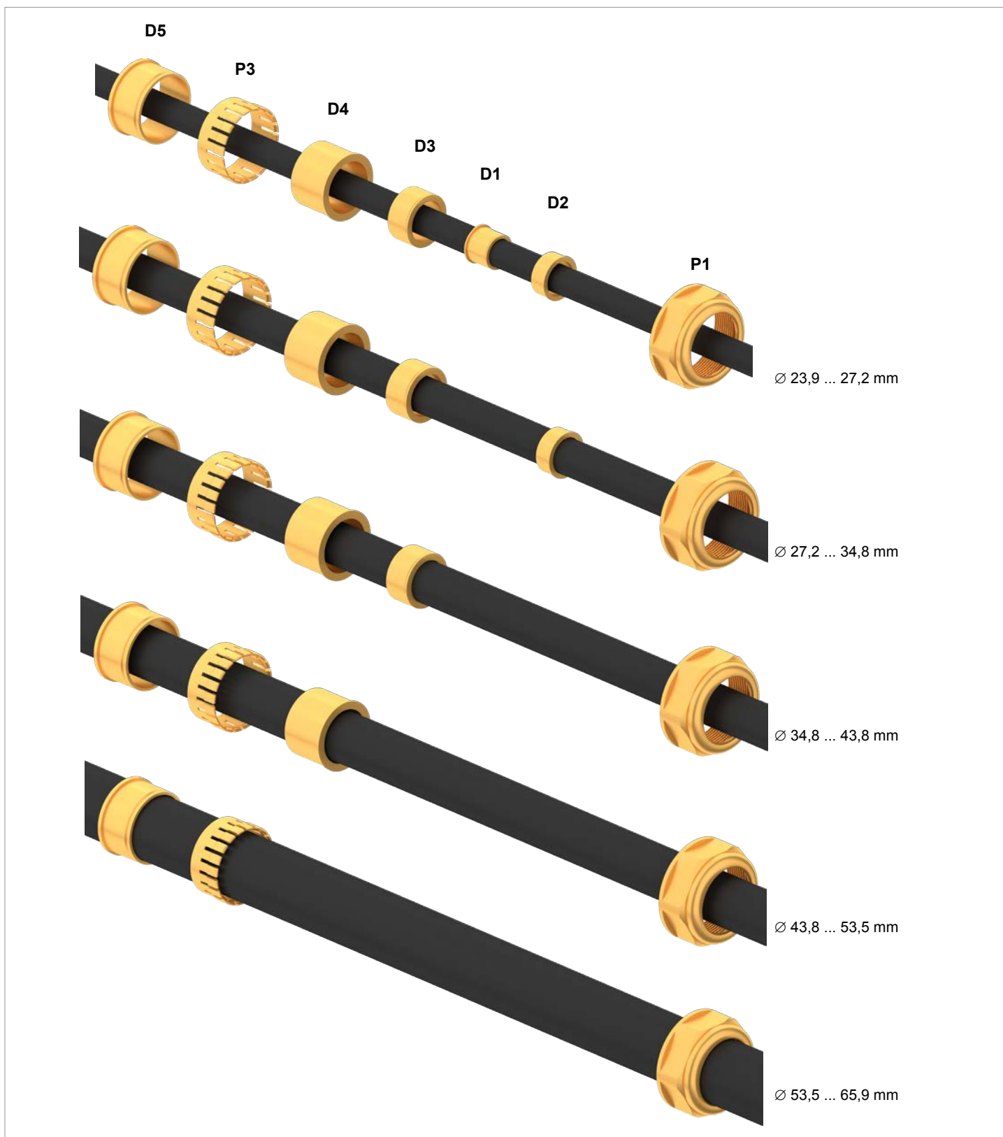
AC-Kabelverschraubung, Variante B: Zuordnung der Dichtungsringe zu den Kabeldurchmessern
