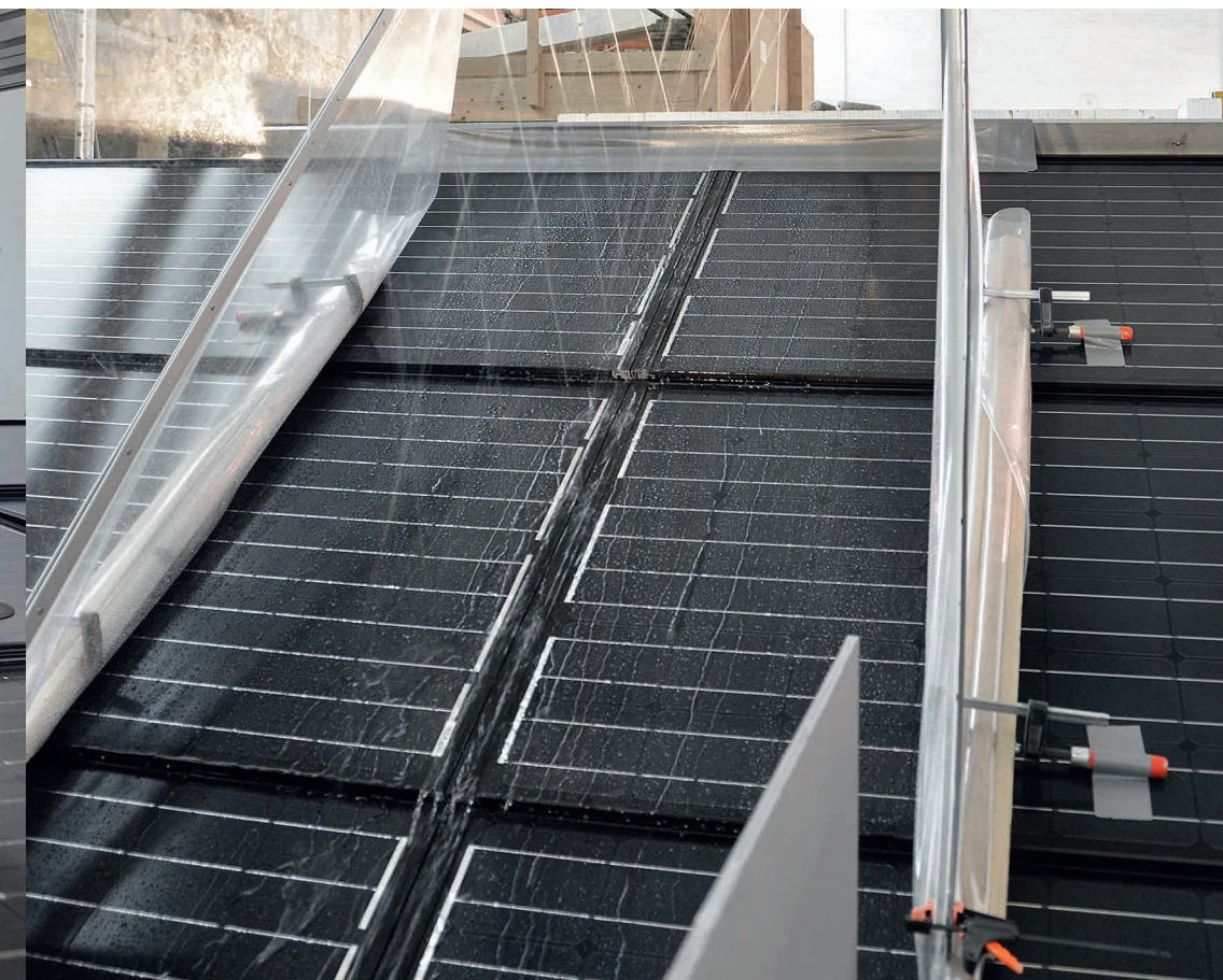
Test d'étanchéité effectué à l'Institut de contrôle et de recherche de Sursee
